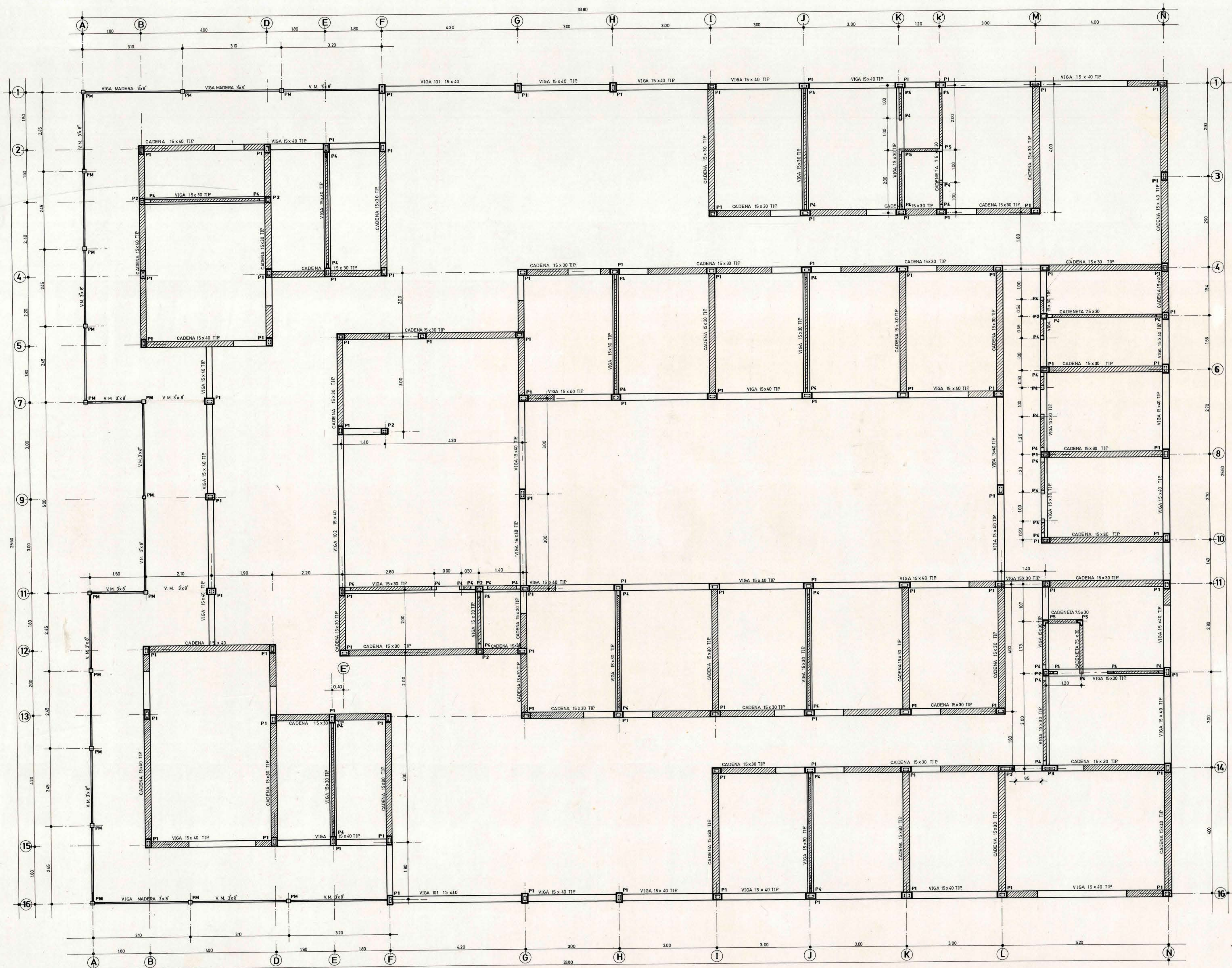
PLANTA DE ESTRUCTURAS ESCALA 1:50
