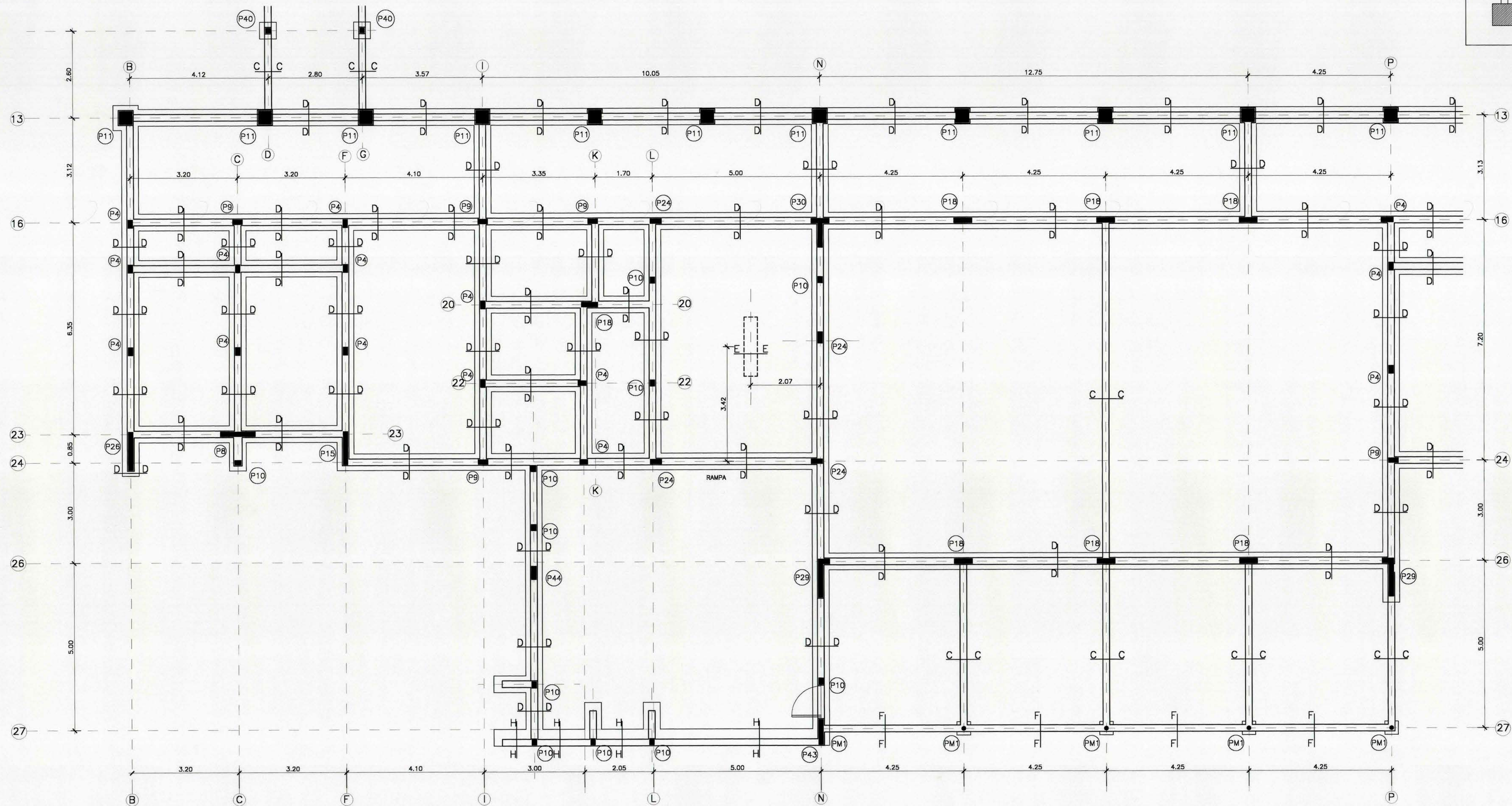
PLANTA DE FUNDACIONES MODULO C ESCALA 1 : 50
