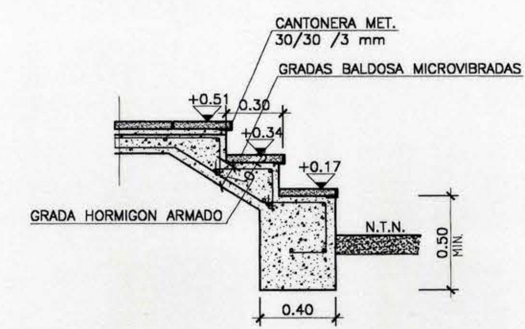
GRADA TIPICA ESCALA 1 : 20
