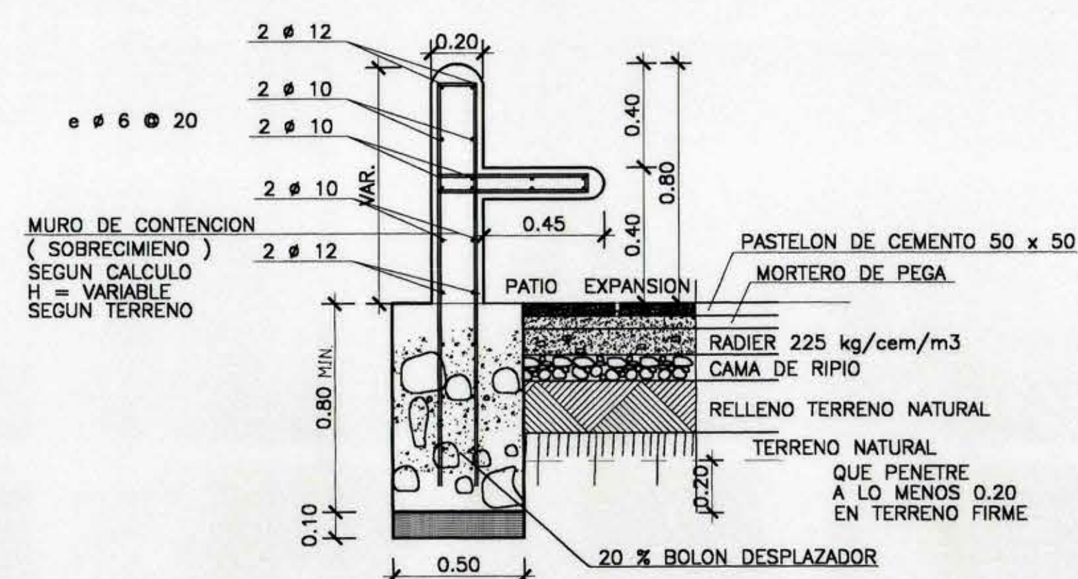
SECCION I-I PATIO DE EXPANSION ESCALA 1 : 20
