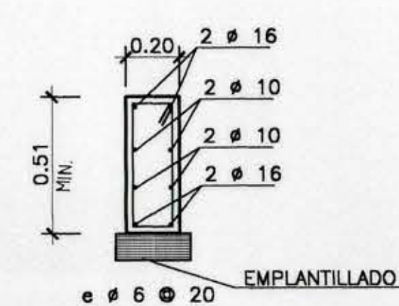
VIGA FUNDACION SECCION G-G ESCALA 1 : 20
