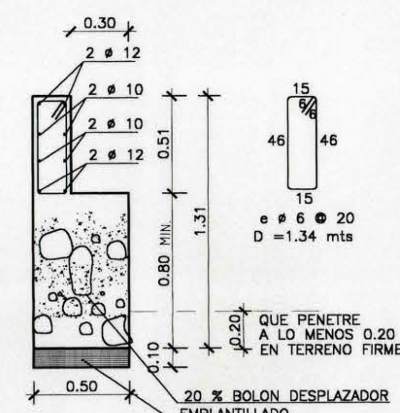
SECCION H-H ESCALA 1 : 20
