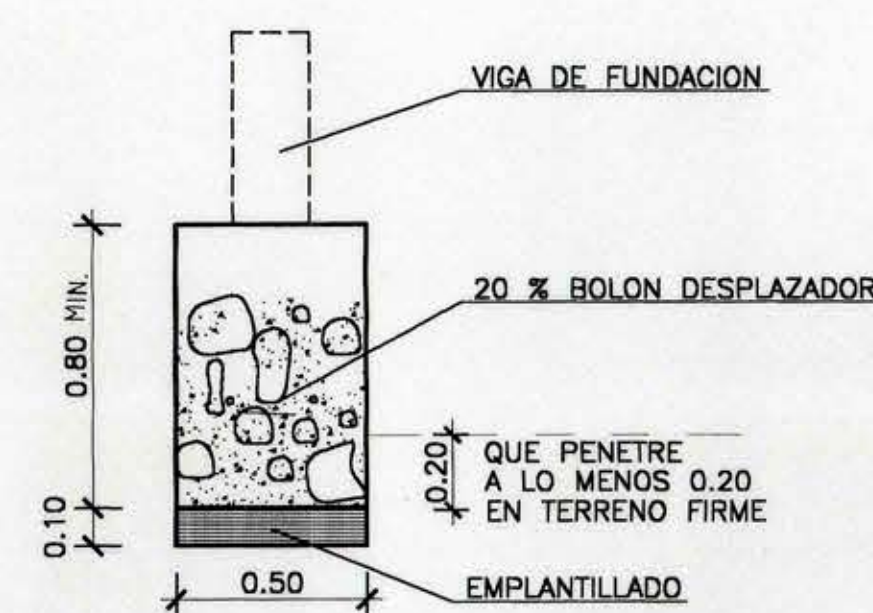
POYO TIPO ESCALA 1 : 20
