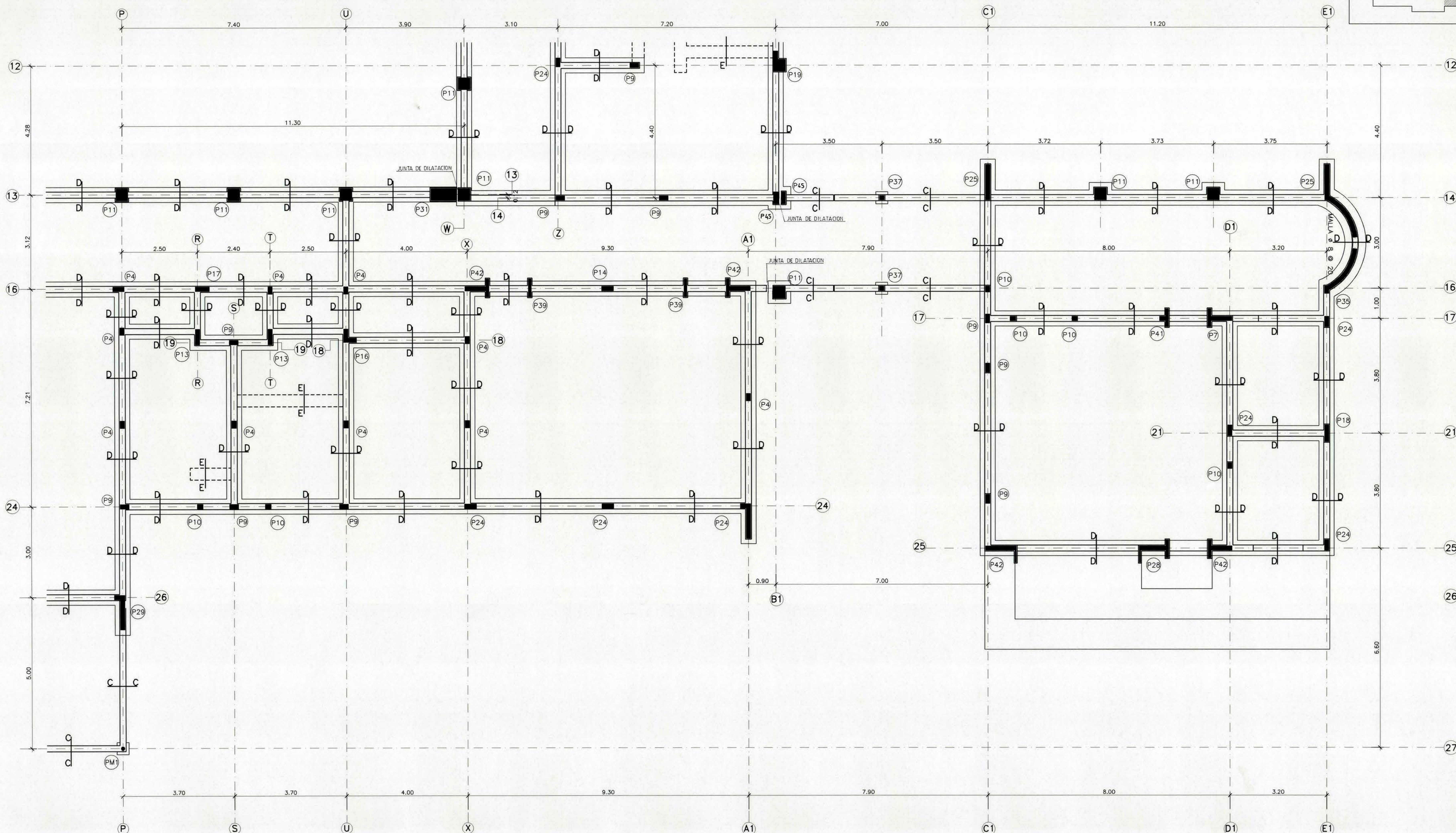
PLANTA DE FUNDACIONES MODULO C
