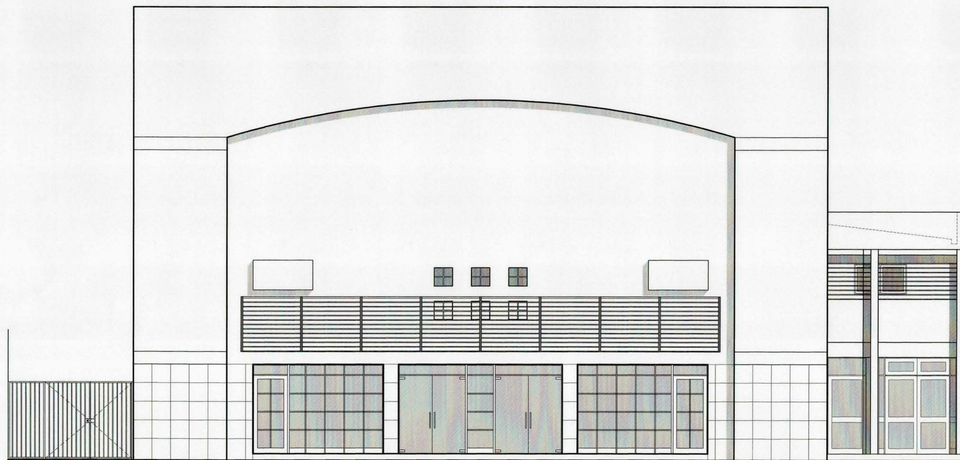
ELEVACION PRINCIPAL ESCALA 1:50
