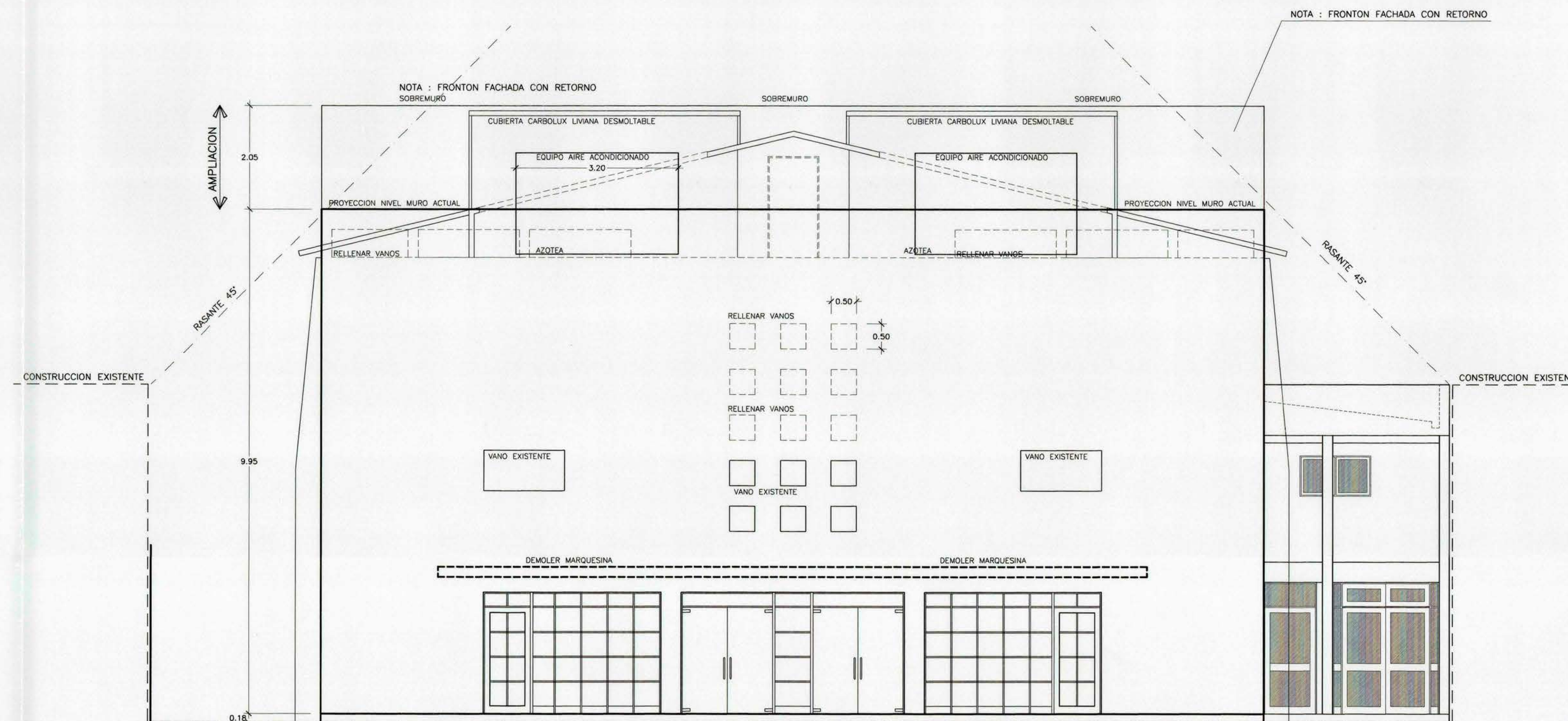
ELEVACION PRINCIPAL A MODIFICAR ESCALA 1:50
