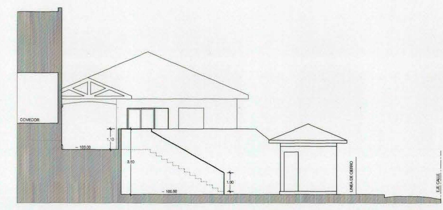
CORTE ESQUEMATICO B-B
