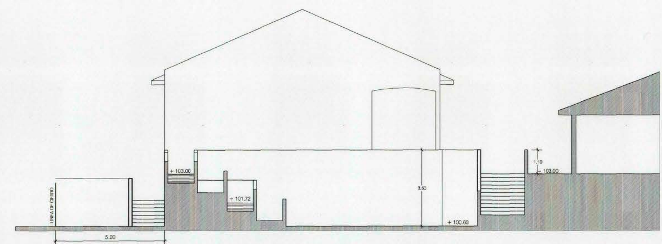
CORTE ESQUEMATICO A-A
