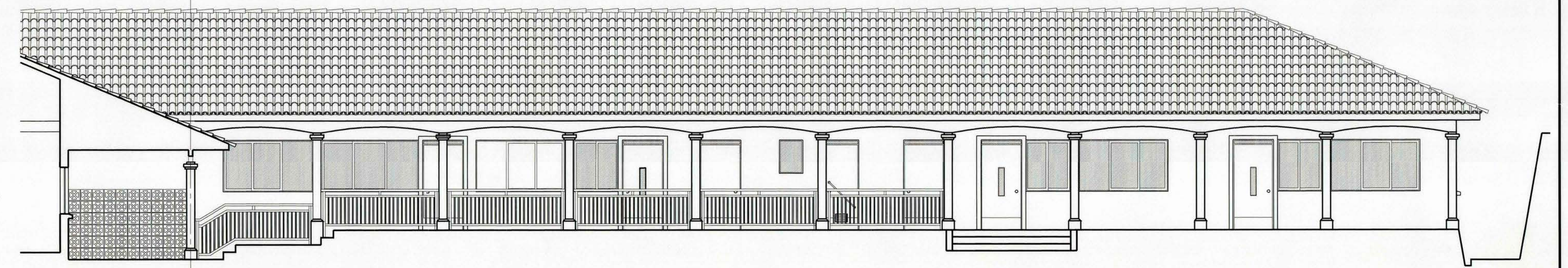
CORTE FACHADA SUR ORIENTE
