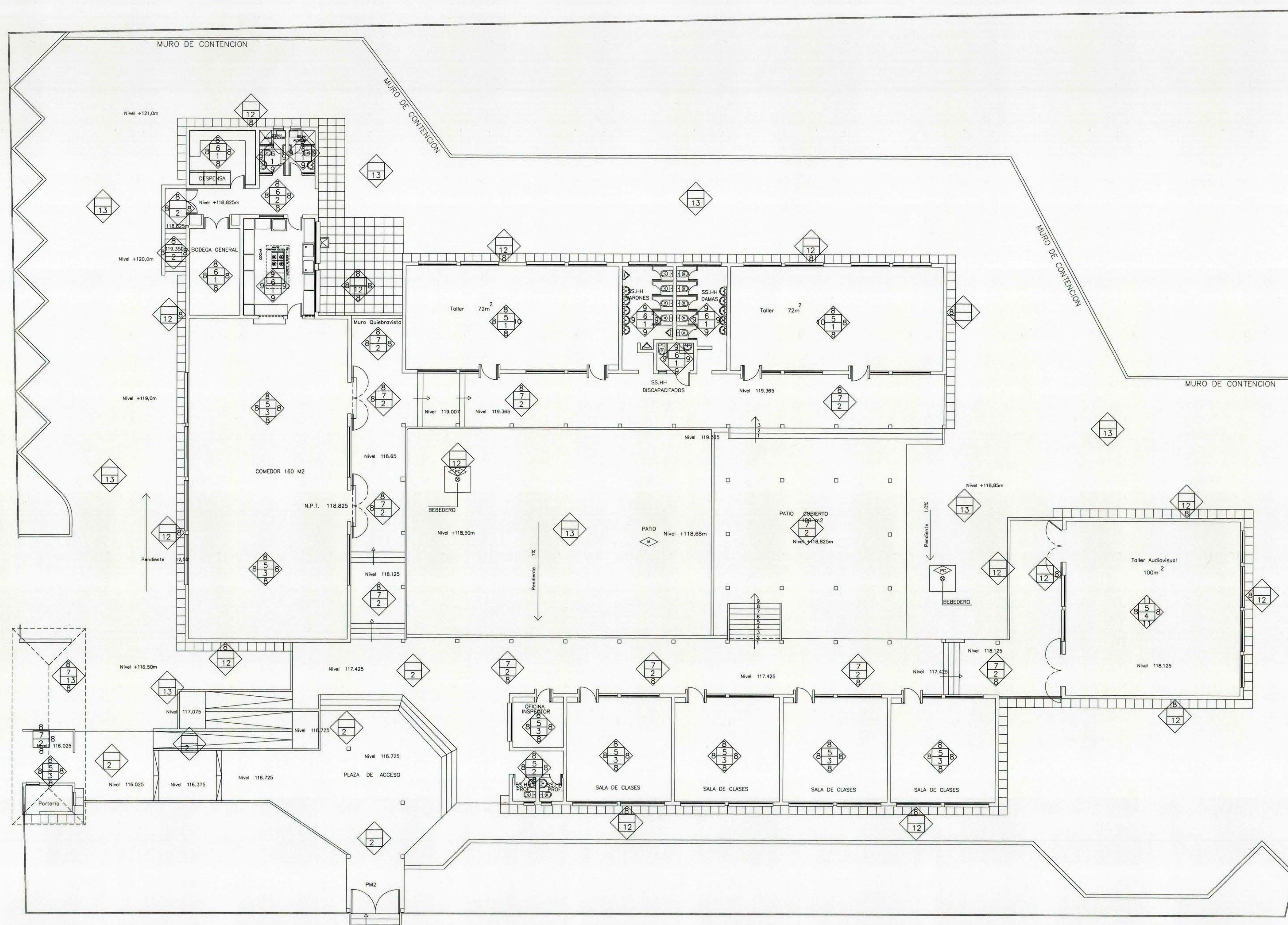
PLANTA GENERAL DE PAVIMENTOS
