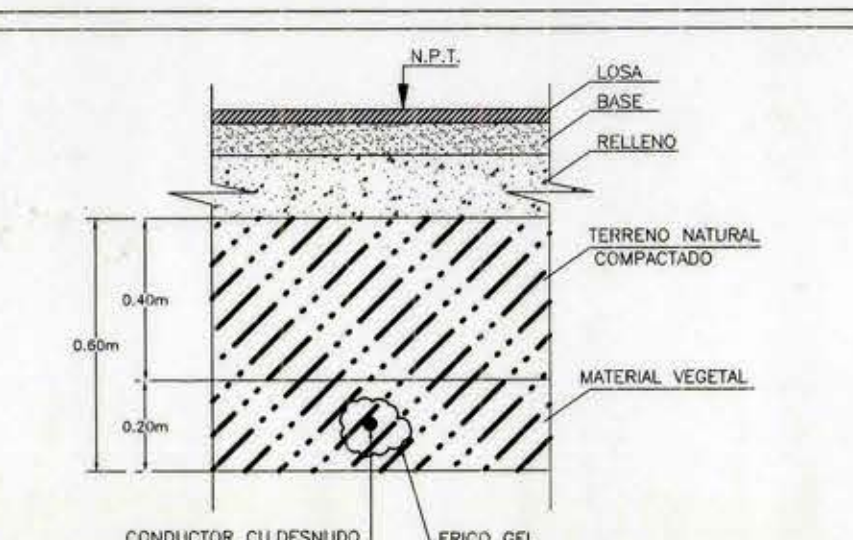
INSTALACIÓN CONDUCTOR MALLA DE TIERRA
