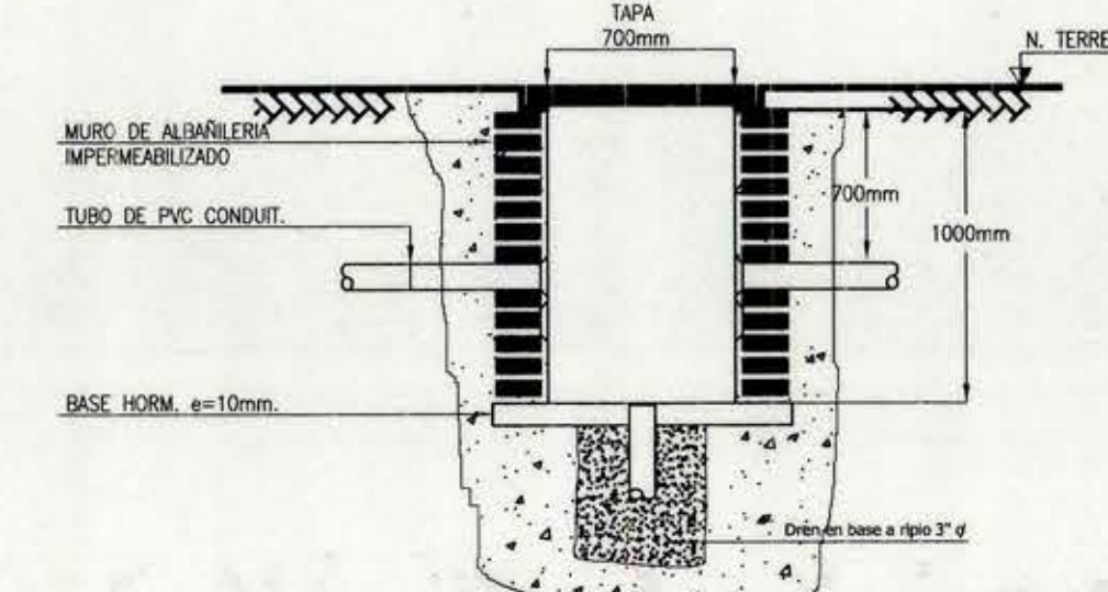
DETALLE DE CÁMARA TIPO B S/ESCALERA
