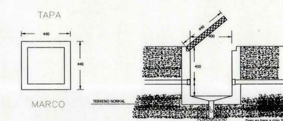
DETALLE DE CÁMARA TIPO C S/ESCALERA
