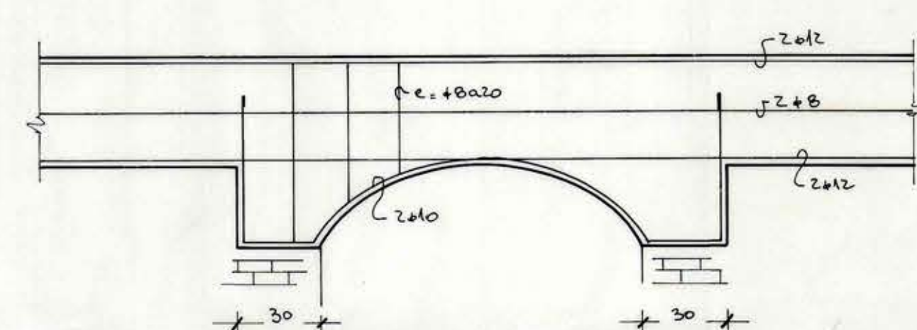
DETALLE - ARCO (TIP)
