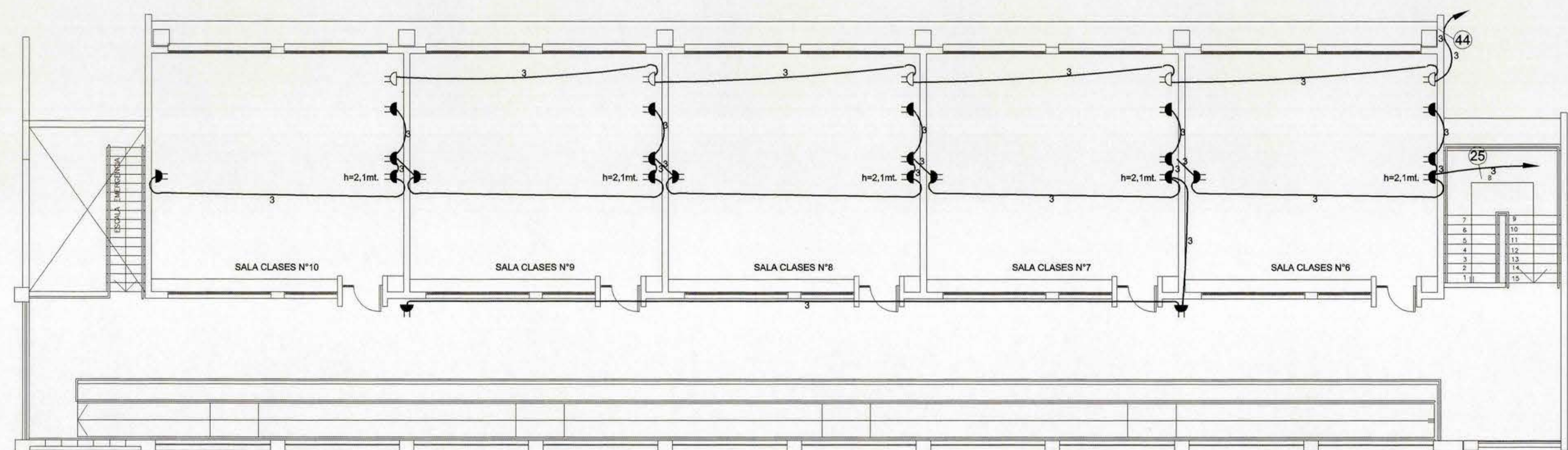
PLANTA 2° PISO ENCHUFES ESCALA 1 : 100
