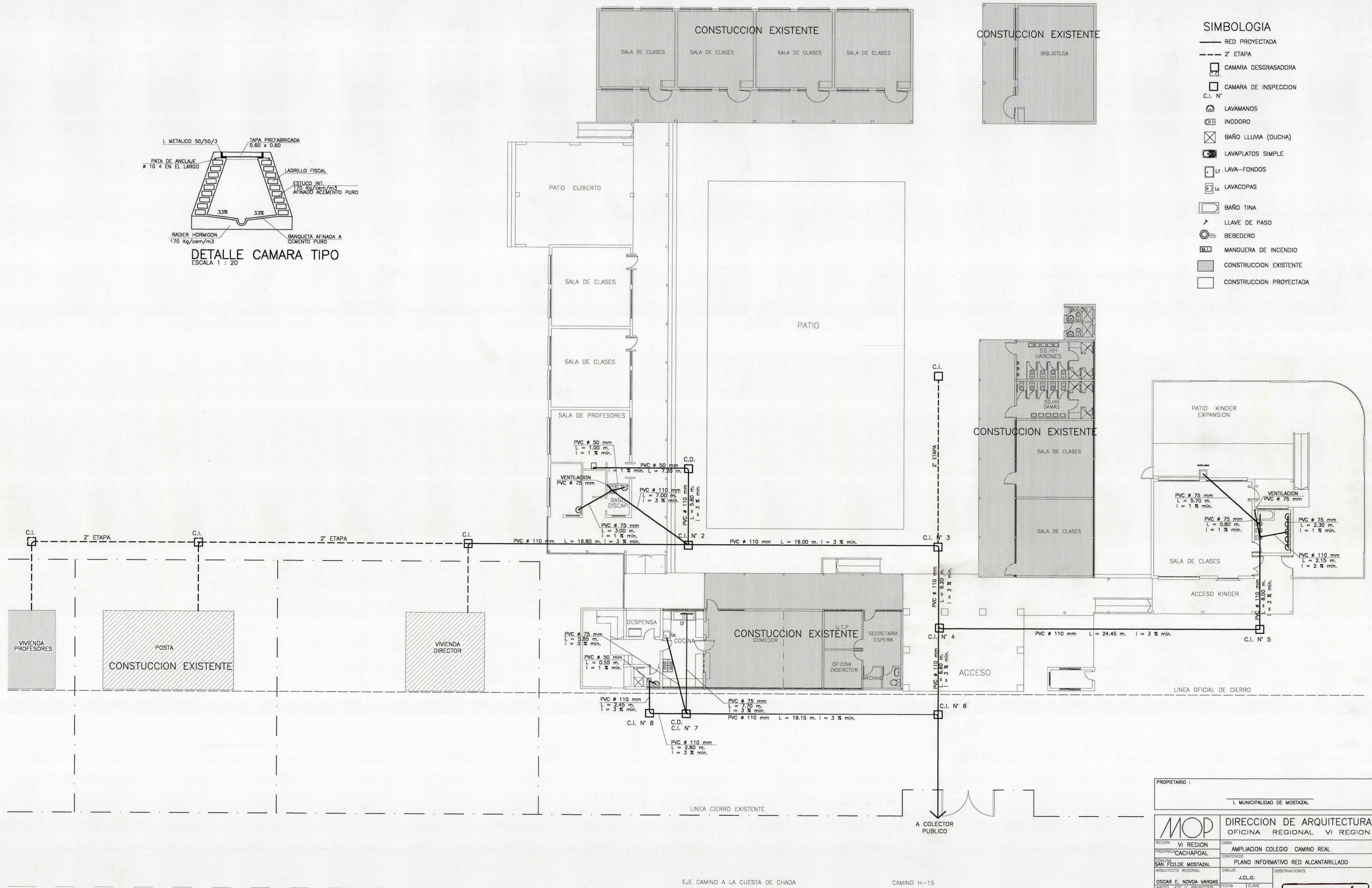
PLANTA GENERAL DE ALCANTARILLADO ESCALA 1 : 100
