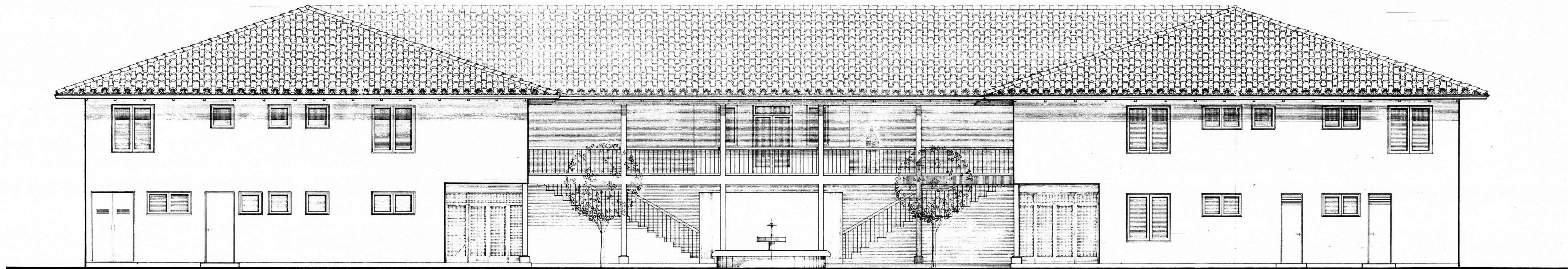
ELEVACION SUR
