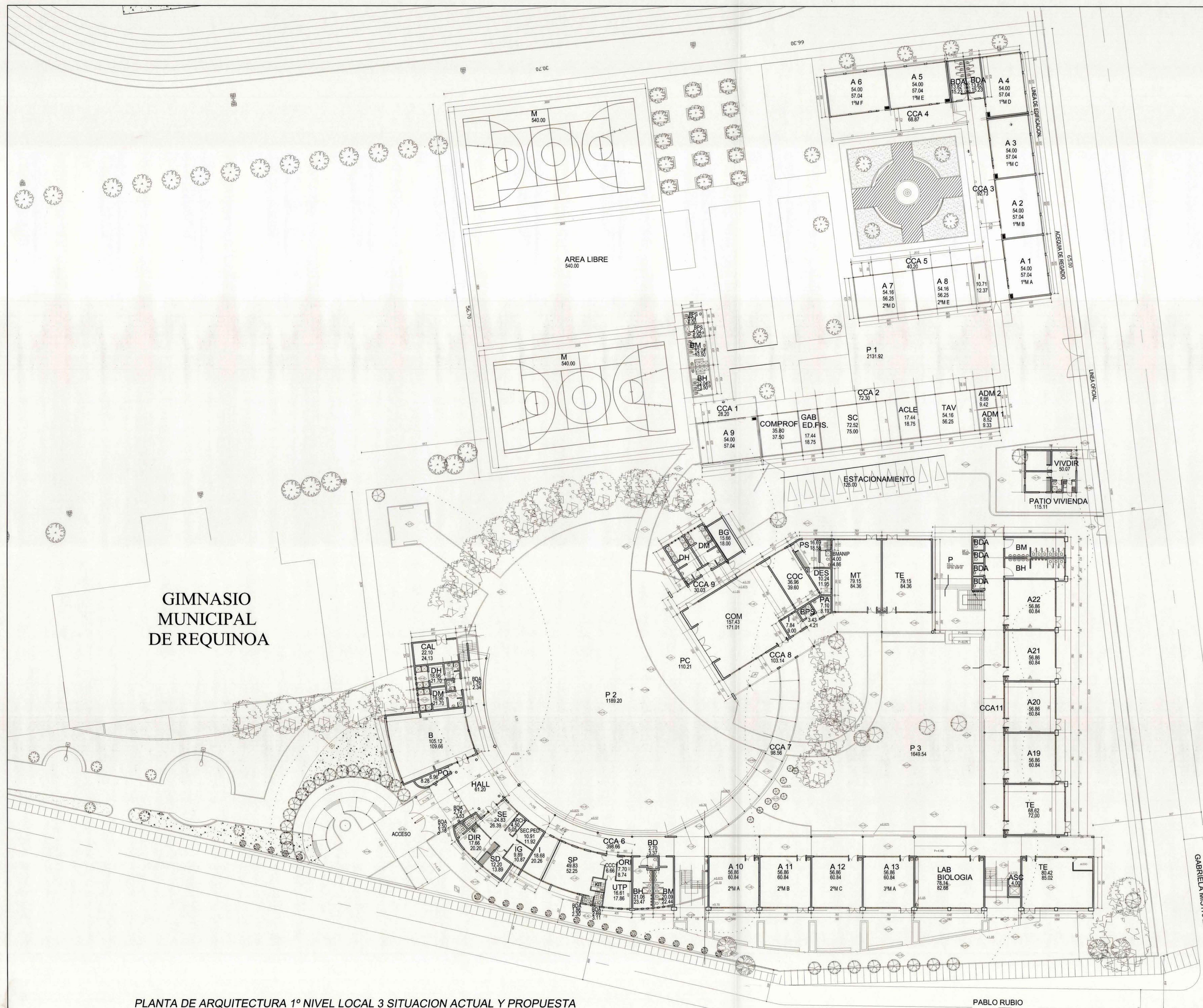
PLANTA DE ARQUITECTURA 1º NIVEL LOCAL 3 SITUACION ACTUAL Y PROPUESTA
