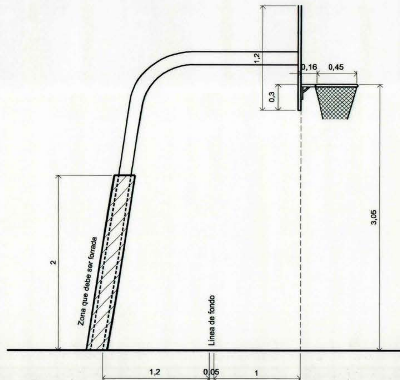
DETALLE TABLERO escala 1:25
