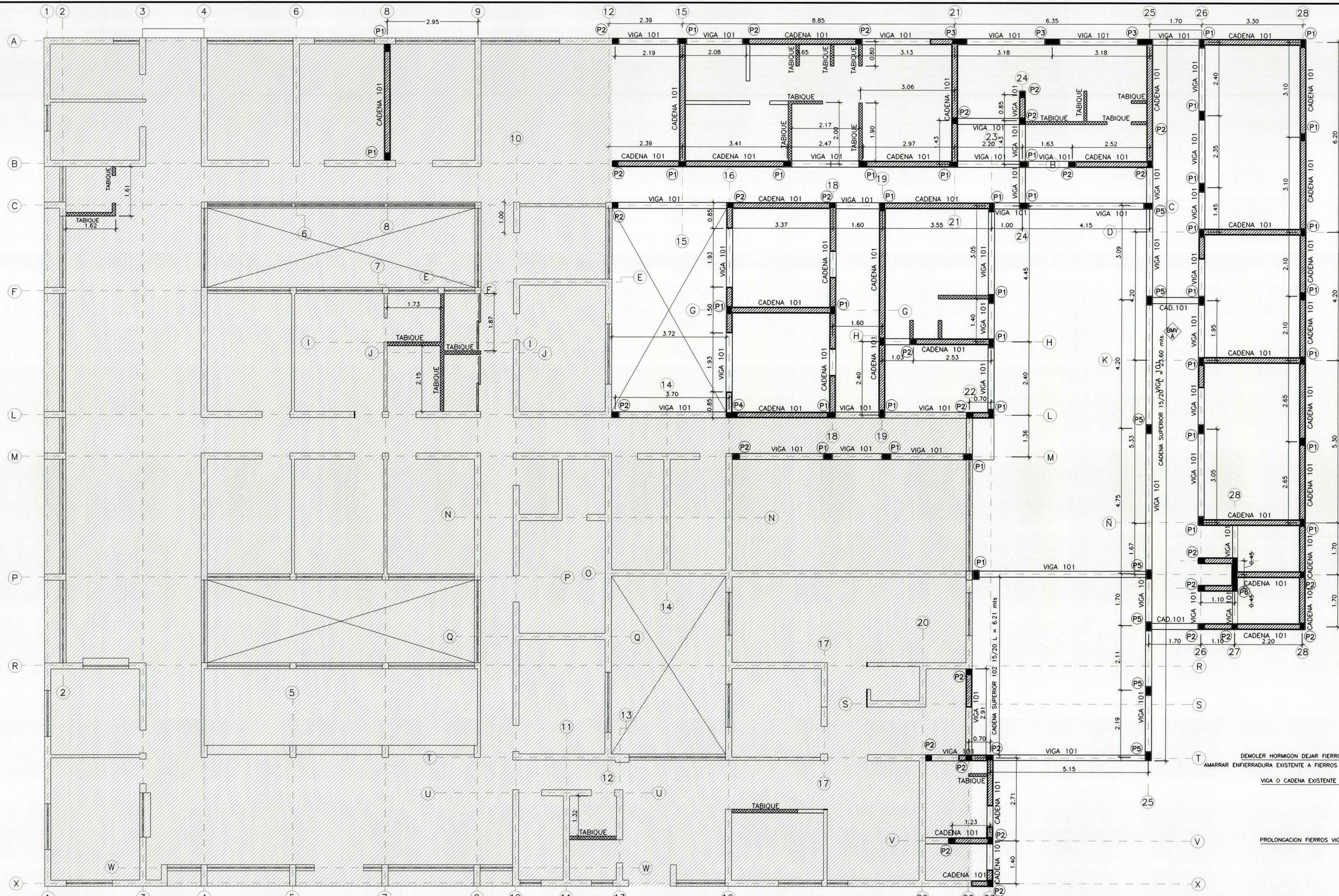
PLANTA DE ESTRUCTURAS ESCALA 1 : 50
