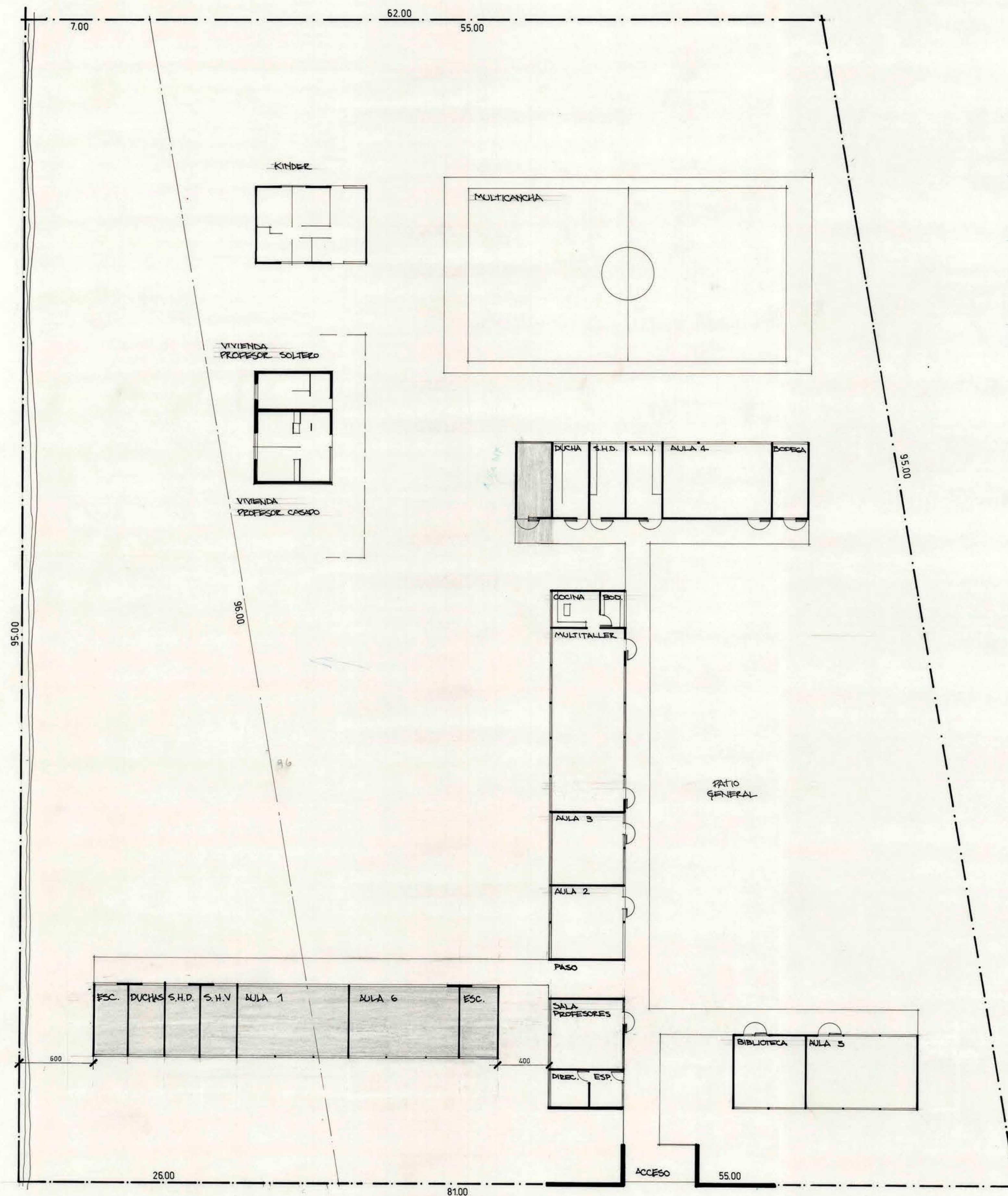
EMPLAZAMIENTO ESCALA 1: 200
