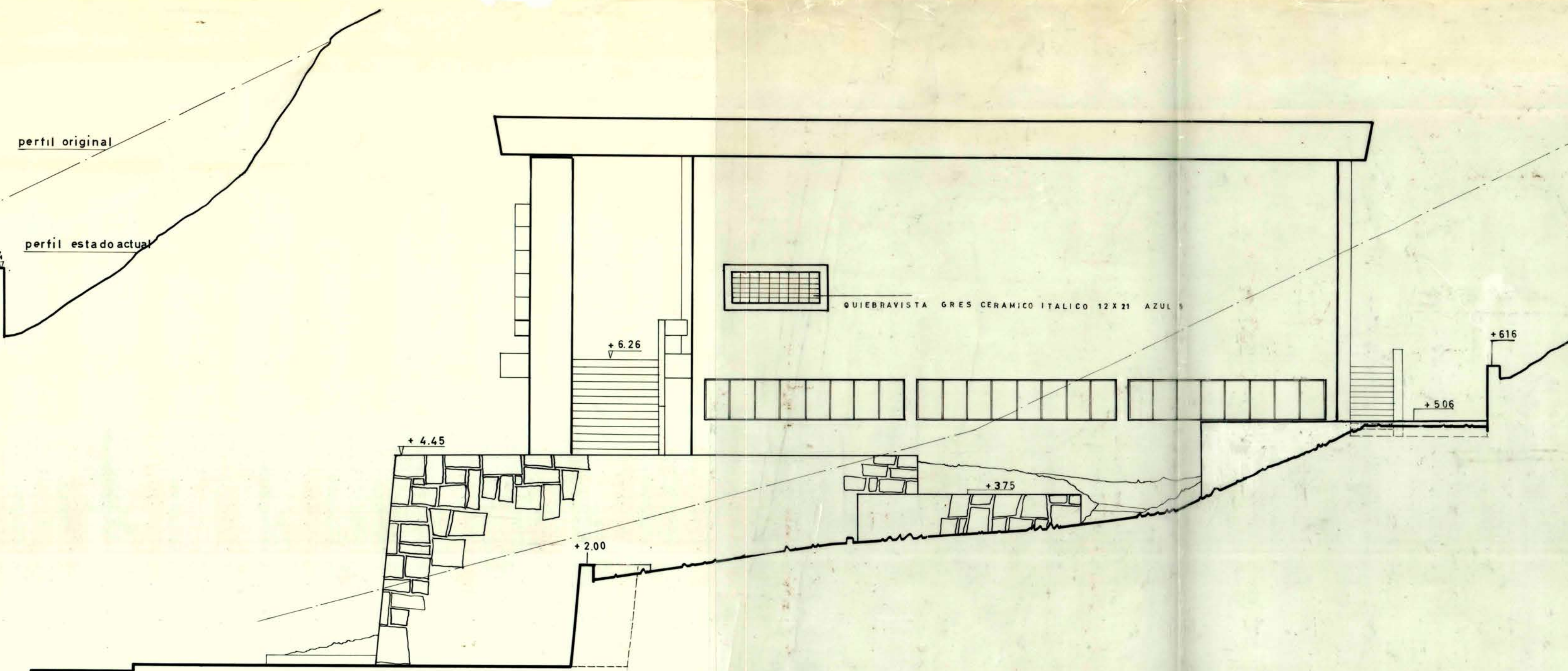
ELEVACION SUR.
