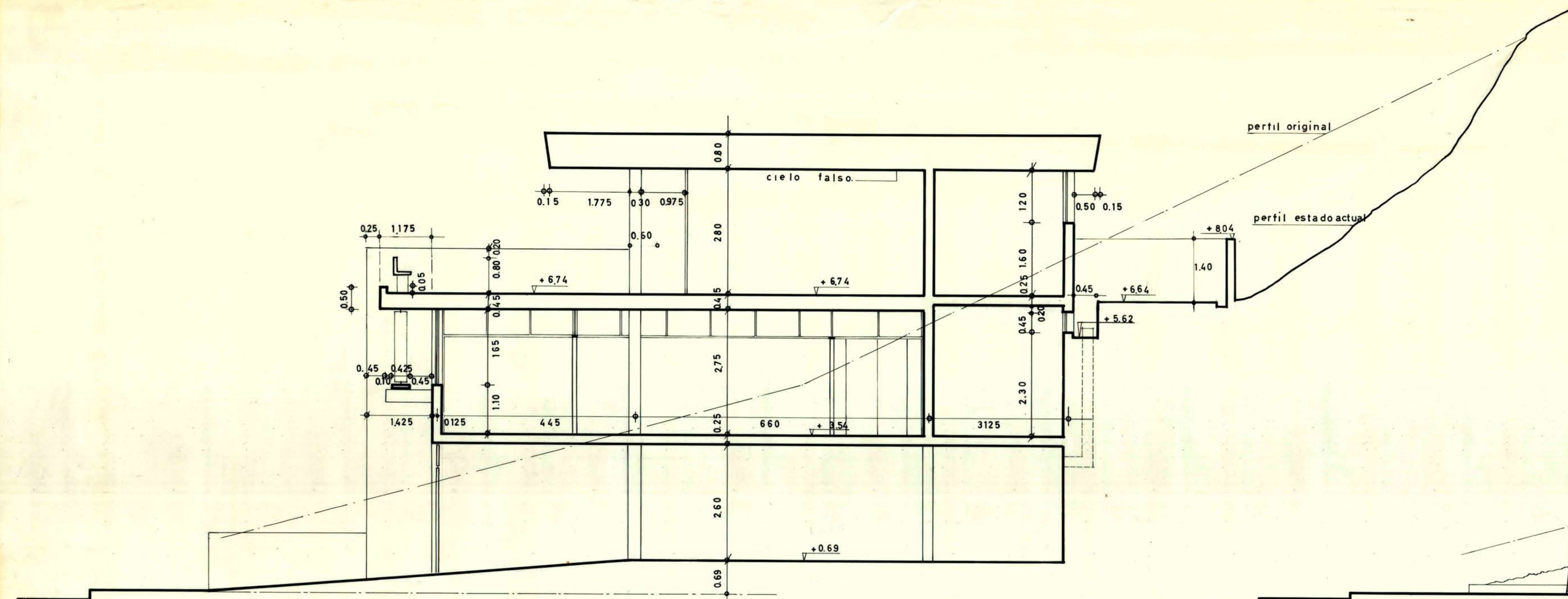
SECCION A A.
