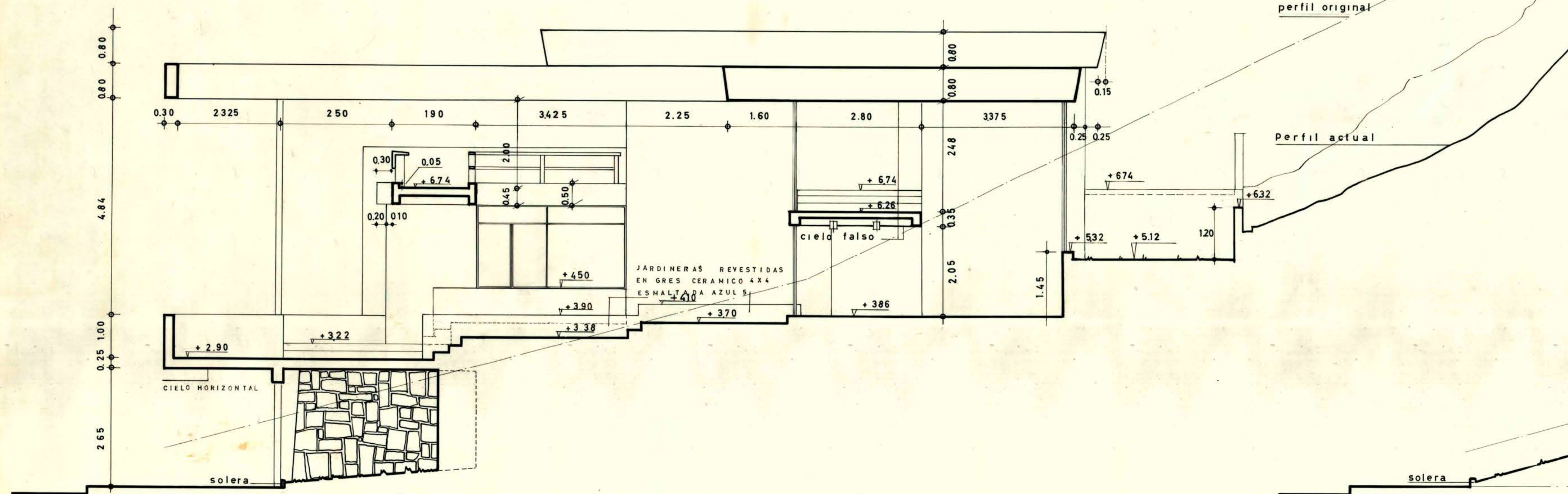
SECCION BB
