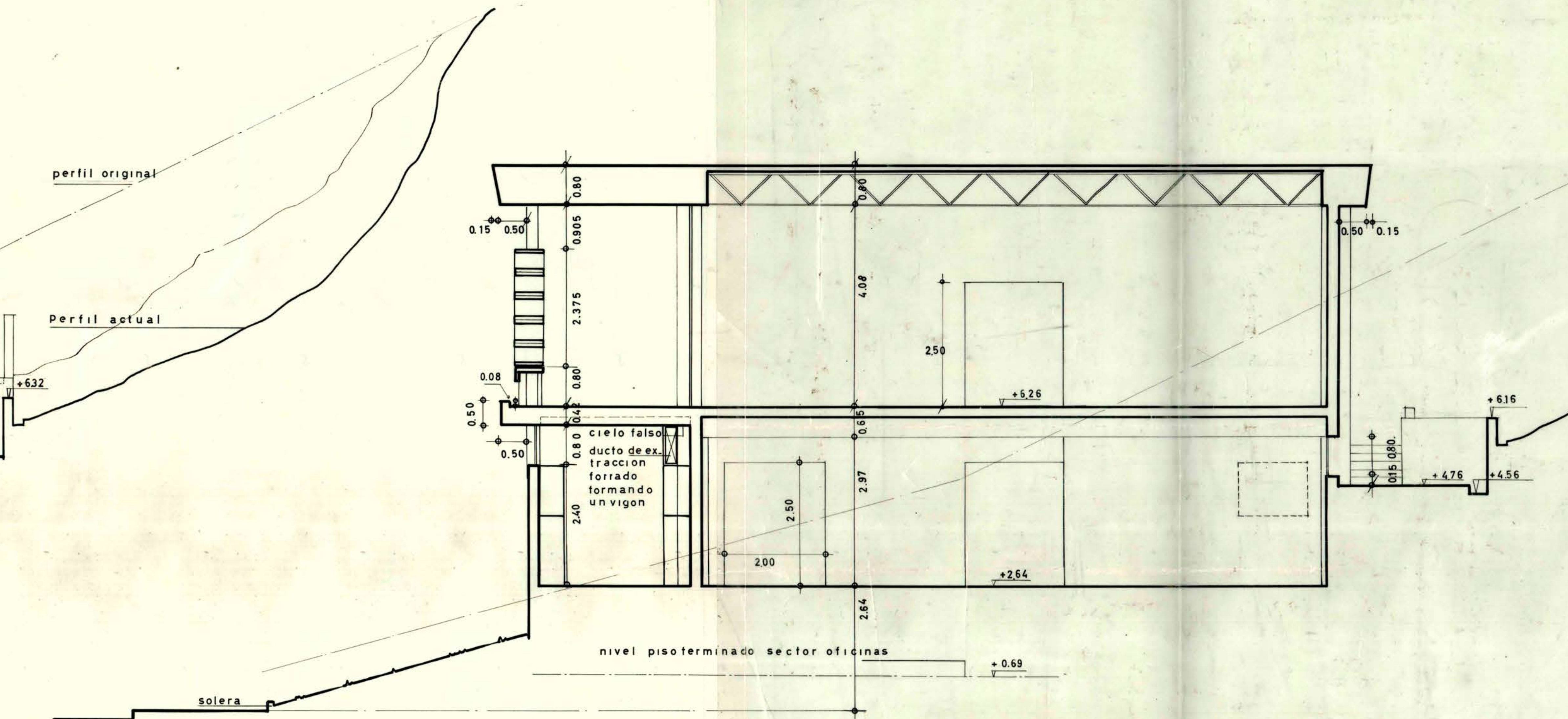
SECCION DD
