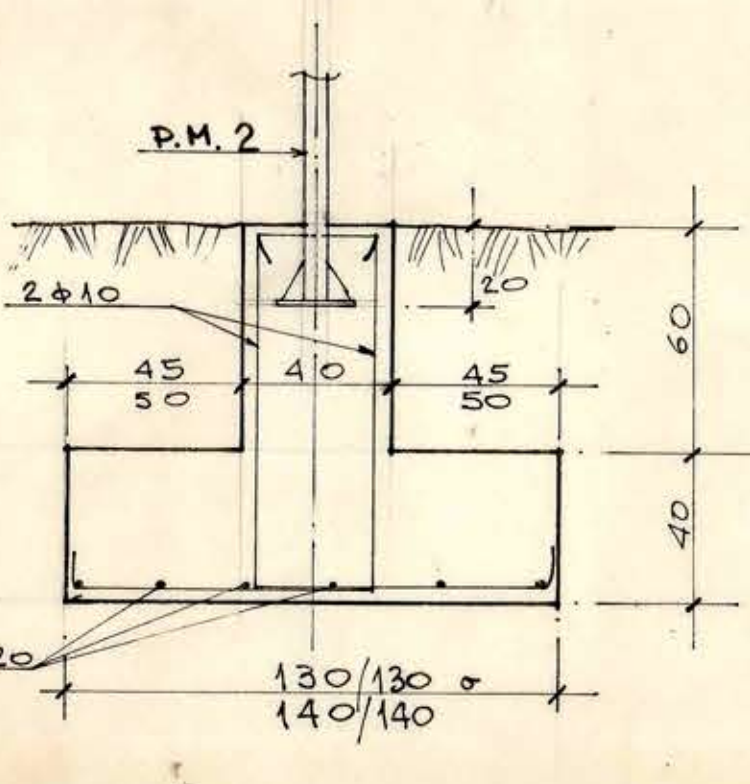
CORTE 15-15
