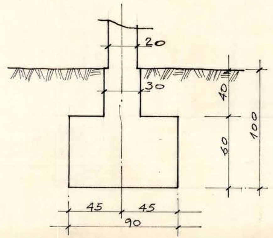
CORTE 14-14
