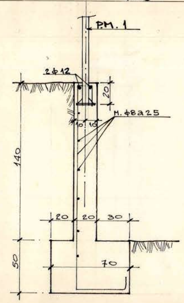
CORTE 16-16 MURO DE CONTENSION
