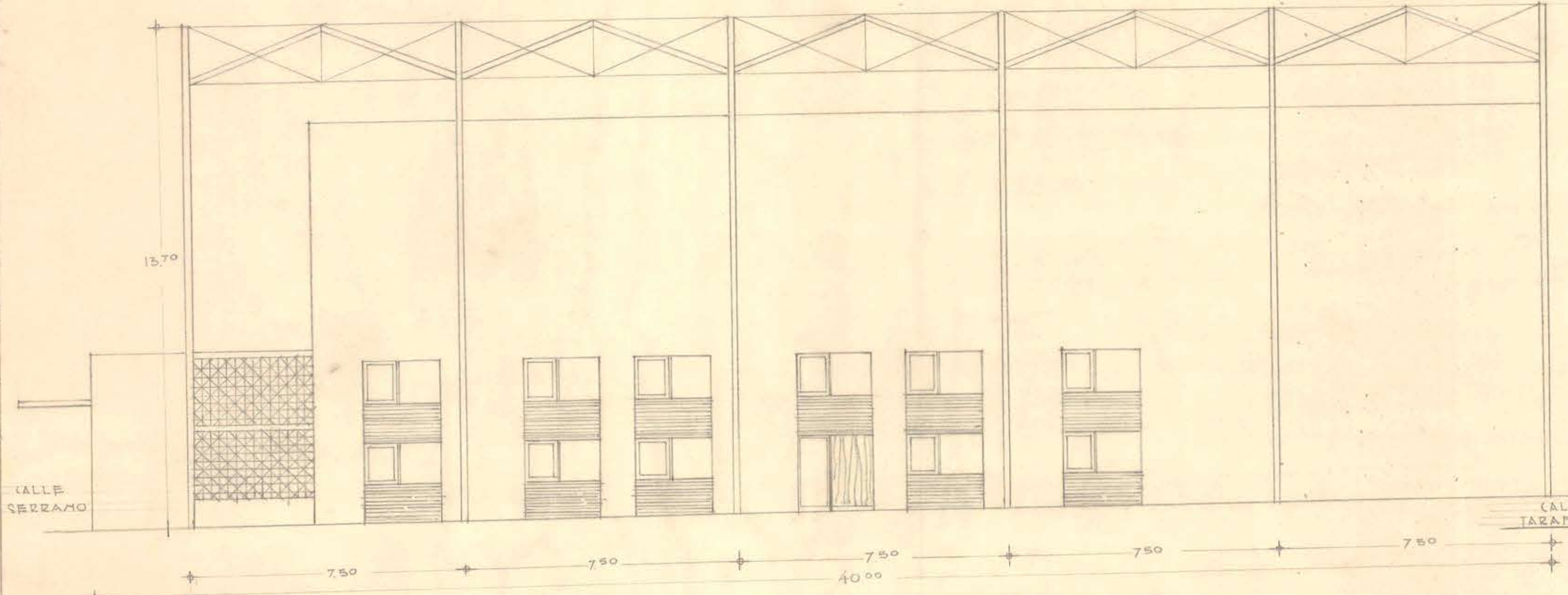
ELEVACION LATERAL.
