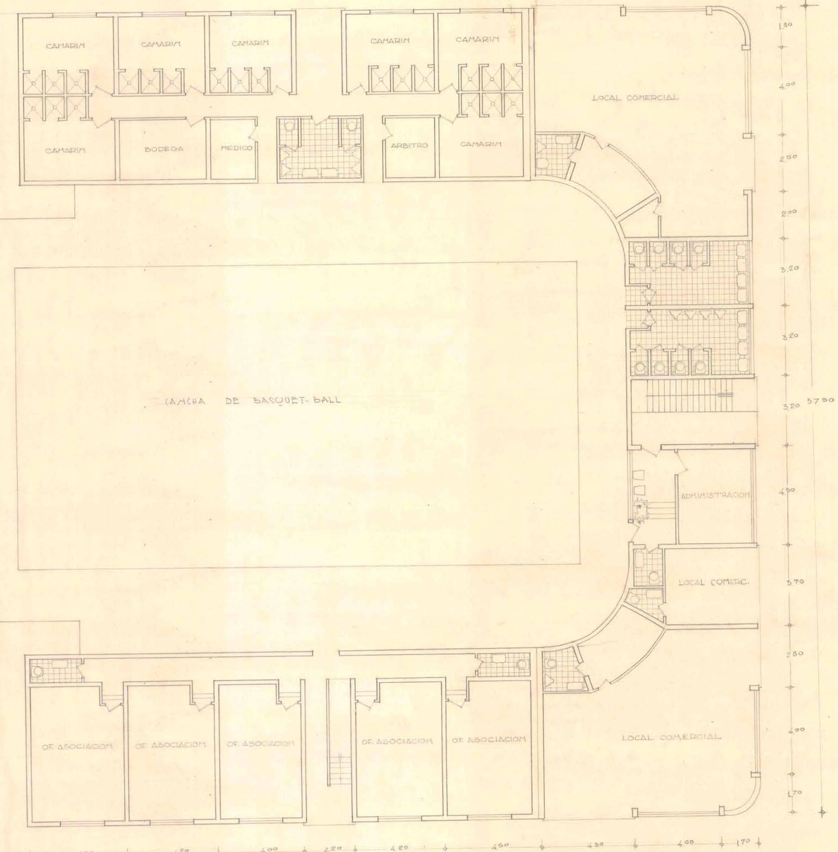
PLANTA PRIMER PISO.
