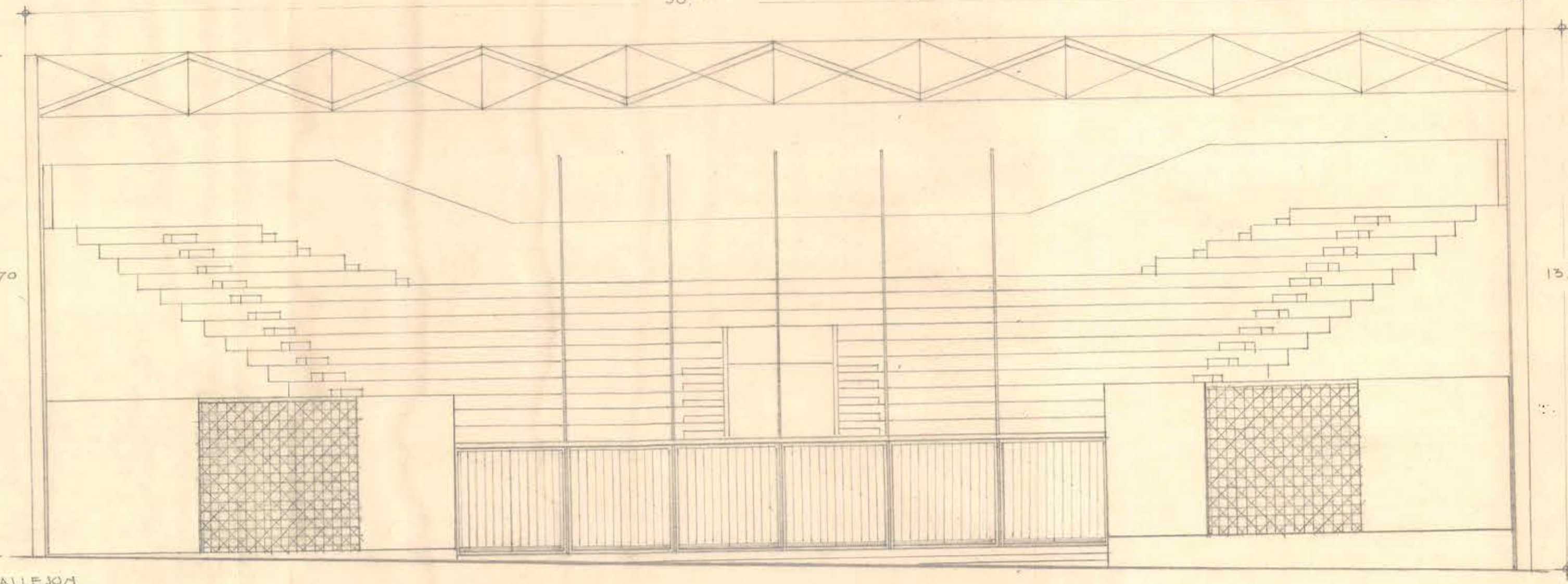
ELEVACION FACHADA PRINCIPAL.
