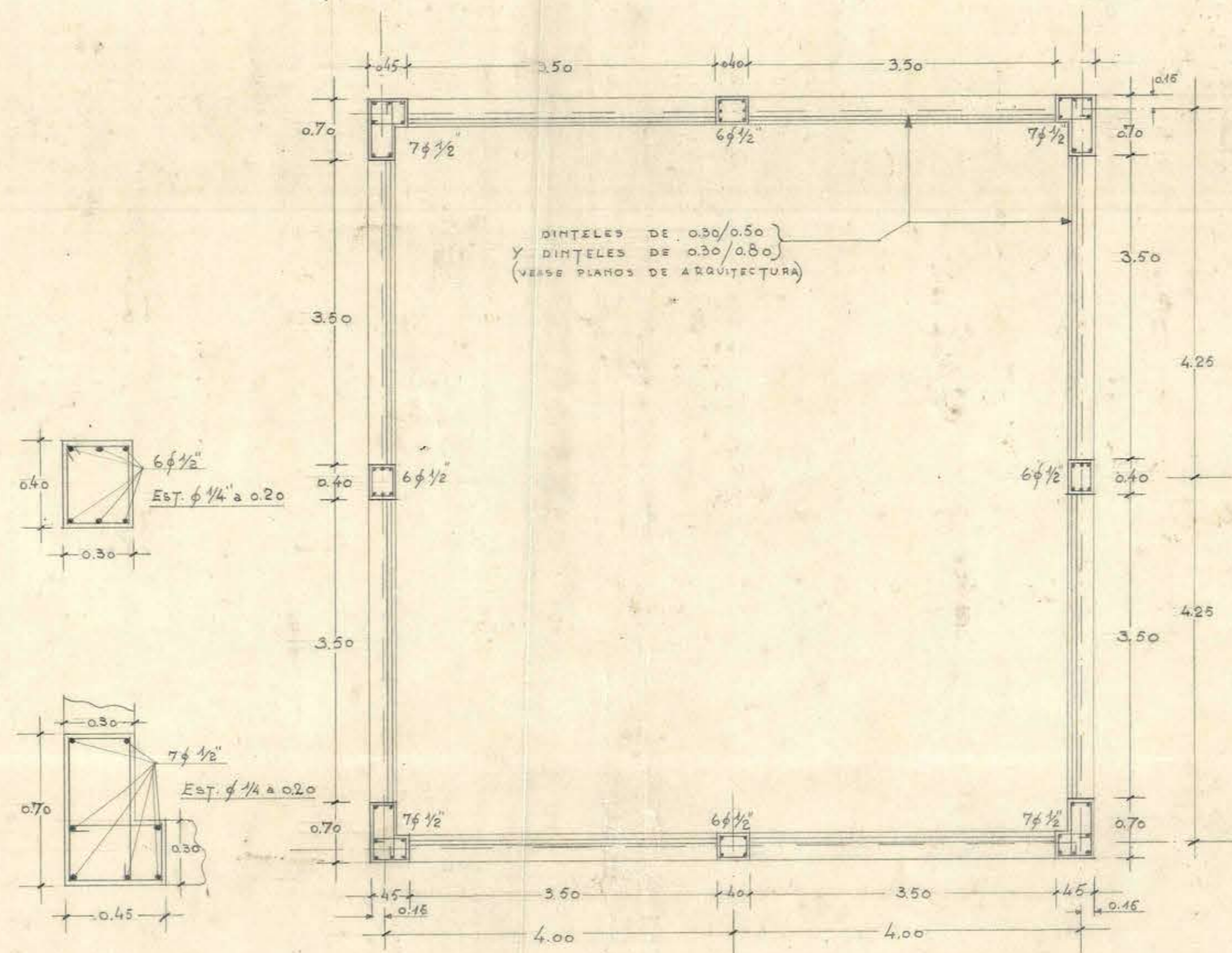
PLANTA DE LA TORRE
