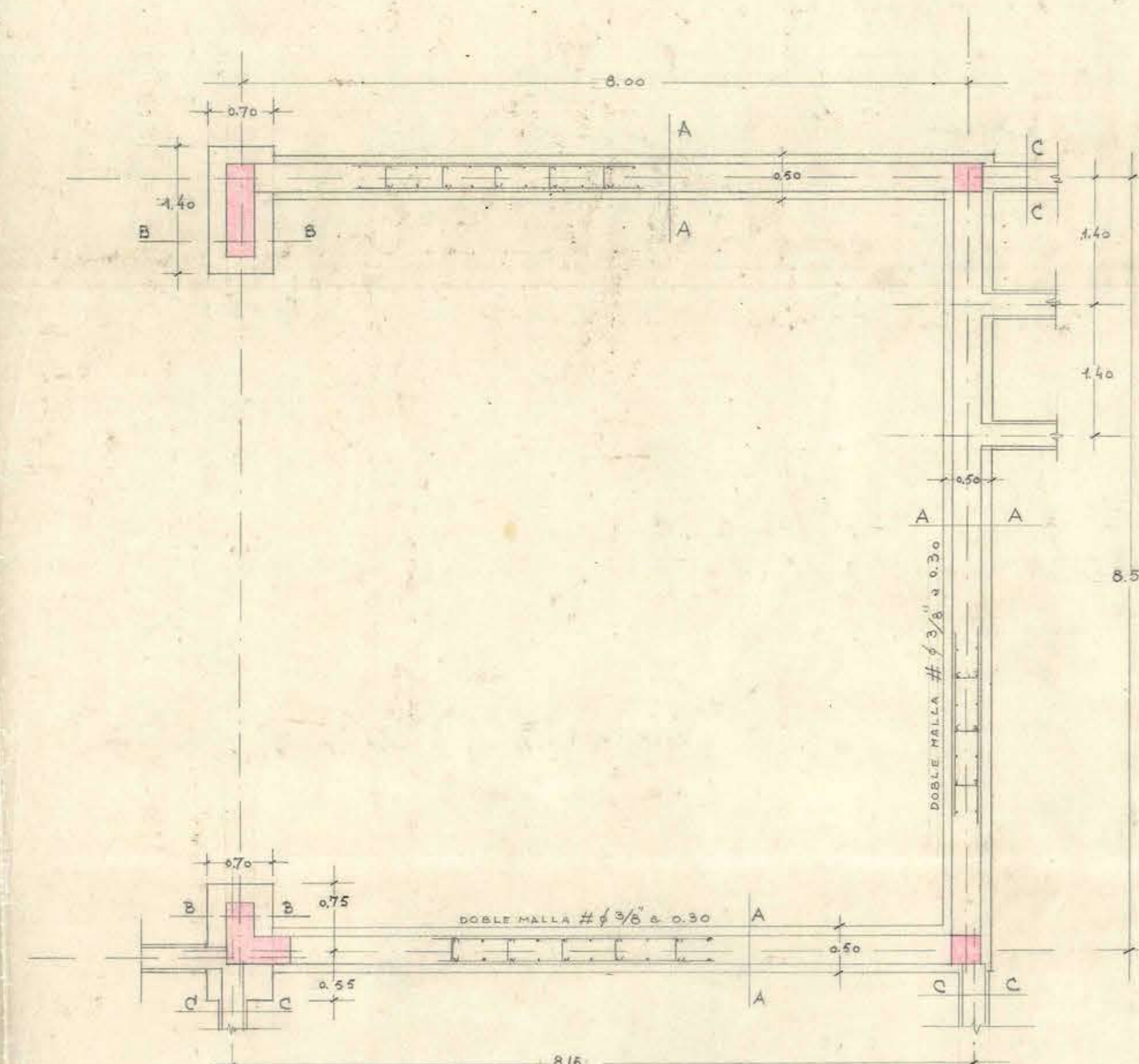
PLANTA DE CIMENTOS
