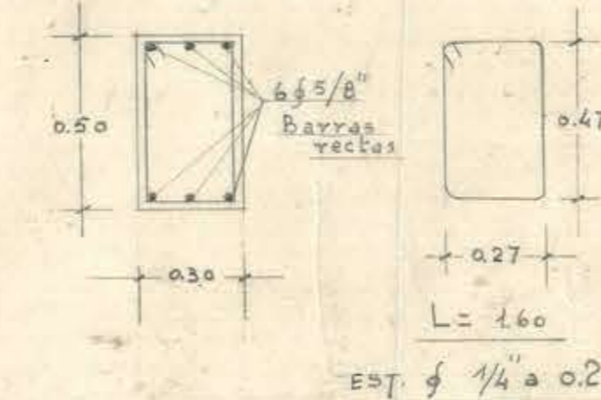
DINTEL EN CONTORNO EN 2º PISO
