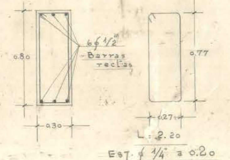
DINTEL EN CONTORNO 3er PISO
