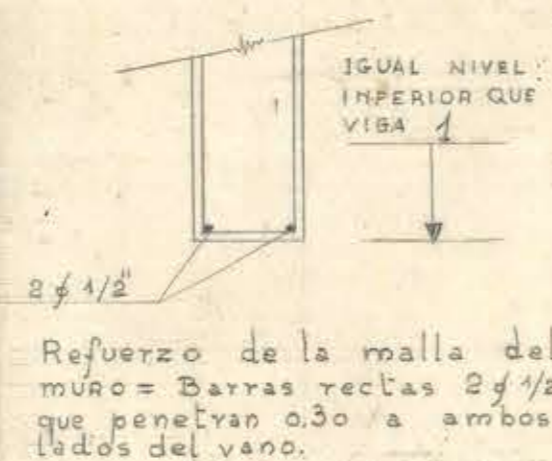
DINTELES D1, D2, D3
