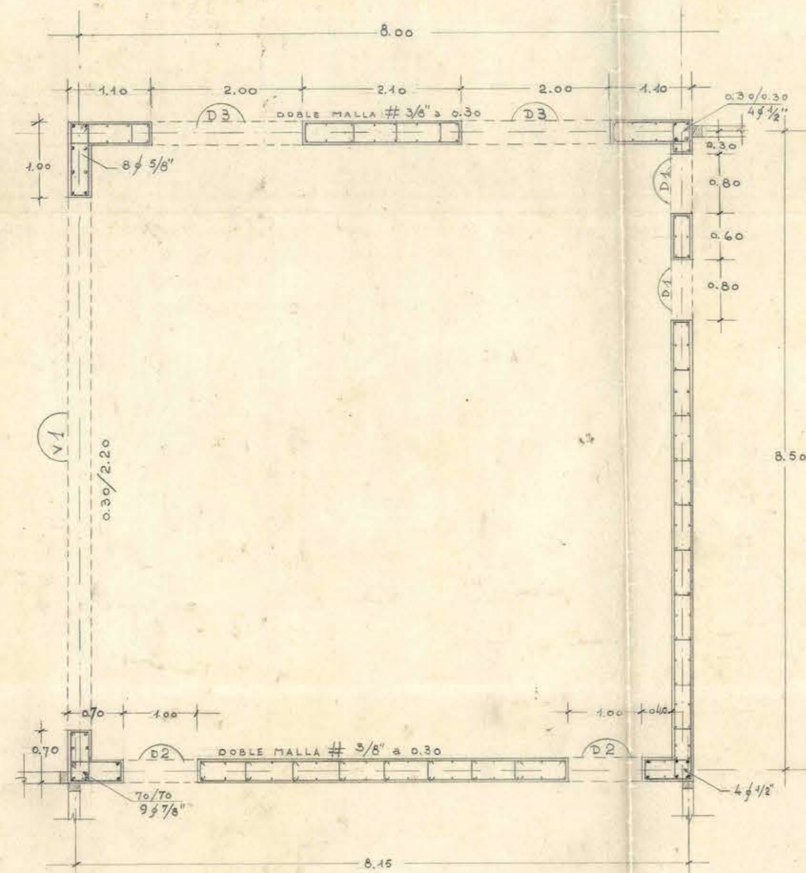
PLANTA 1er PISO
