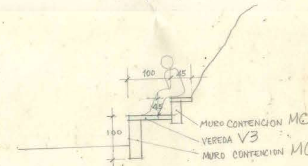
CORTE C 1:50
