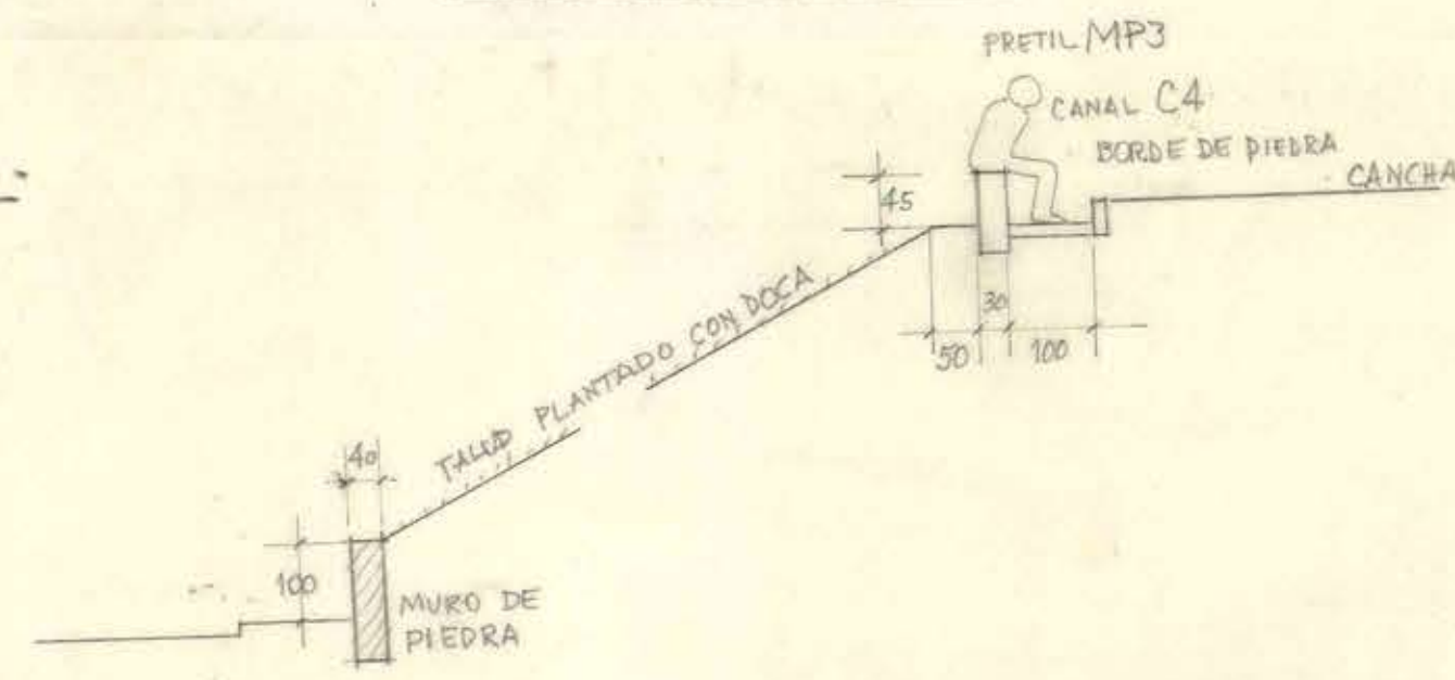
CORTE A 1:100
