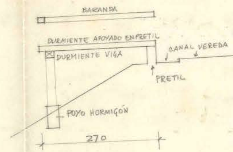
CORTE B 1:50
