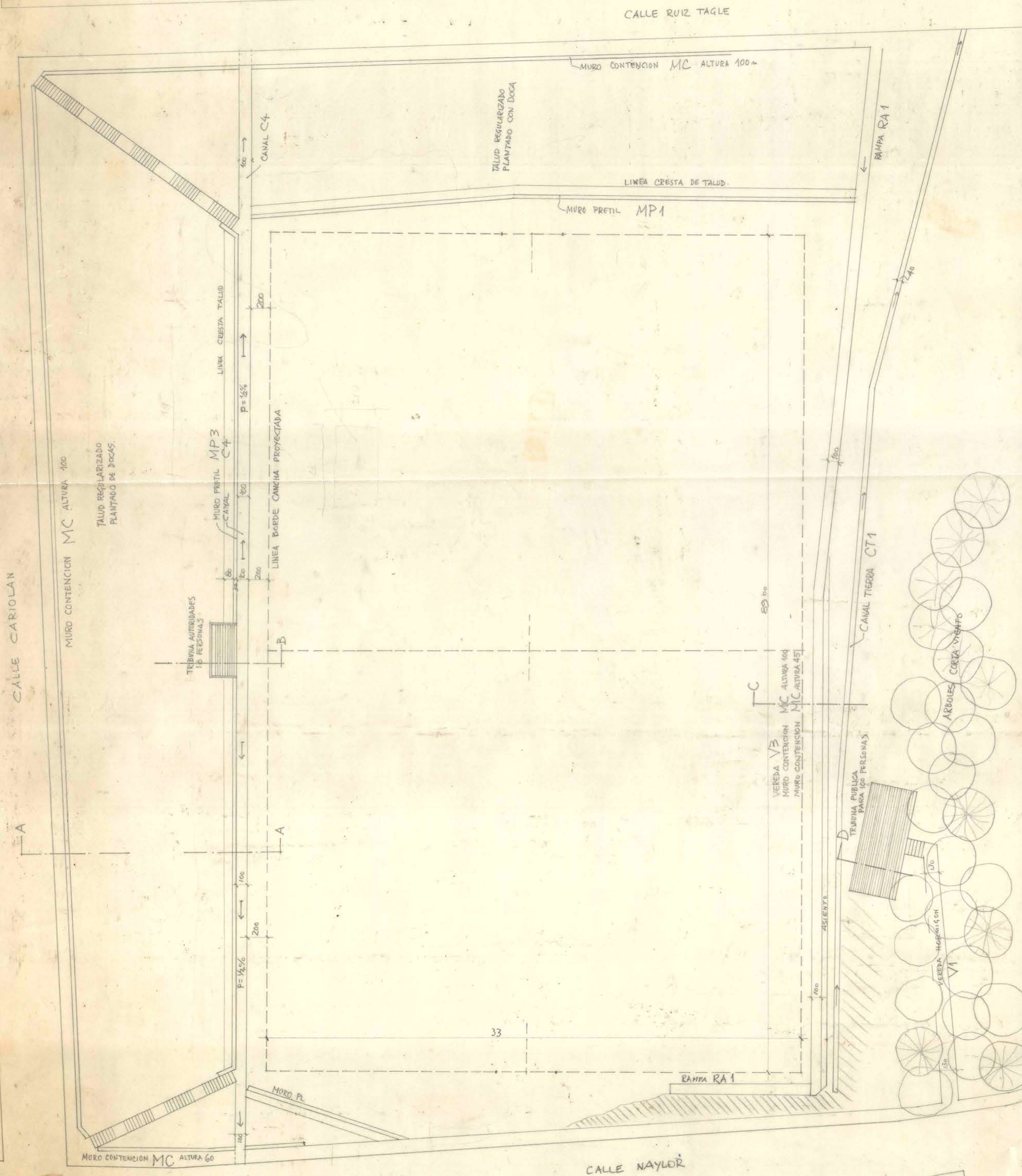
PLANTA GENERAL ESC. 1:200
