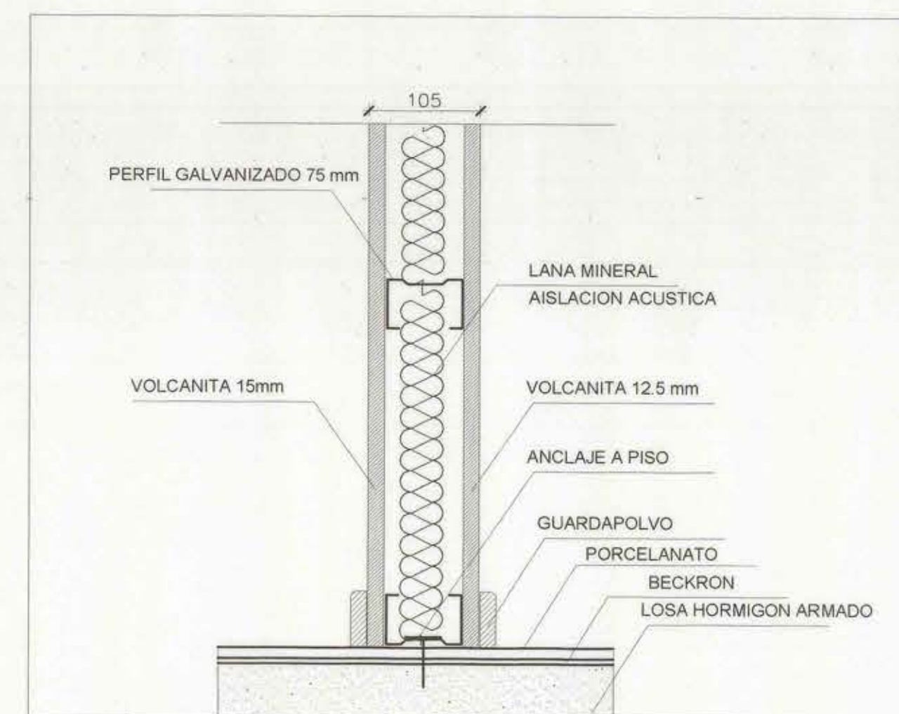
DETALLE MODULO AEROBRIS / (planta tipo) ESC. 1:10
