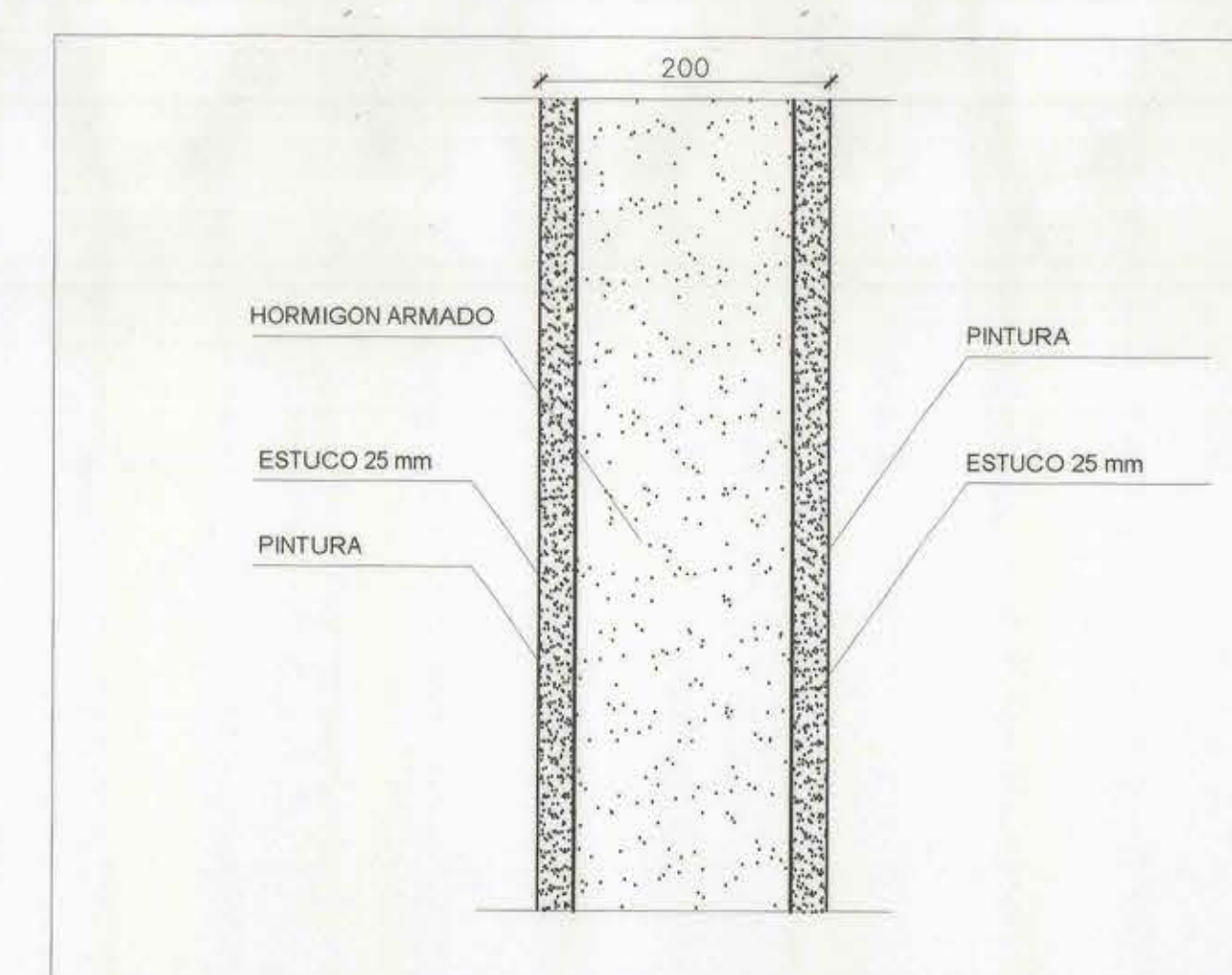
DETALLE 2 ESC. 1:2
