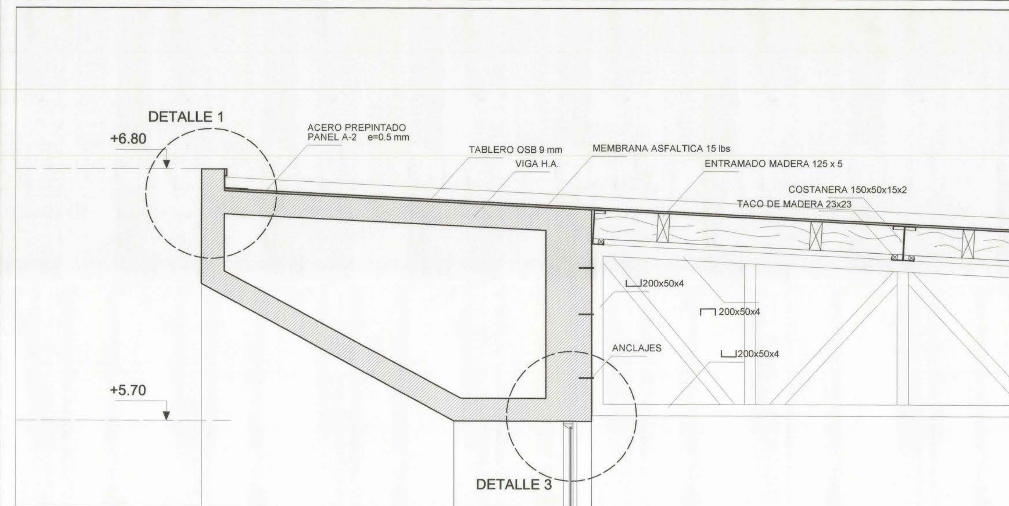
ESCANTILLON ALERO FACHADA PRINCIPAL ESC. 1:10
