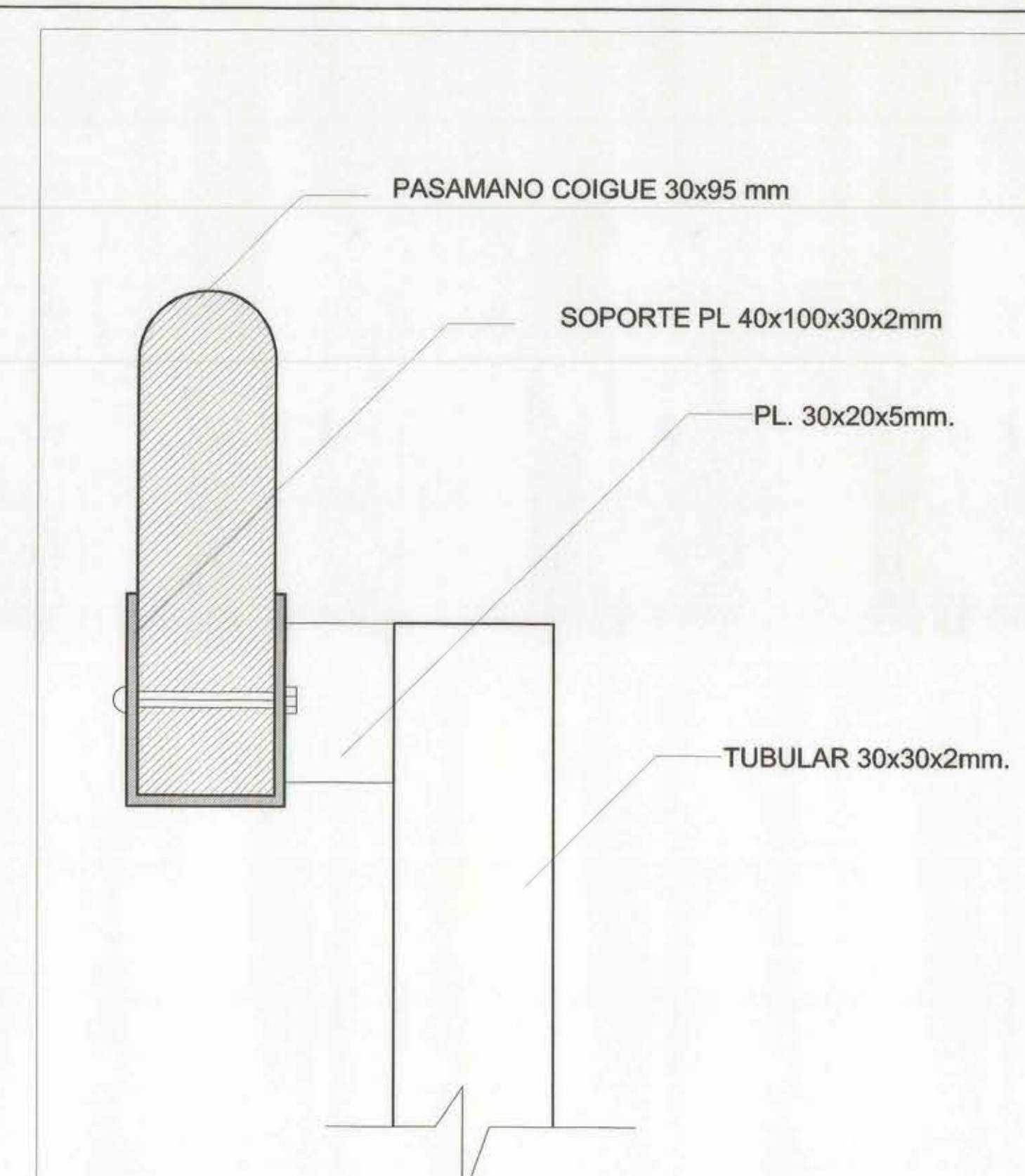
DETALLE 2 ESC. 1:2
