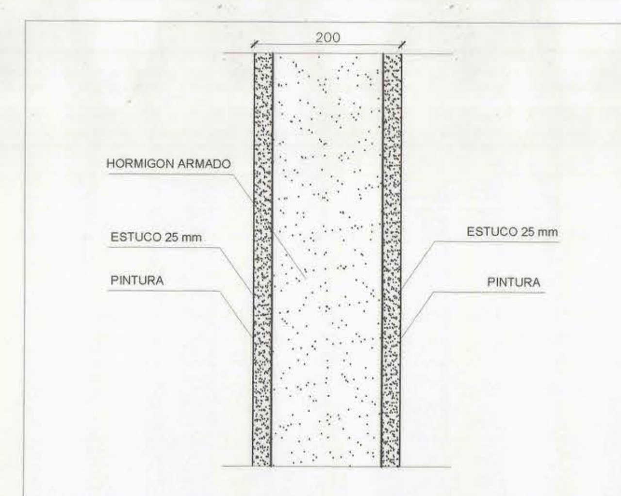
DETALLE 3 ESC. 1:2
