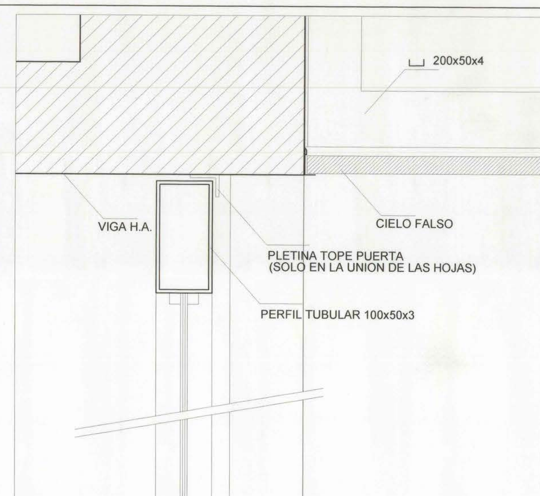
DETALLE 3 ESC. 1:2
