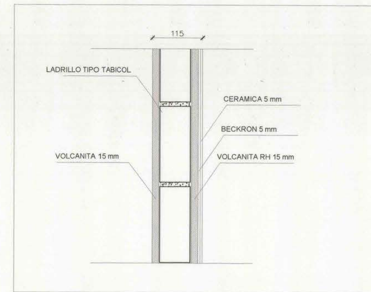
DETALLE MODULO AEROBRIS / (planta tipo) ESC. 1:10
