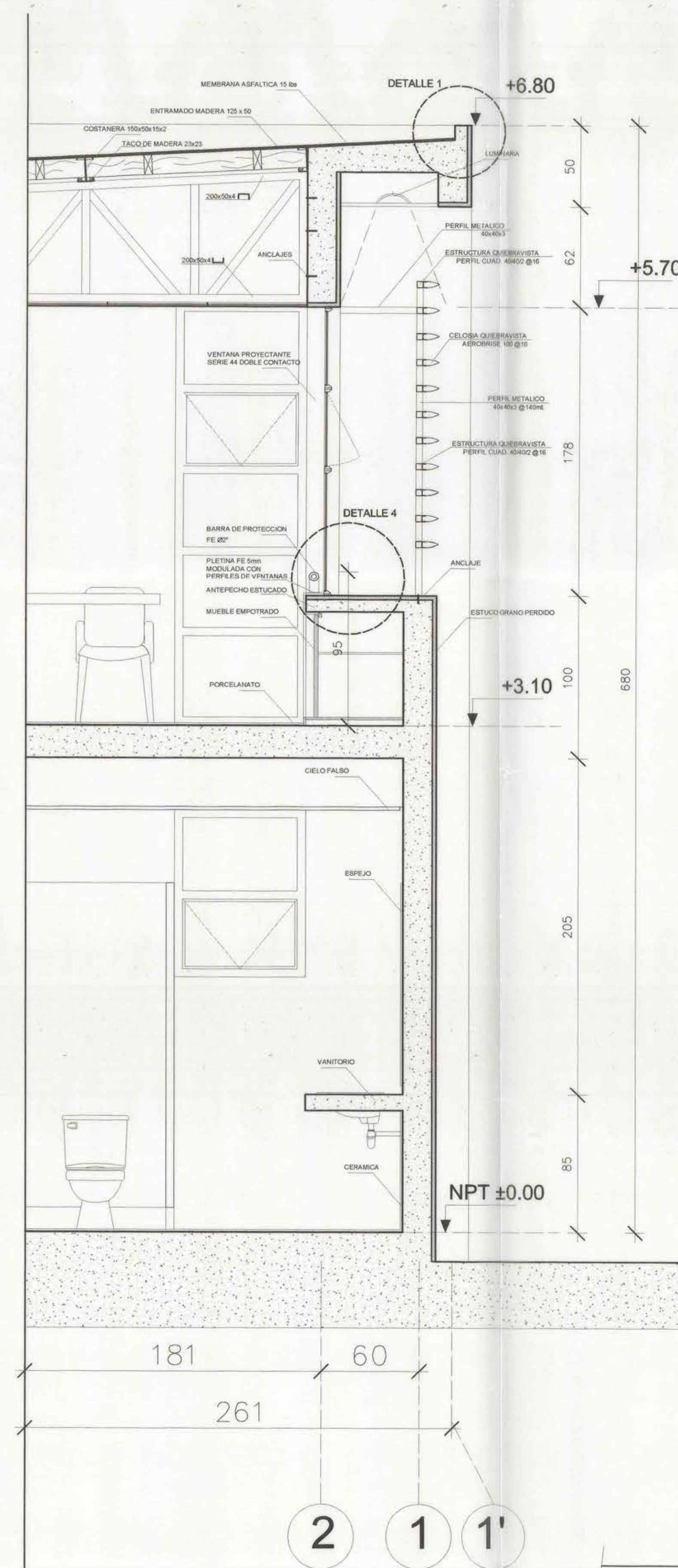
ESCANTILLON FACHADA PONIENTE ESC. 1:20
