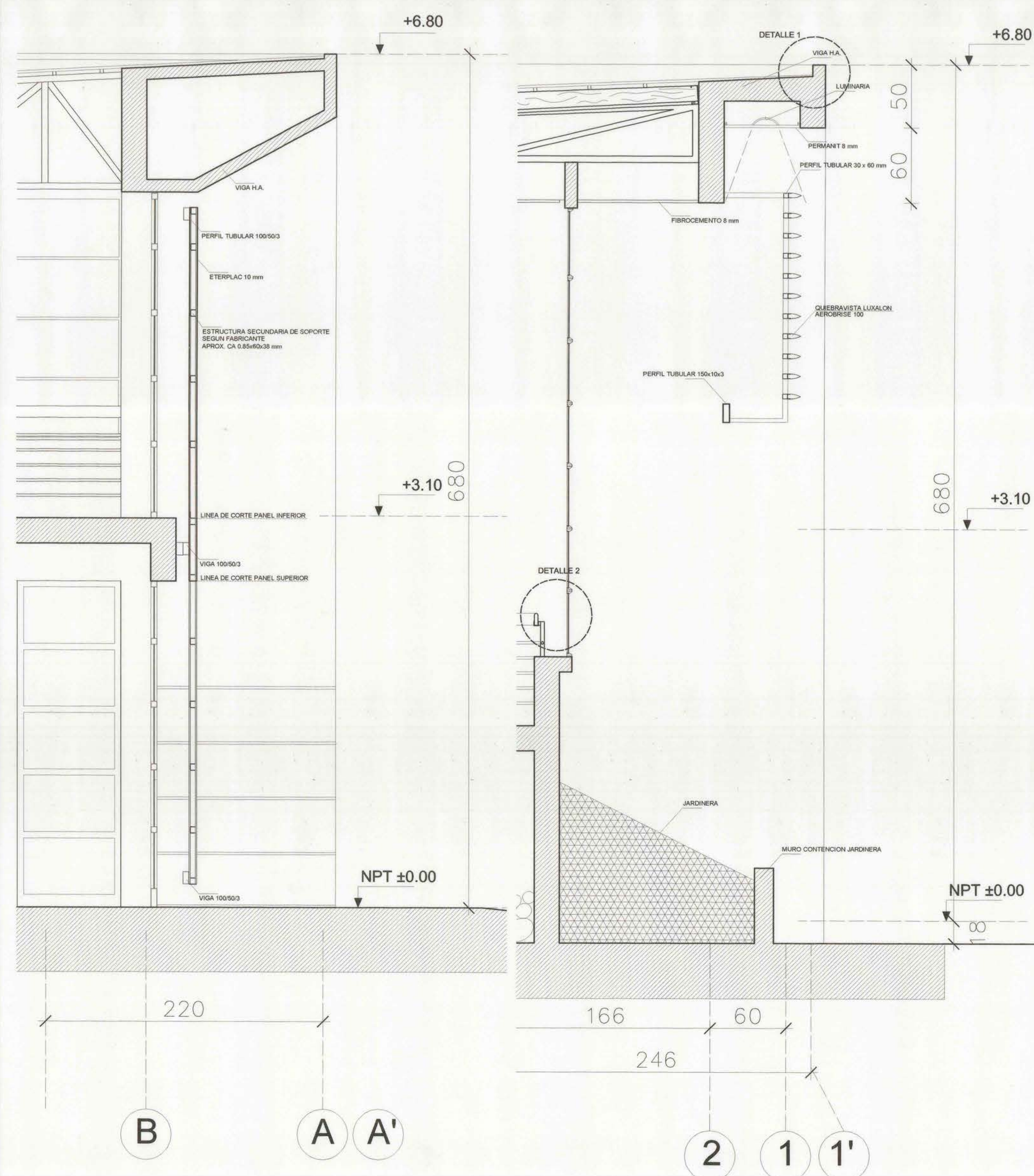
ESCANTILLON FACHADA PRINCIPAL ESC. 1:20
