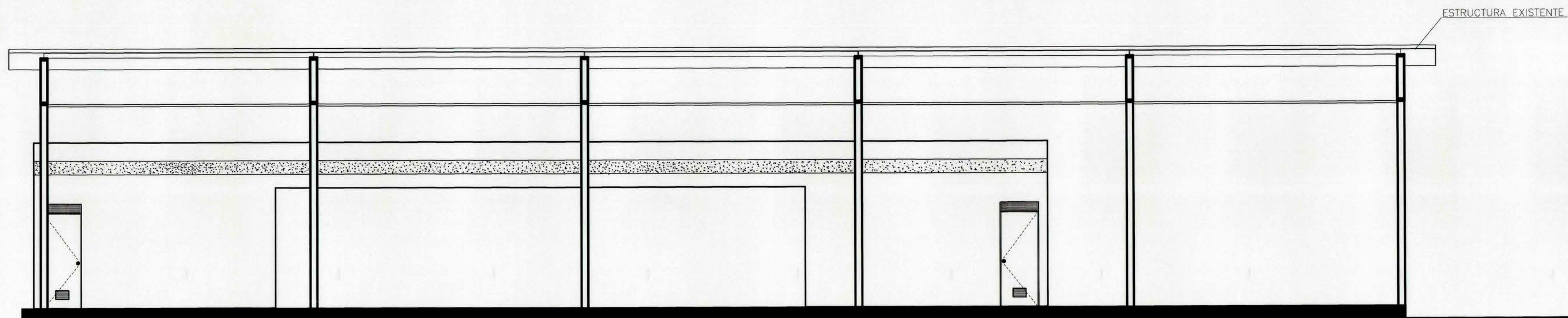
CORTE ELEVACION ORIENTE ESCALA 1 : 50
