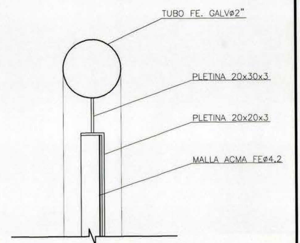
DETALLE R-R ESCALA 1:2
