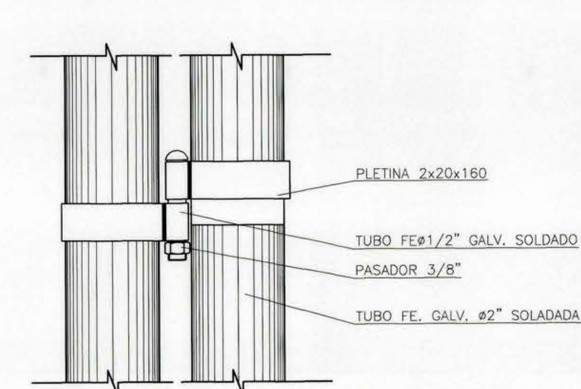
DETALLE Q ESCALA 1:2
