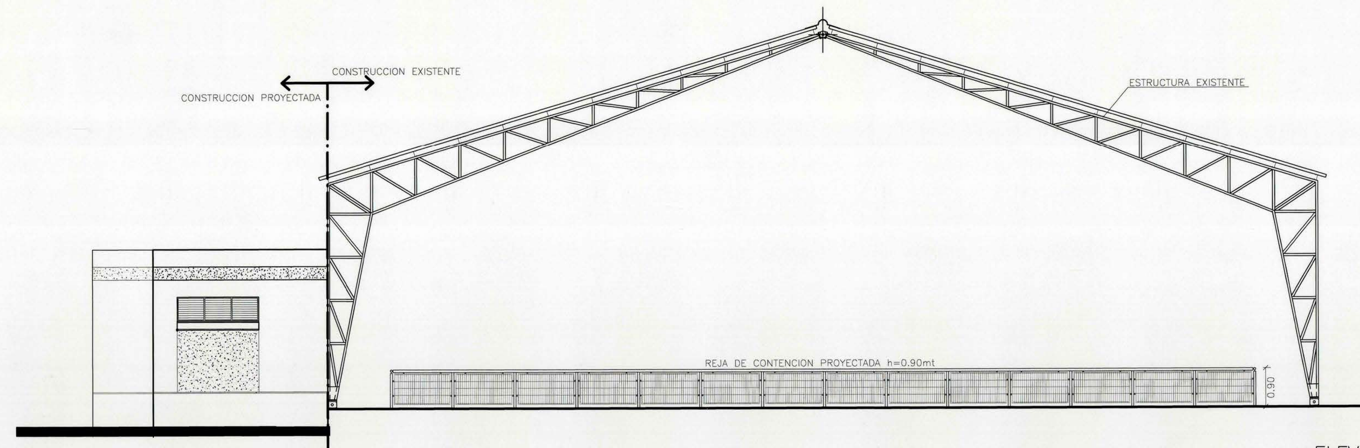
ELEVACION SUR ESCALA 1 : 50
