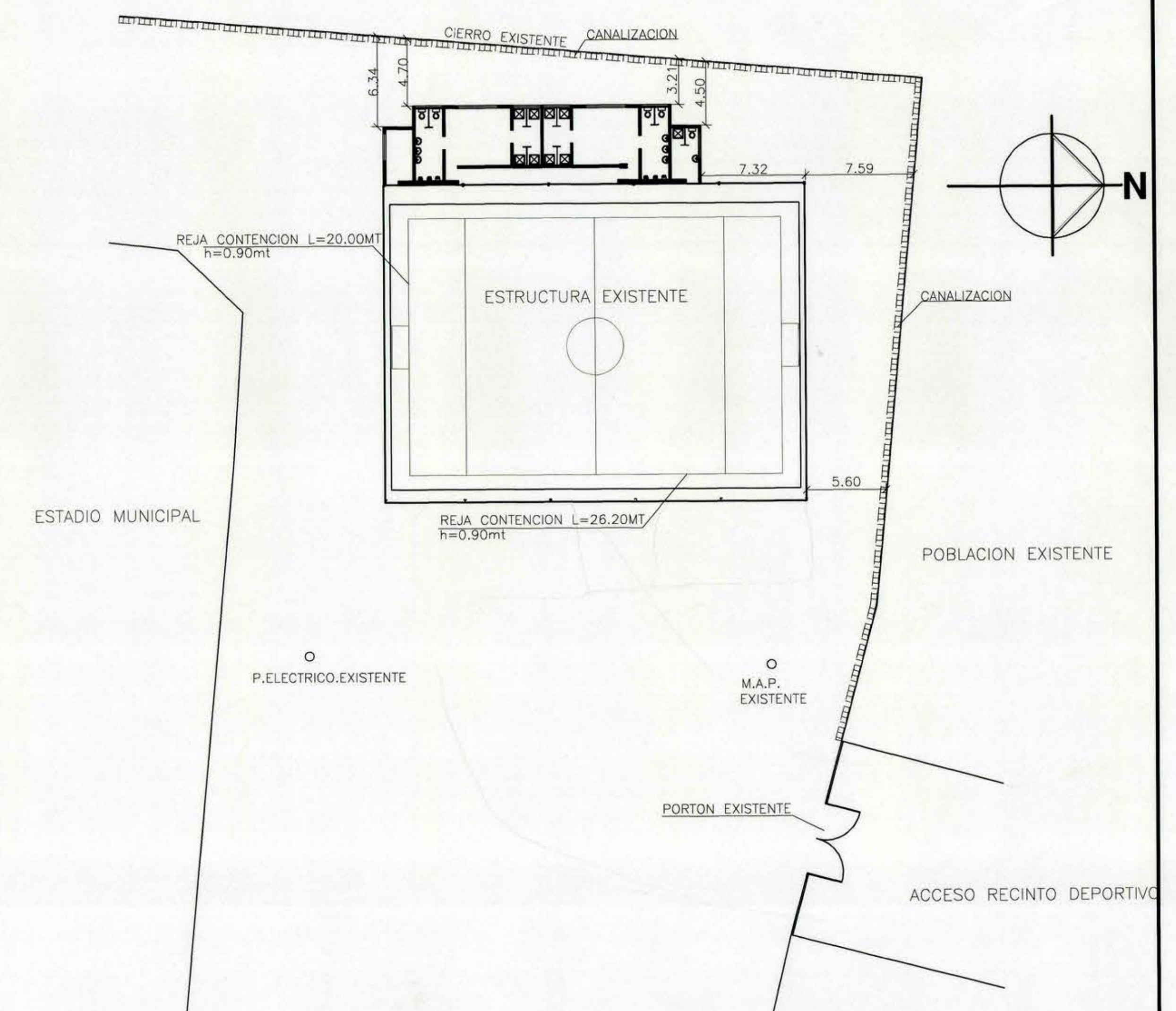
PLANO de EMPLAZAMIENTO ESCALA 1 : 250
