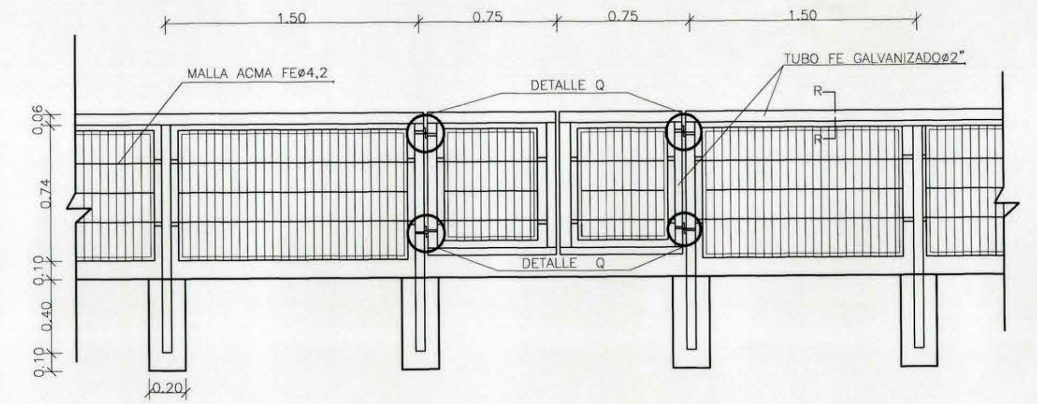
DETALLE REJA DE CONTENCIÓN ESCALA 1 : 20
