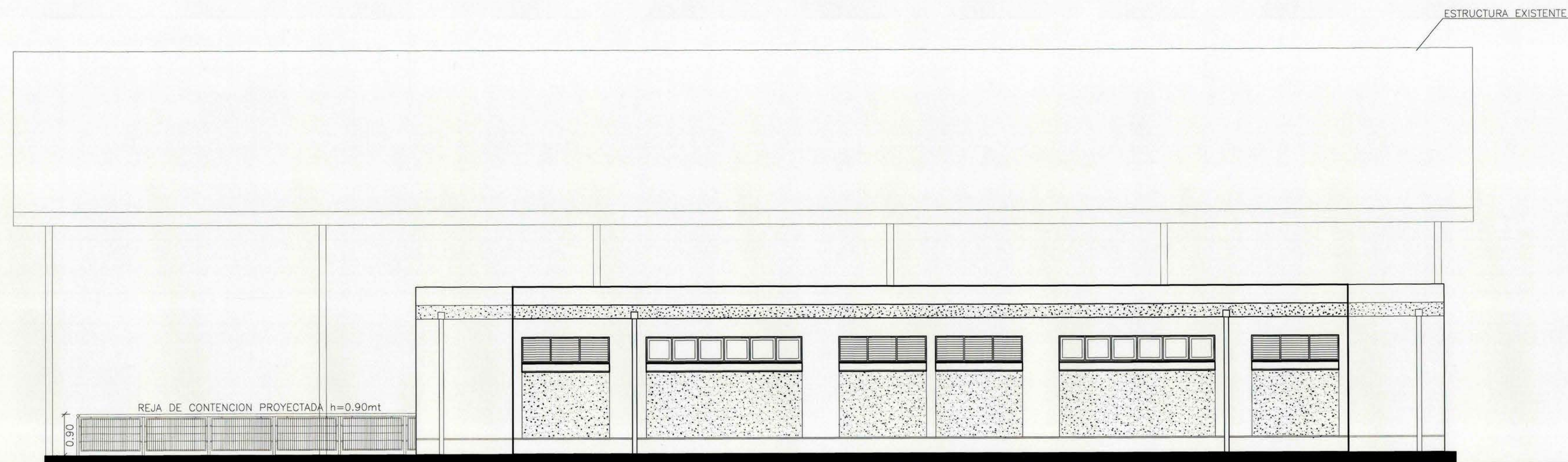
ELEVACION PONIENTE ESCALA 1 : 50
