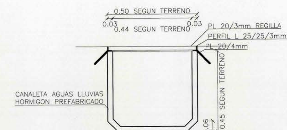
DETALLE CANALIZACION AGUAS LLUVIAS ESCALA 1 : 10
