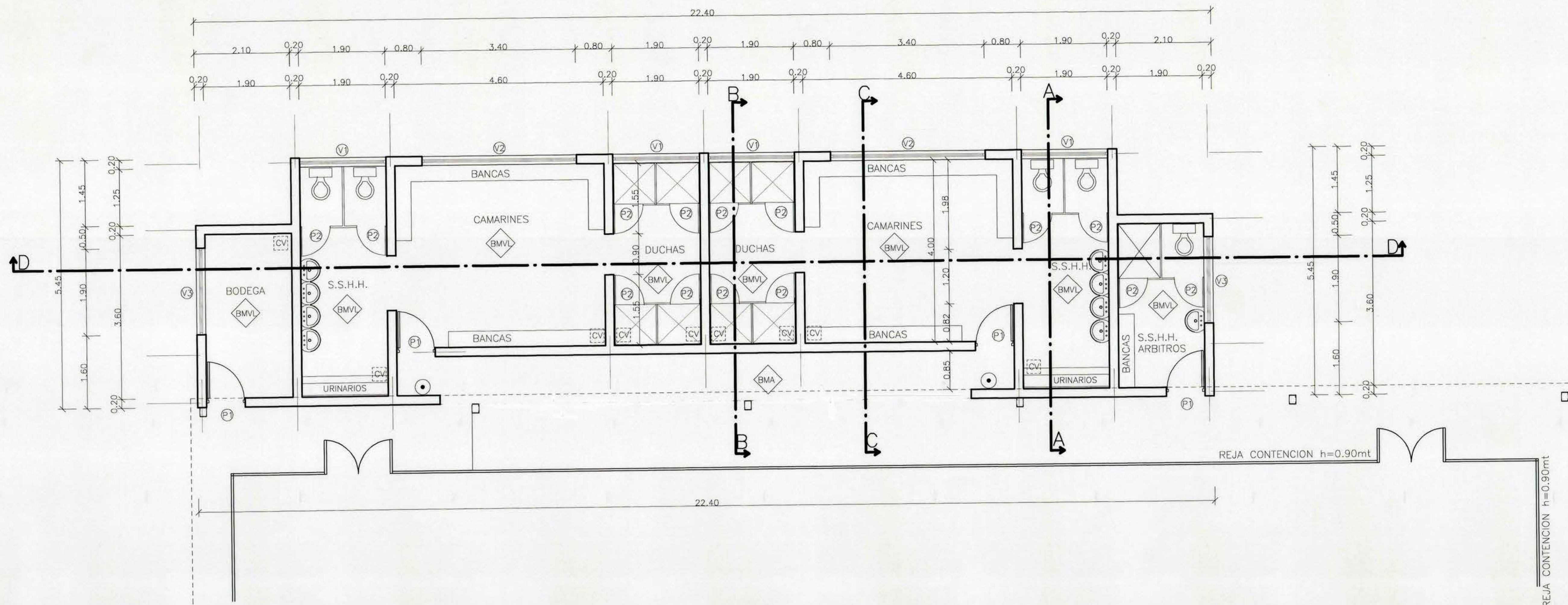
PLANTA GENERAL ESCALA 1 : 50
