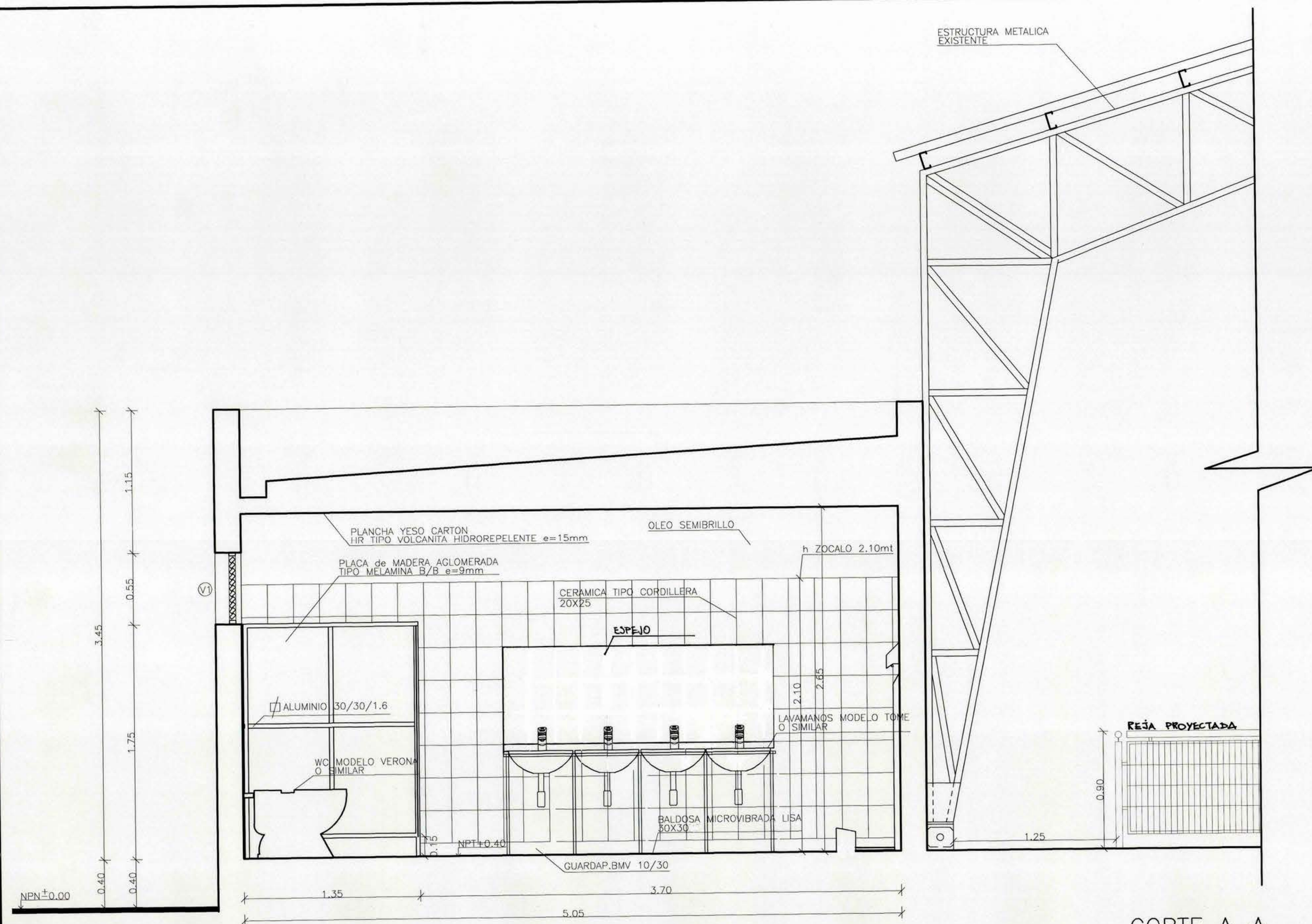
CORTE A-A ESCALA 1 : 20
