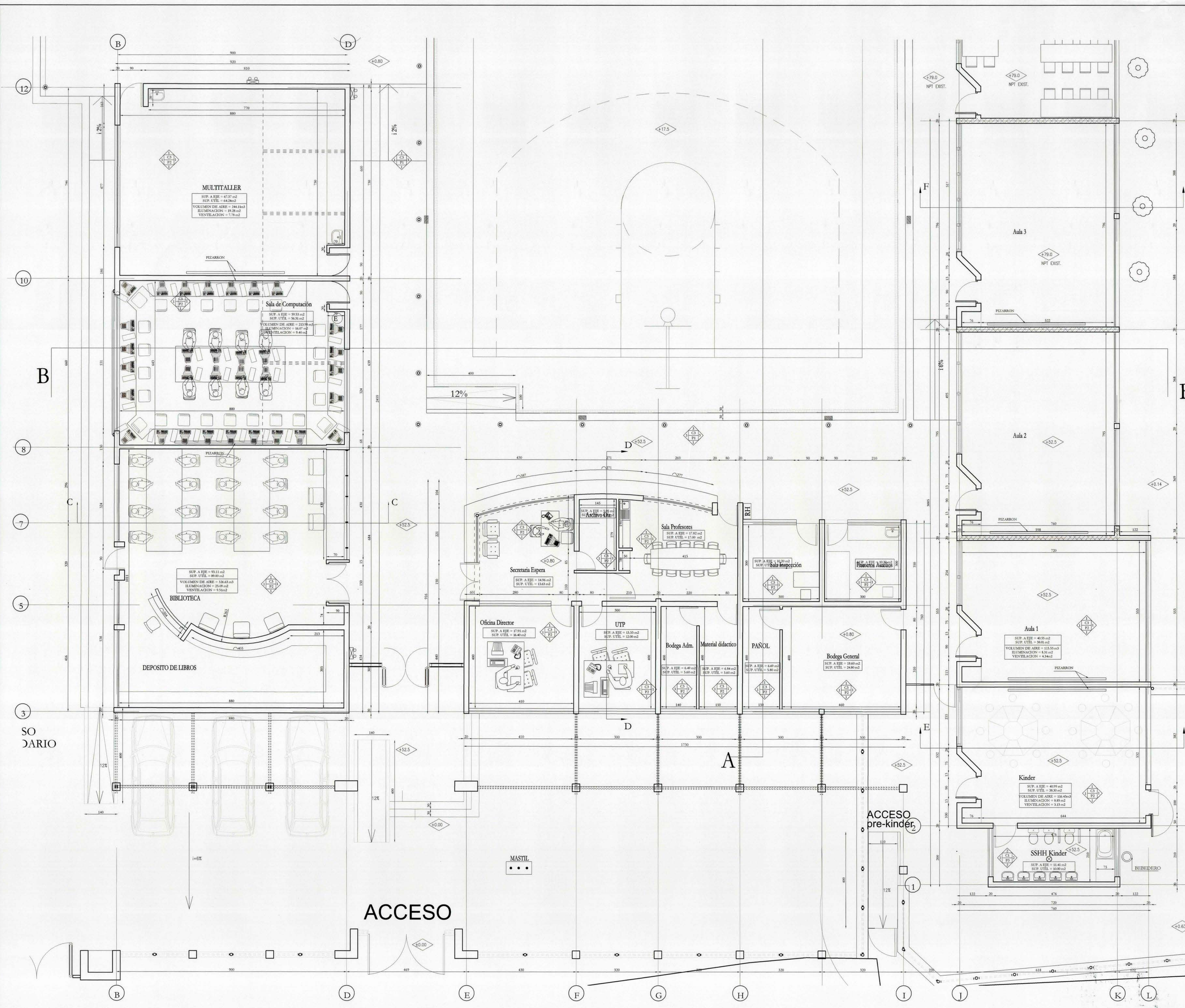
PLANTA GENERAL Esc. 1/50
