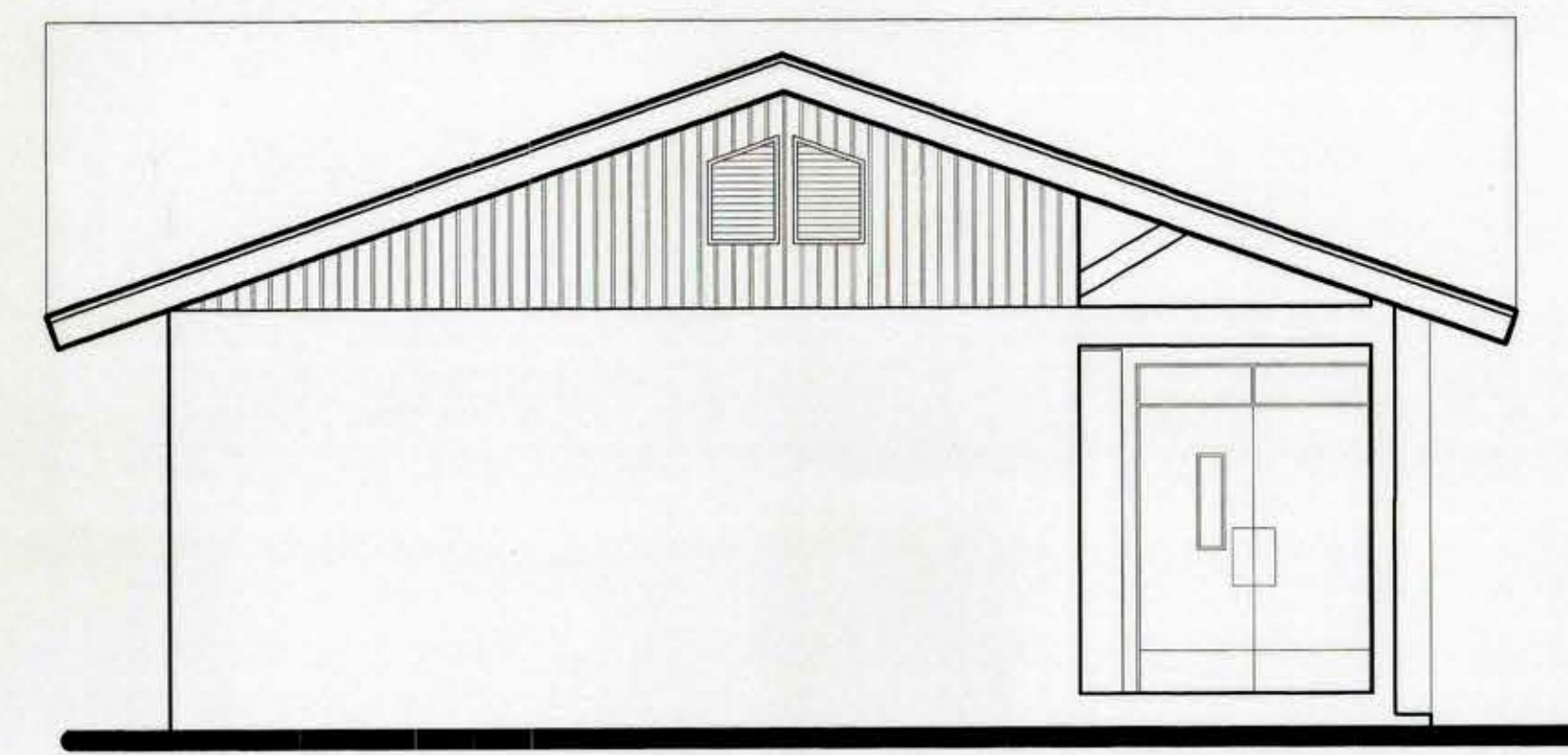
ELEVACION NOR-ORIENTE ESCALA 1:50
