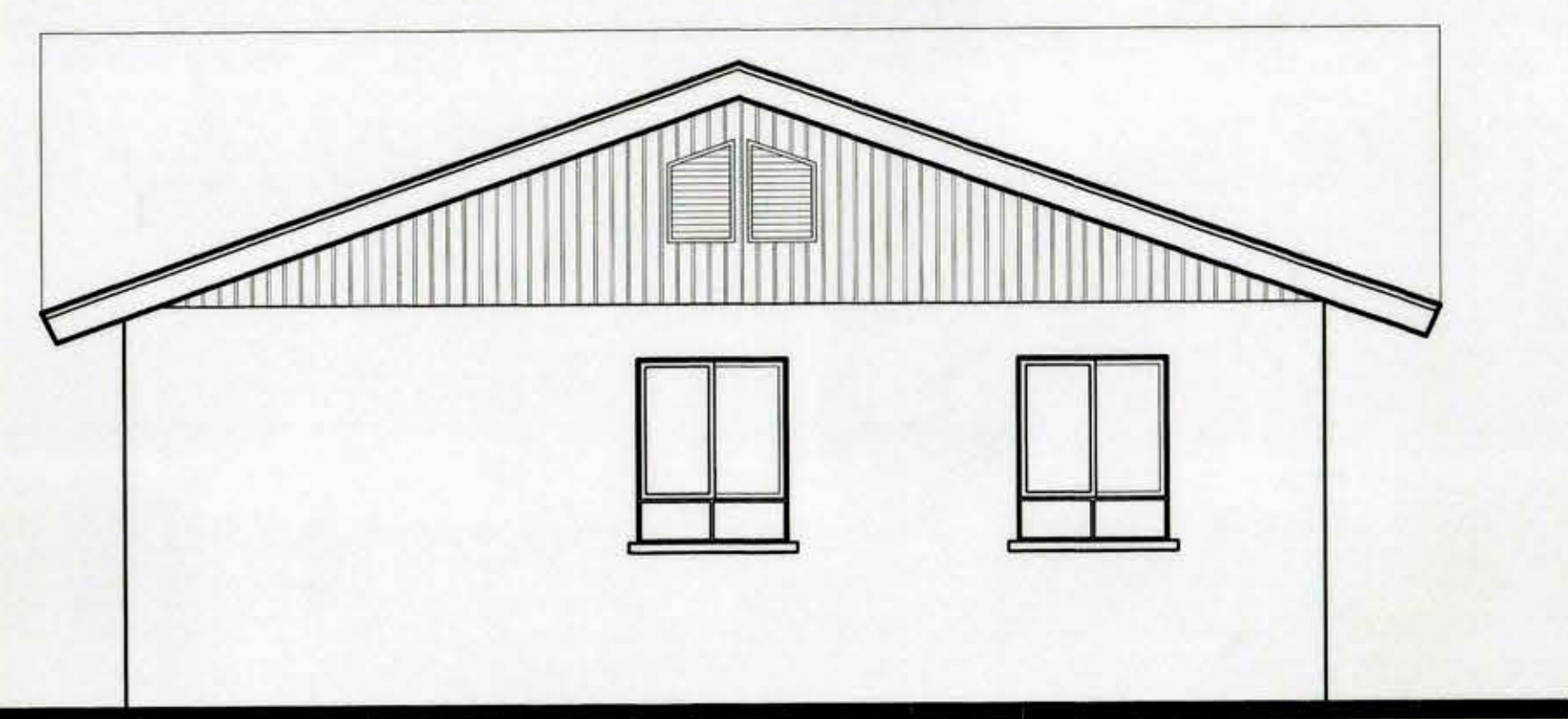
ELEVACION SUR-PONIENTE ESCALA 1:50
