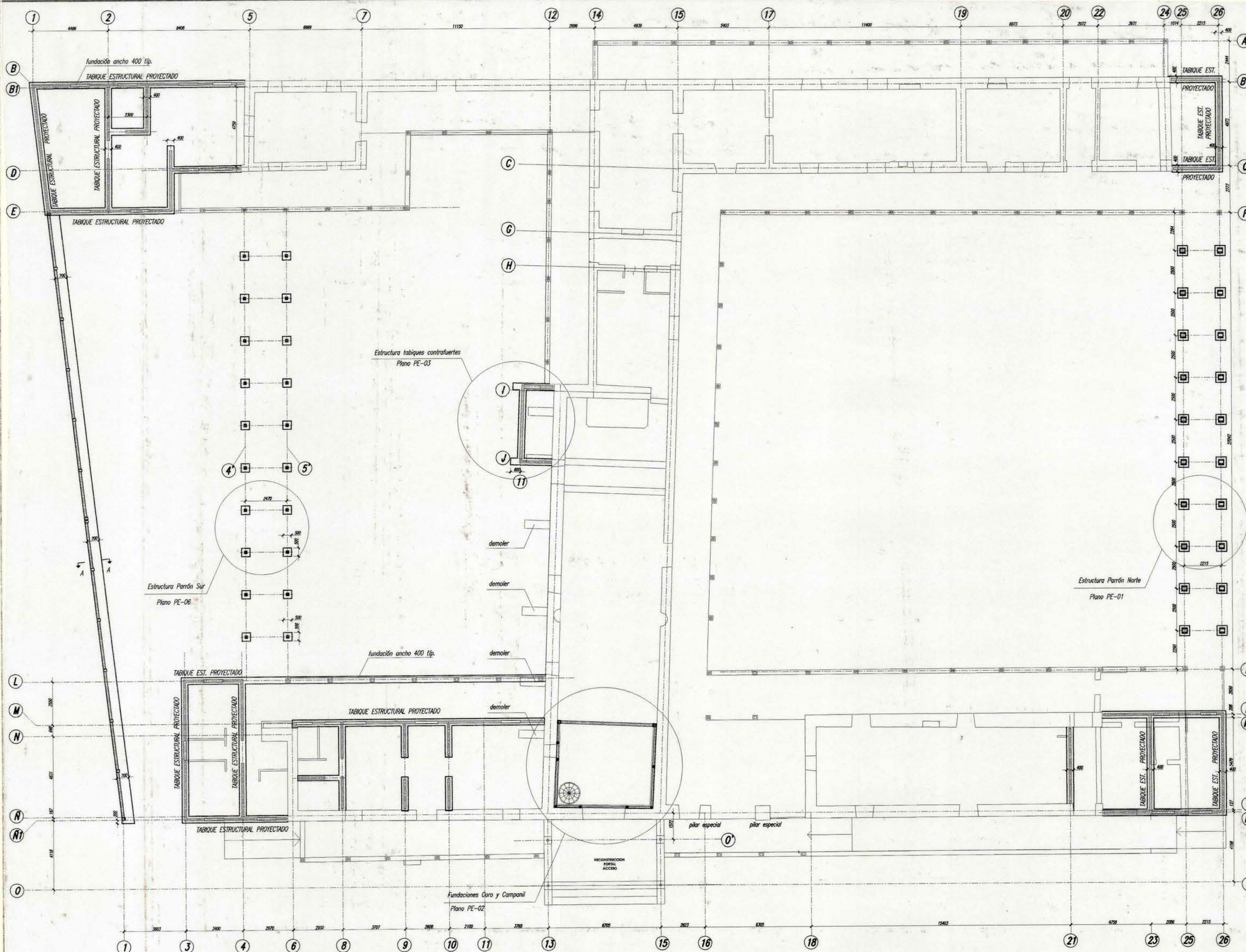
PLANTA GENERAL DE FUNDACIONES ESC.=1:100
