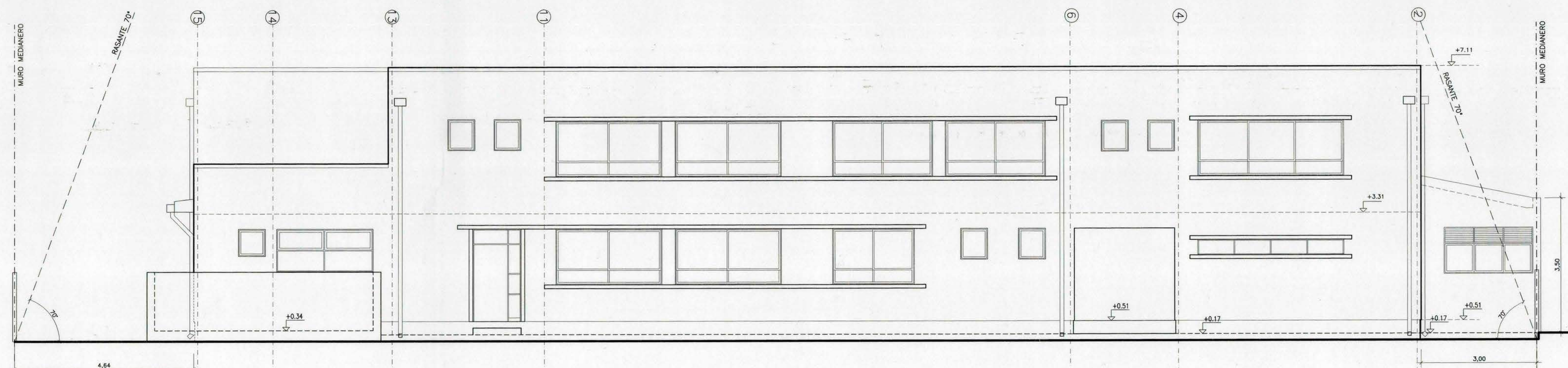
ELEVACION SUR ESCALA 1:50
