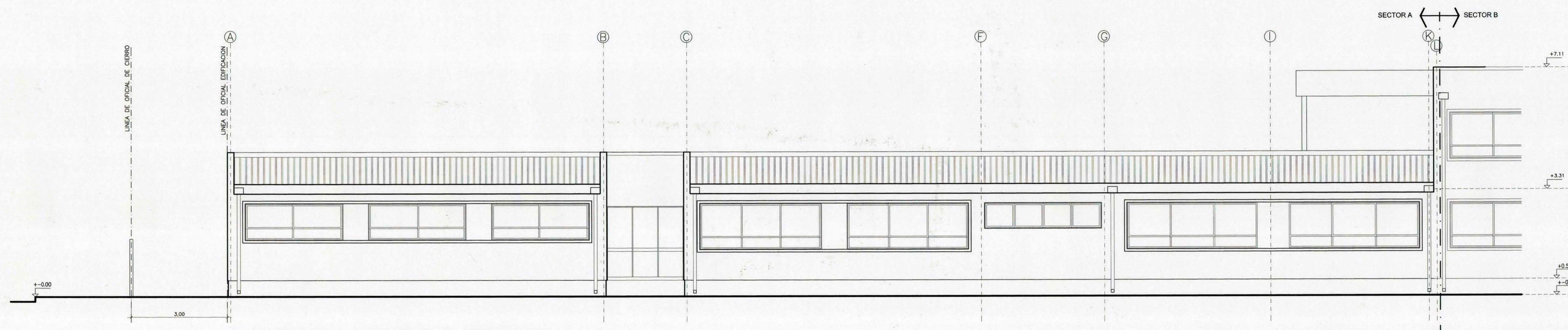
ELEVACION PONIENTE SECTOR A ESCALA 1:50
