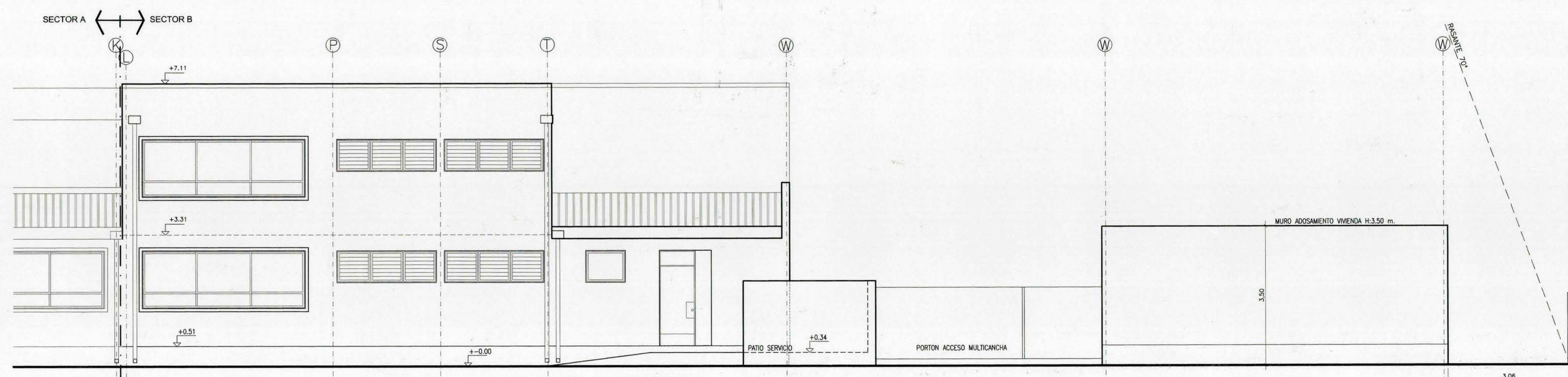
ELEVACION PONIENTE SECTOR B ESCALA 1:50
