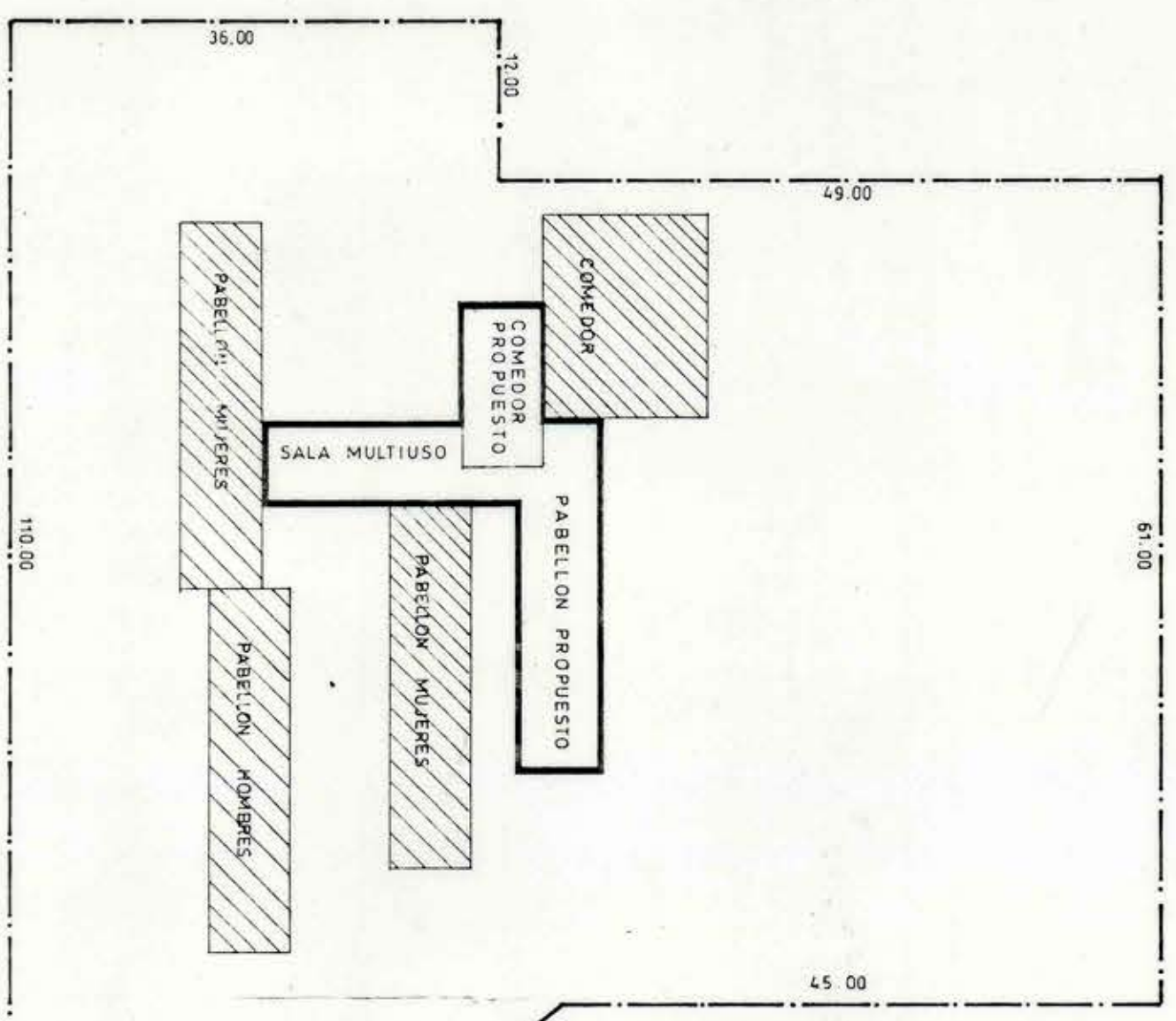
PLANO EMPLAZAMIENTO ESC. 1:500
