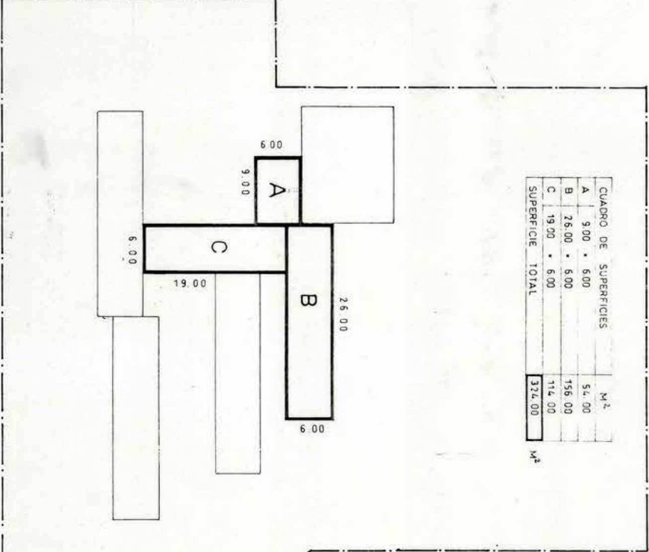
CALCULO SUPERFICIES
