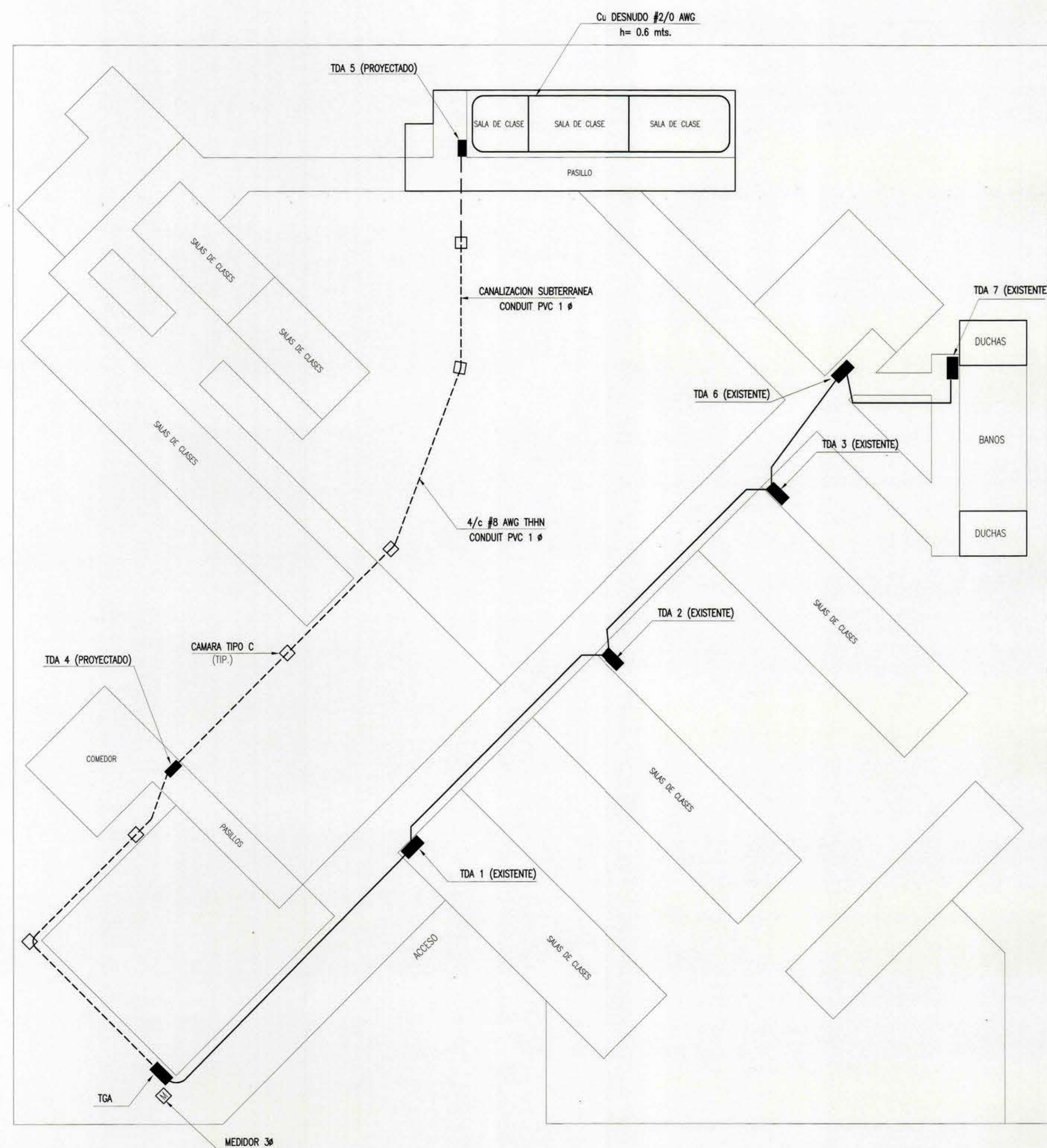
PLANO DE EMPLAZAMIENTO Esc. 1: 250
