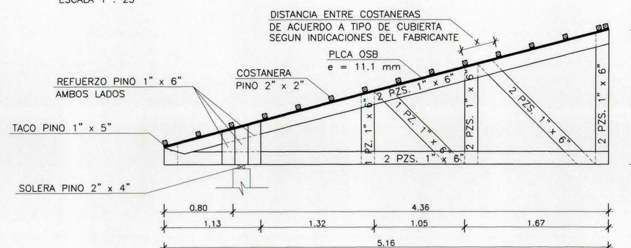
CERCHA TIPO C-7 ESCALA 1 : 25
