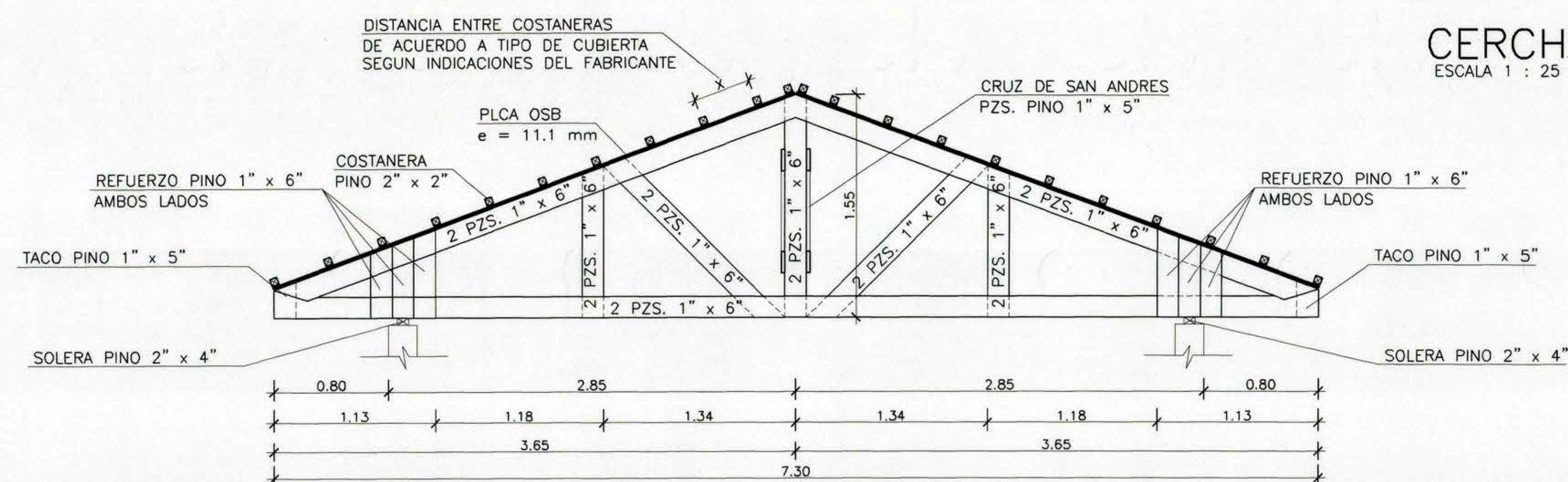
CERCHA TIPO C-7 ESCALA 1 : 25
