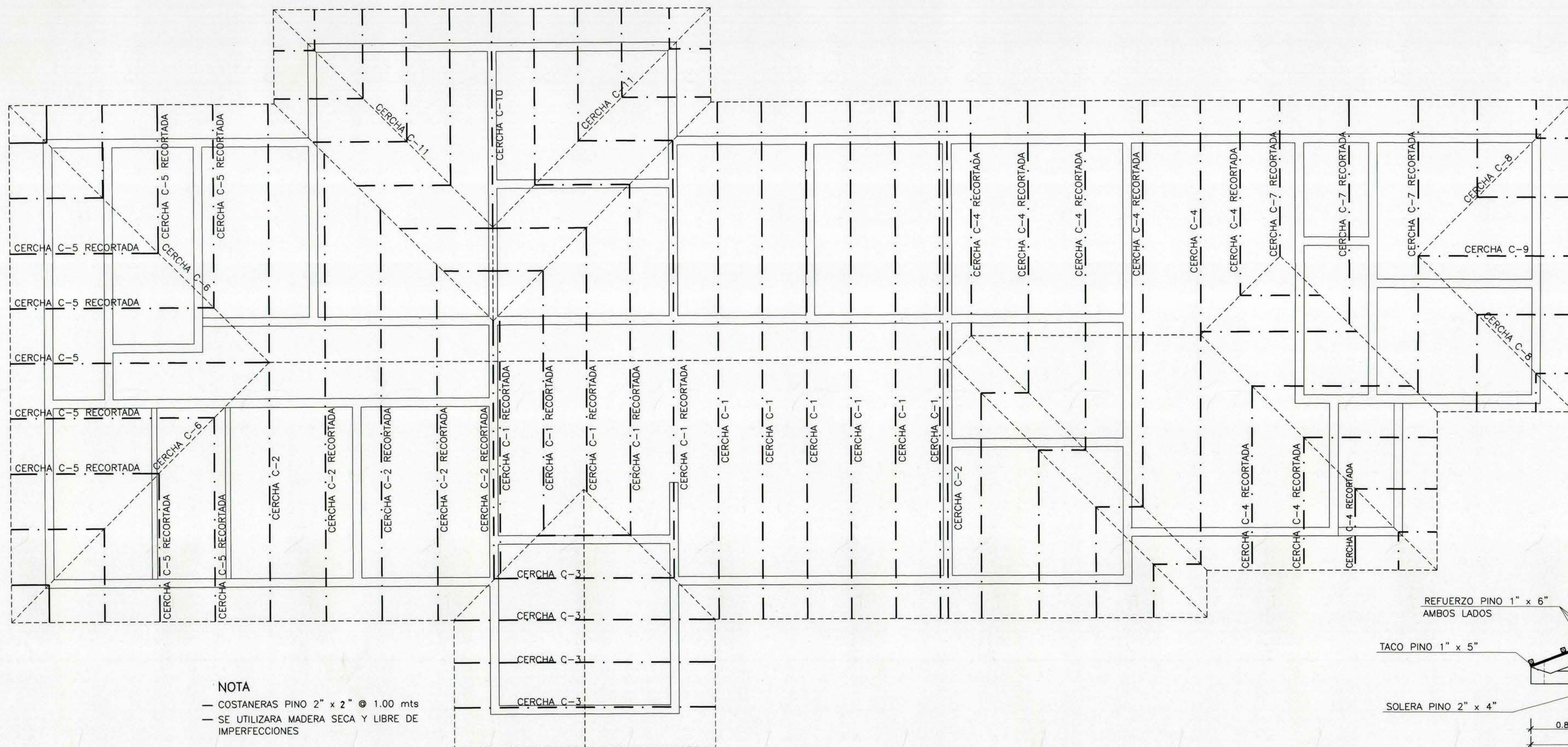
PLANTA DE ESTRUCTURA DE TECHUMBRE ESCALA 1 : 50
