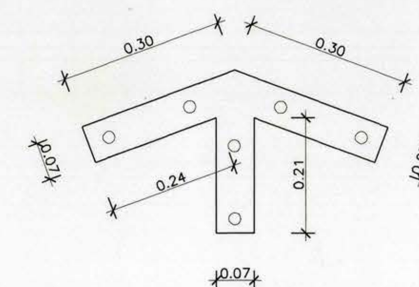
DETALLE N° 2 ESCALA 1 : 7.5
