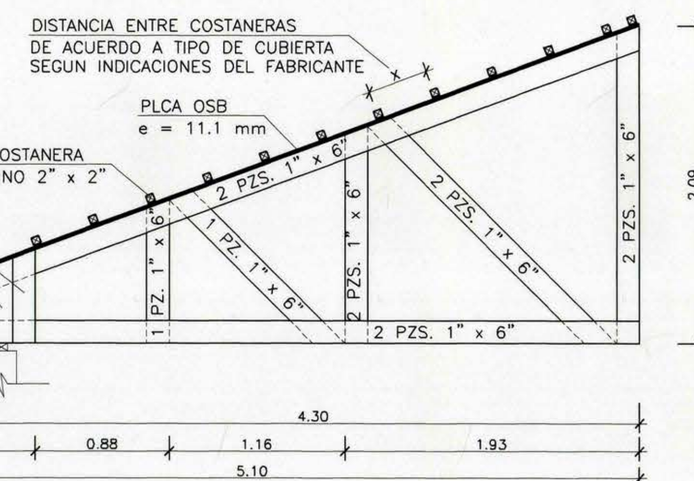
CERCHA TIPO C-10 ESCALA 1 : 25
