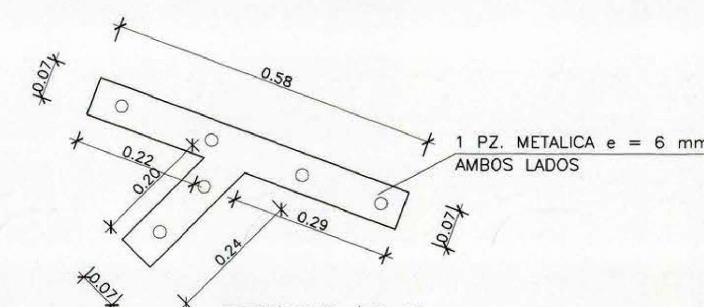
DETALLE N° 3 ESCALA 1 : 7.5
