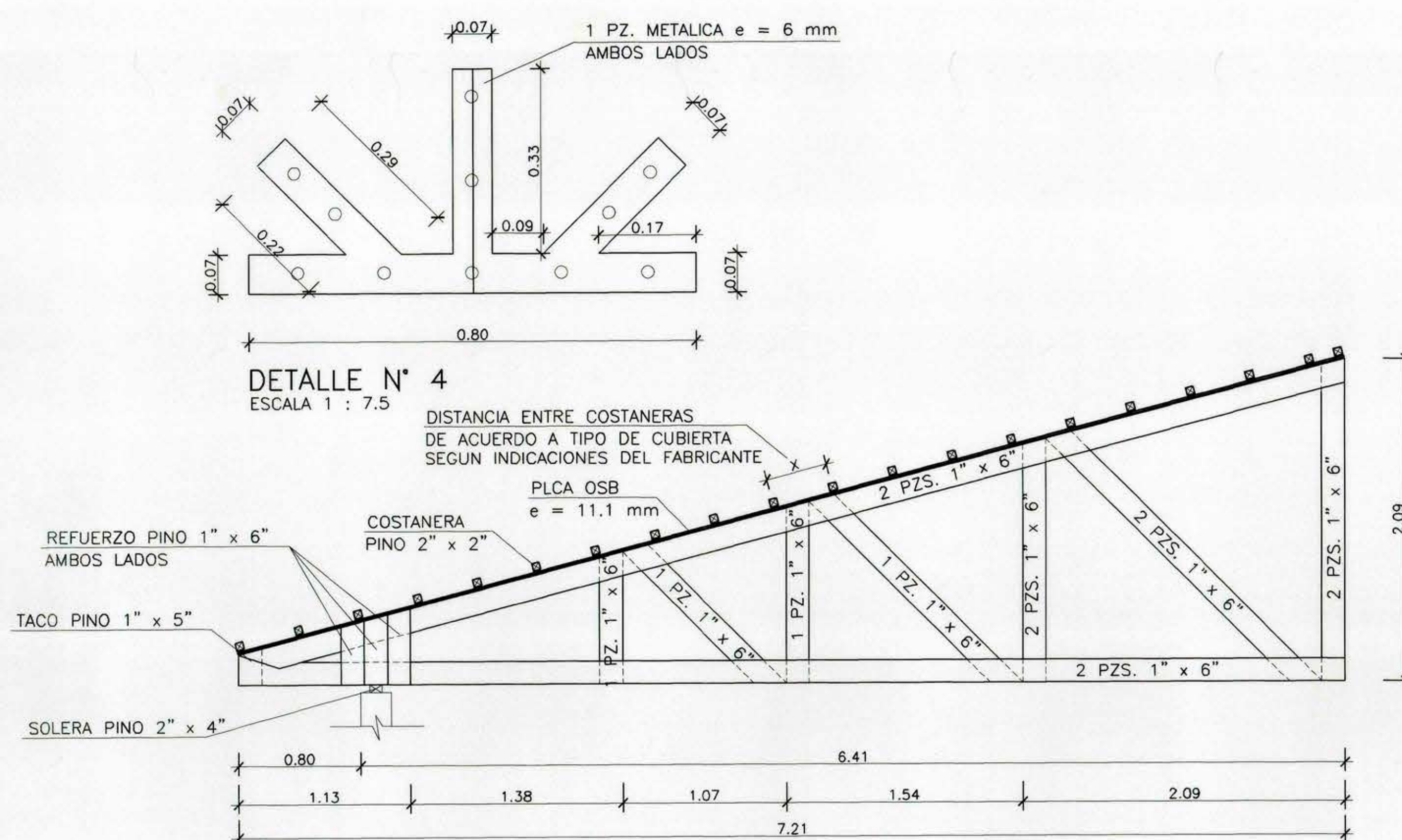
CERCHA TIPO C-11 ESCALA 1 : 25
