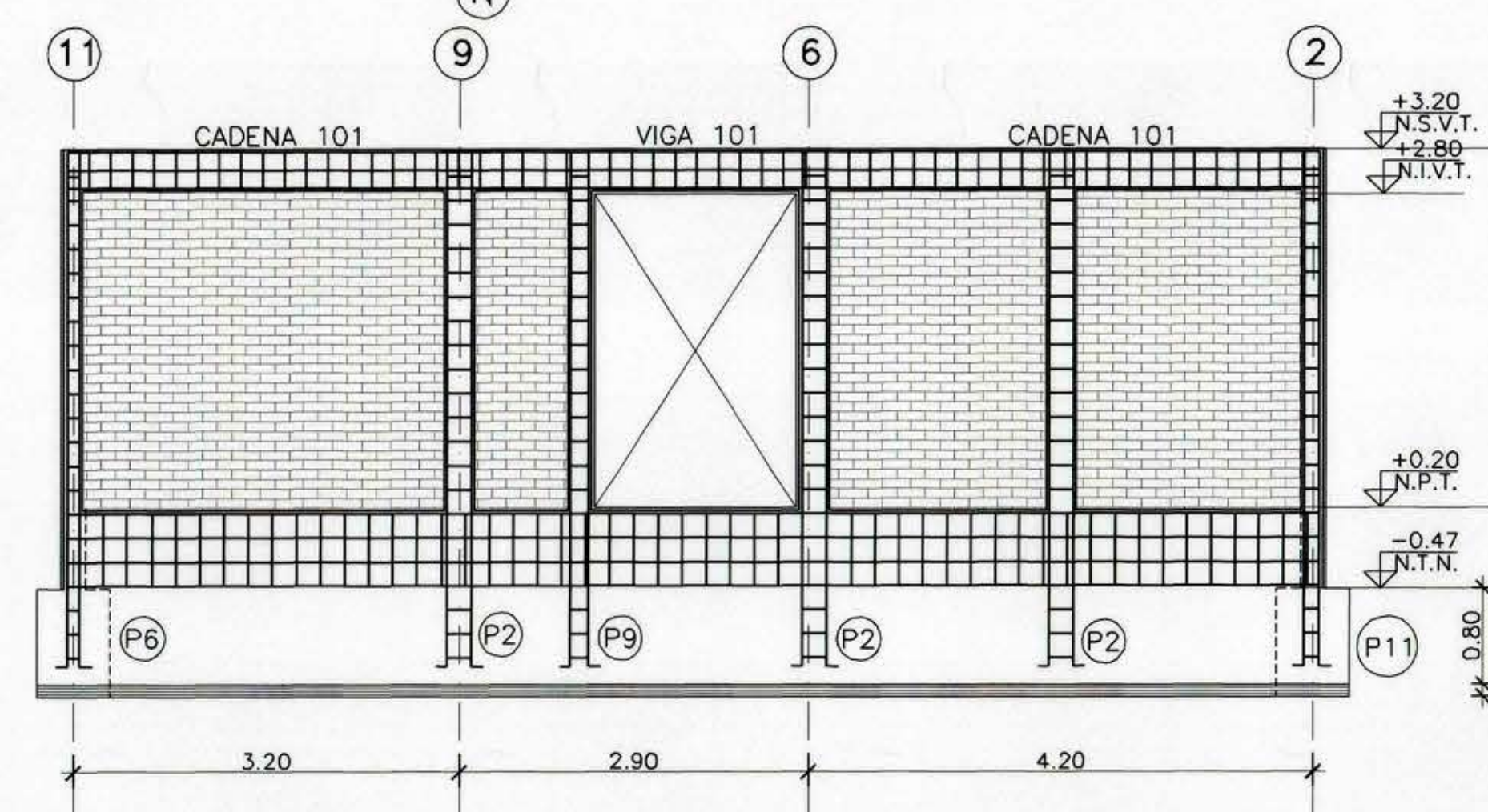
ELEVACION EJE I ESCALA 1:50
