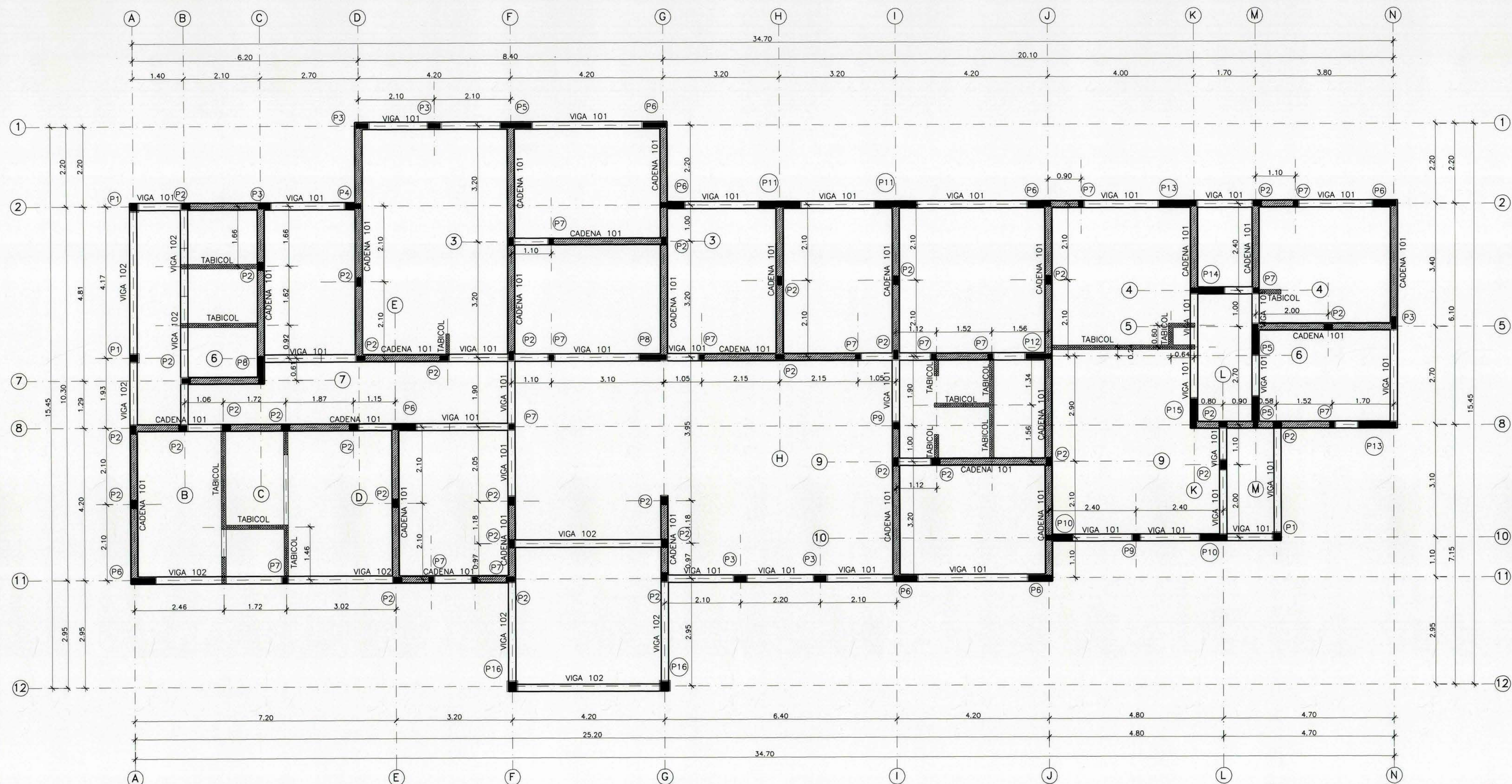
PLANTA DE ESTRUCTURAS ESCALA 1 : 50
