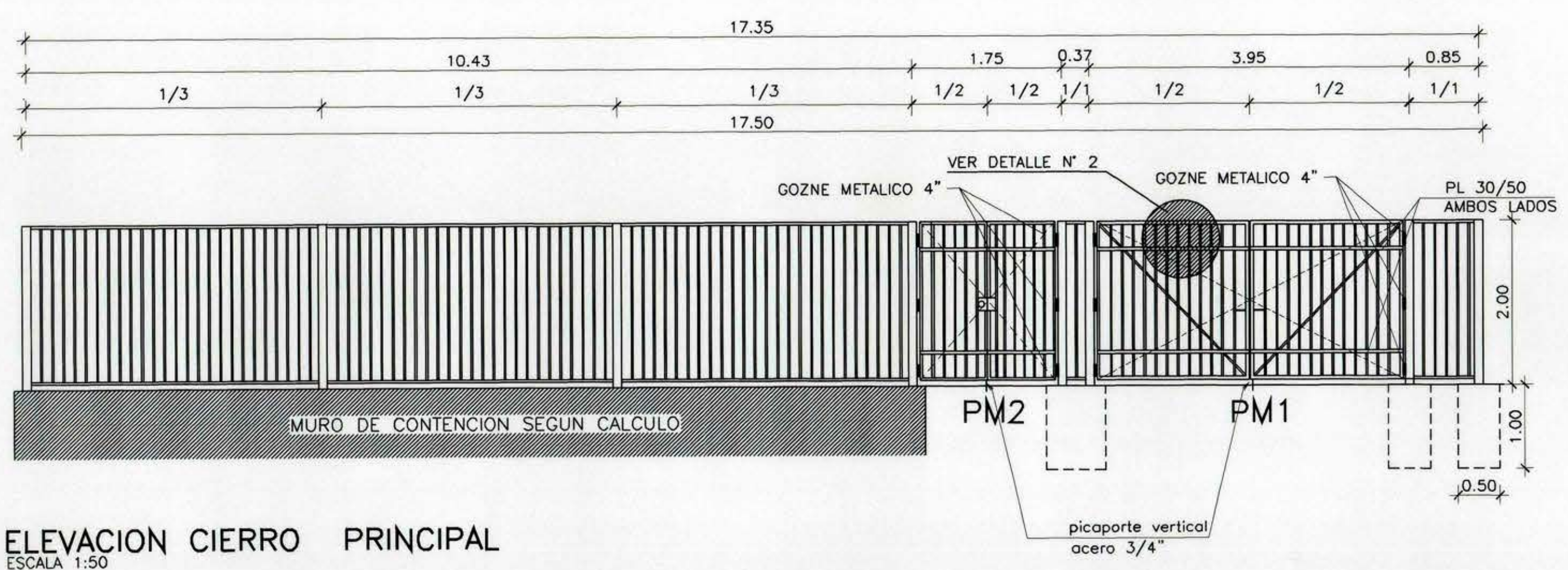
PAÑO TIPICO REJA METALICA ESCALA 1:50
