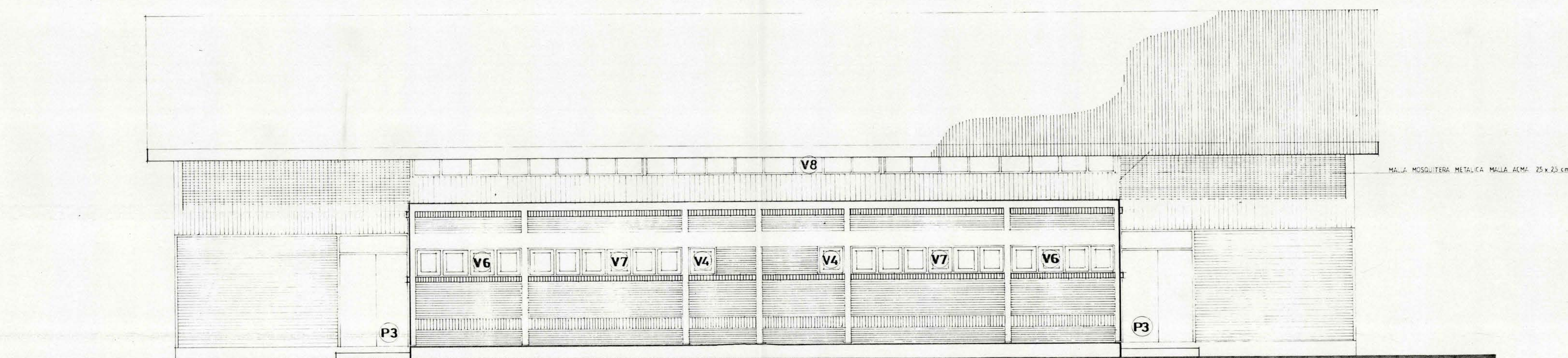
ELEVACION SUR
