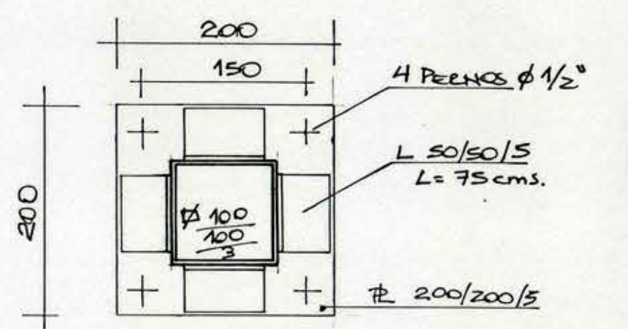
DETALLE 2 ESC. 1:5
