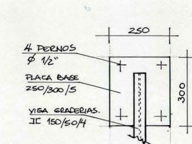
DETALLE 1 ESC. 1:10
