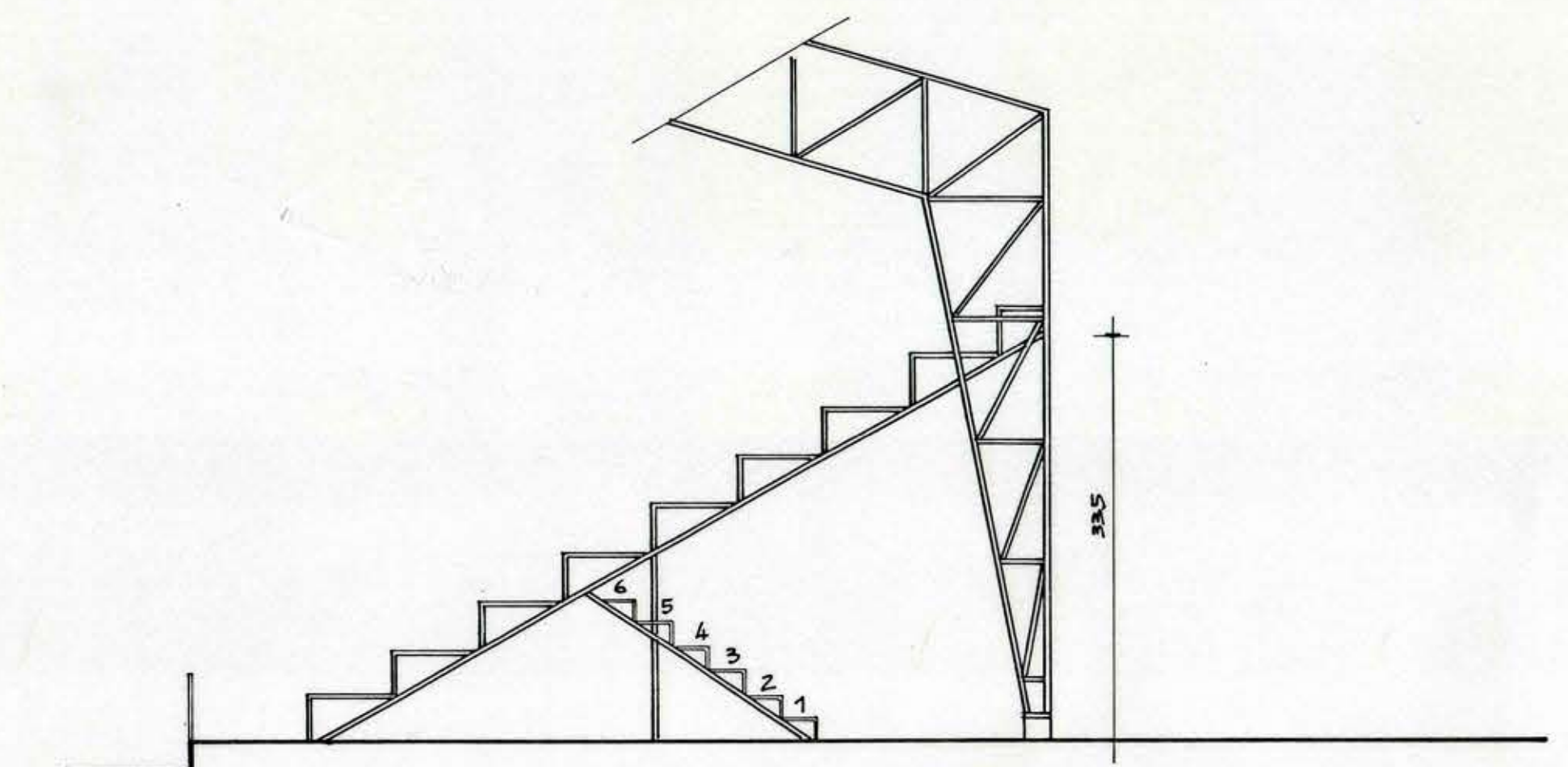
CORTE ESQUEMATICO
