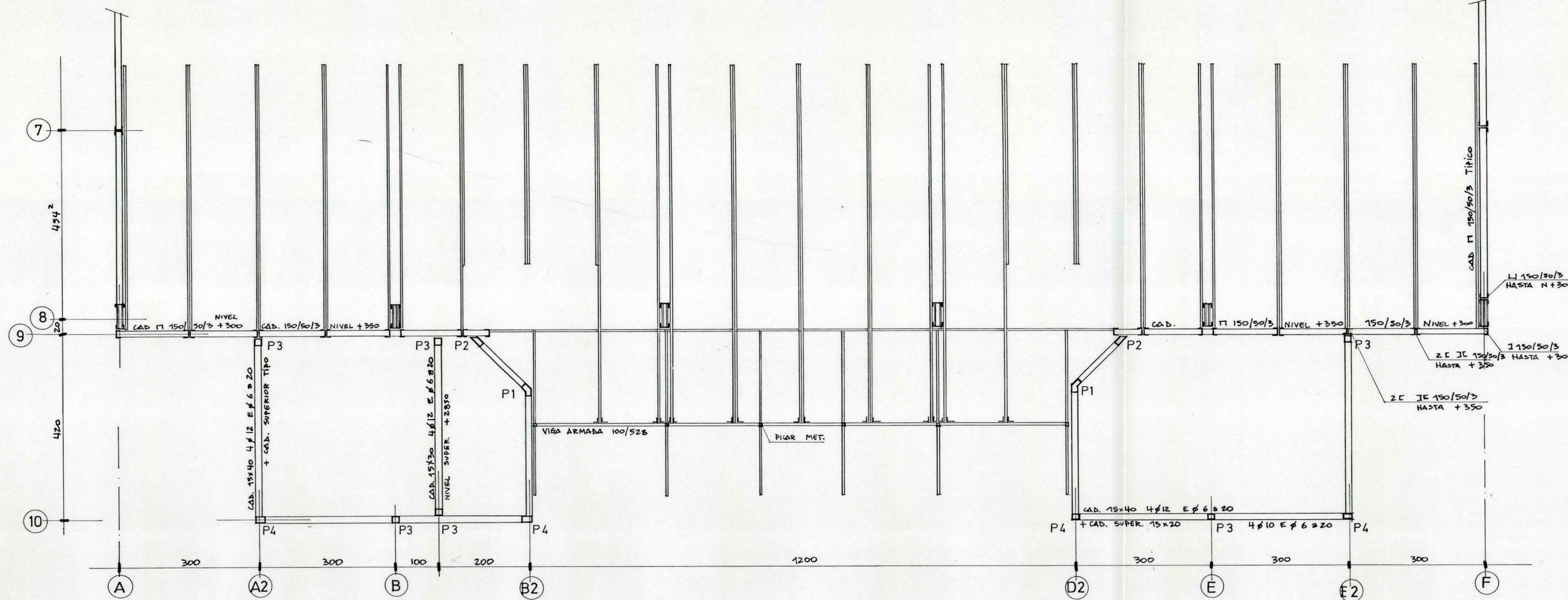
PLANTA ESTRUCTURA ESCALA 1/50
