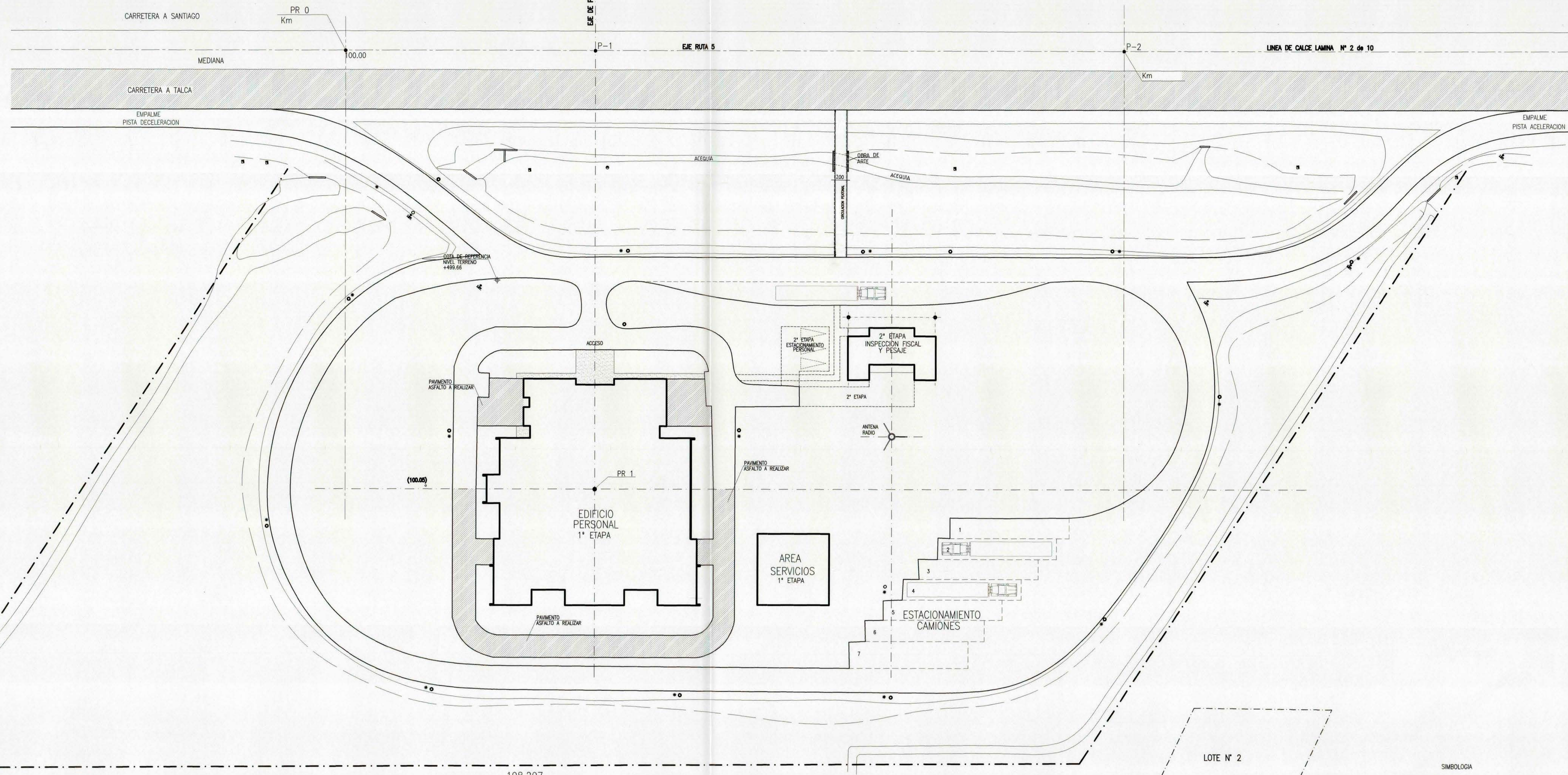
PLANTA GENERAL LOTE N° 1 ESC. 1/250 (REFERENCIAL PARA EMPLAZAMIENTO)
