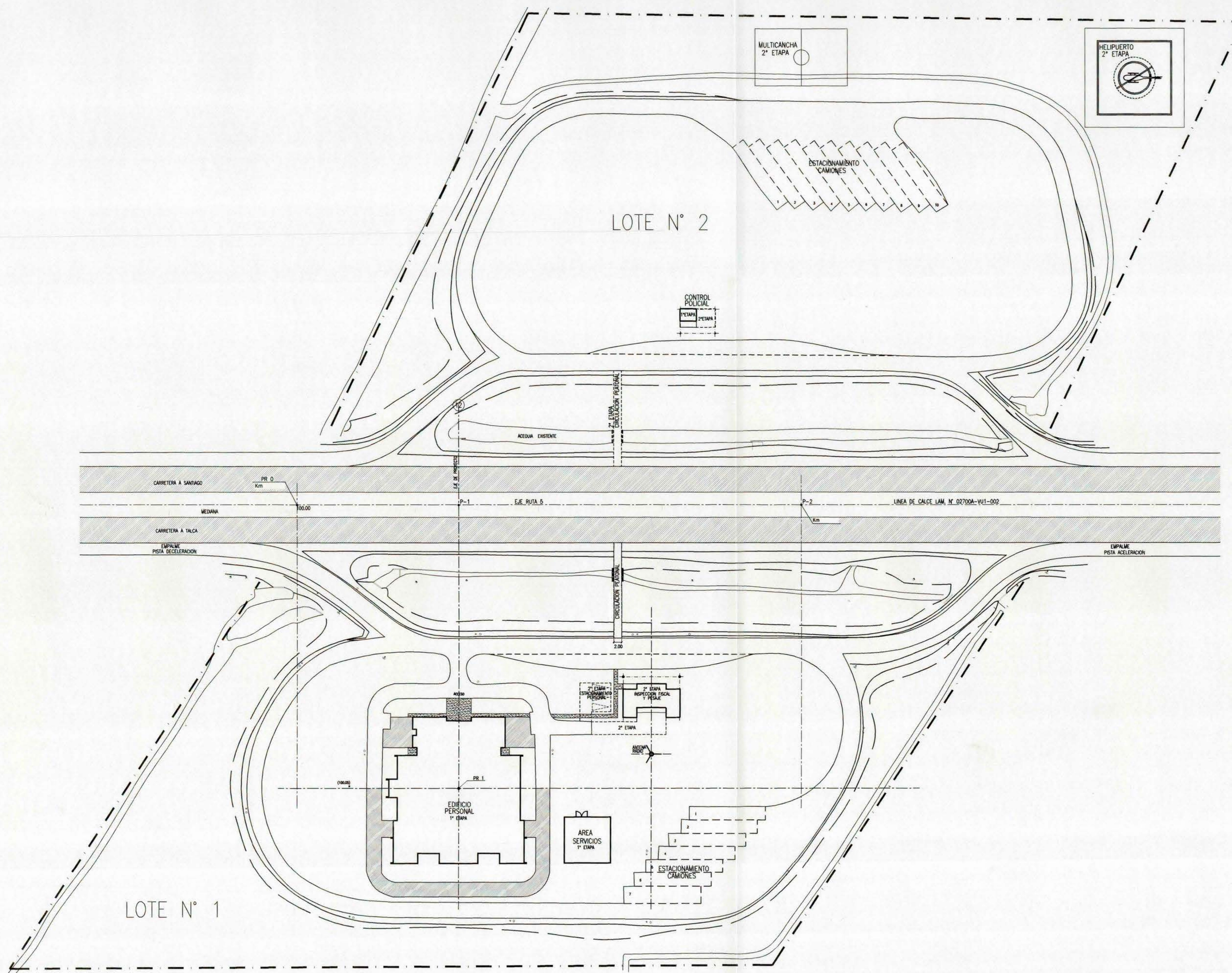
PLANTA EMPLAZAMIENTO GENERAL LOTES N° 1 Y N°2 ESC. 1/250 (REFERENCIAL PARA EMPLAZAMIENTO)
