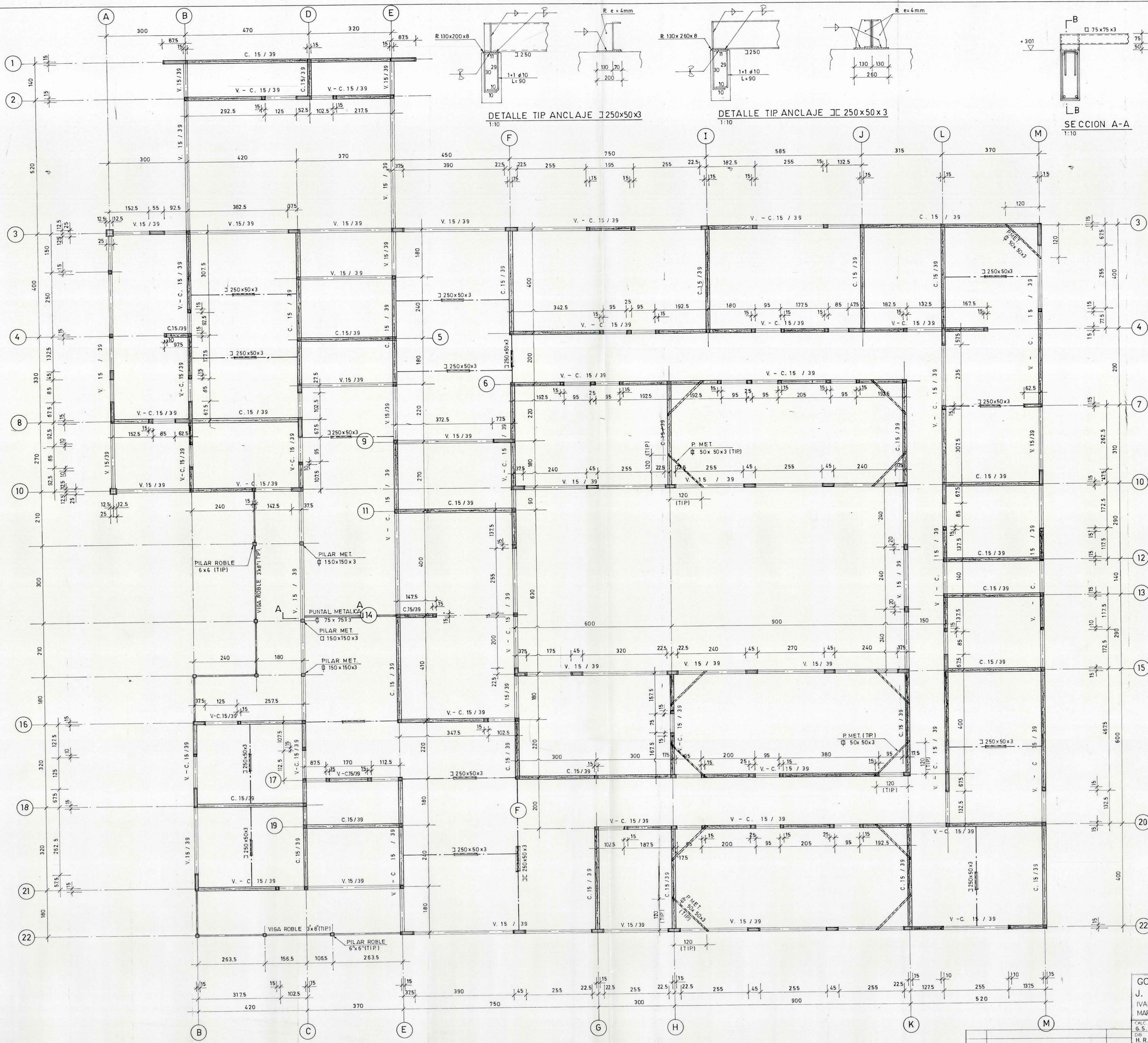
PLANTA DE ESTRUCTURA CIELO 1° PISO 1:50 ELEV. SUP. VIGAS Y CADENAS +301
