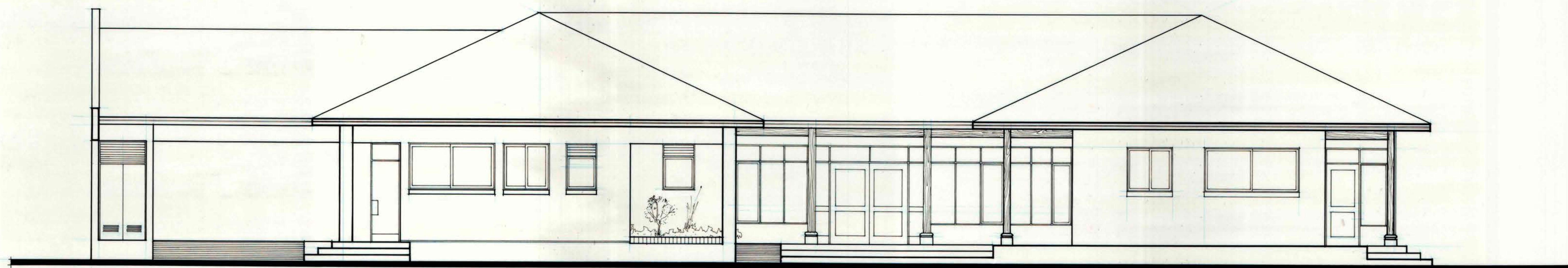
ELEVACION PONIENTE
