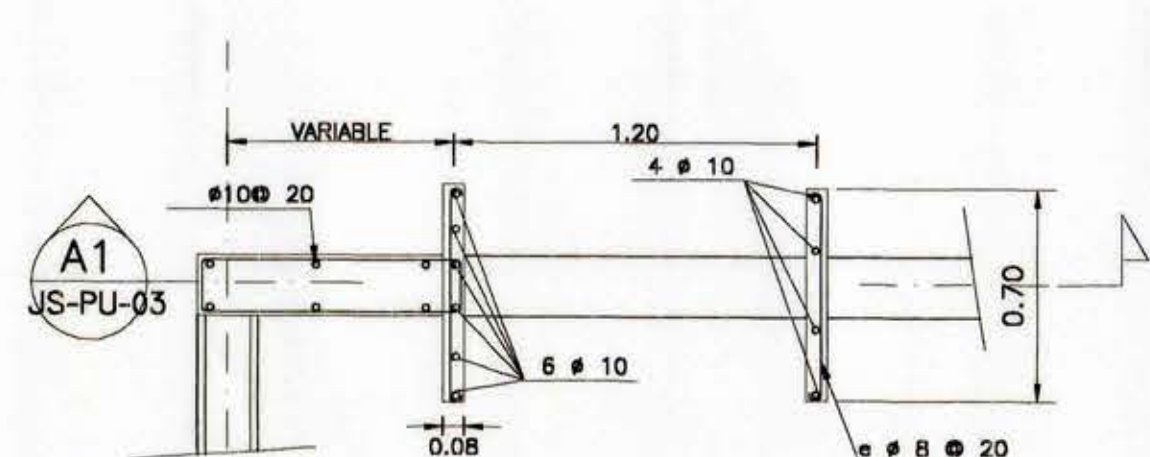
DETALLE A escala 1/25
