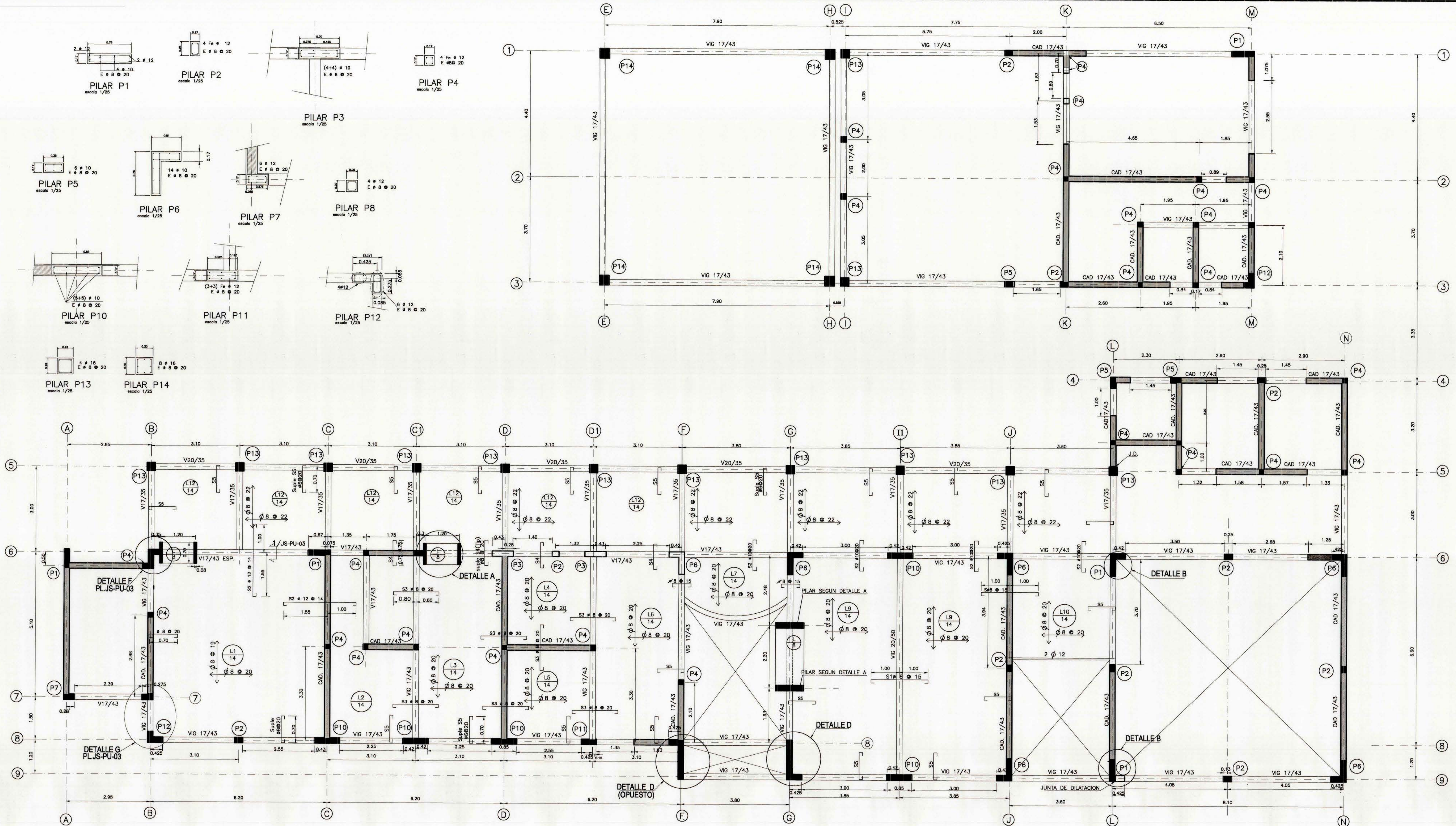
PLANTA DE ESTRUCTURAS 1º PISO ESCALA 1 : 50
