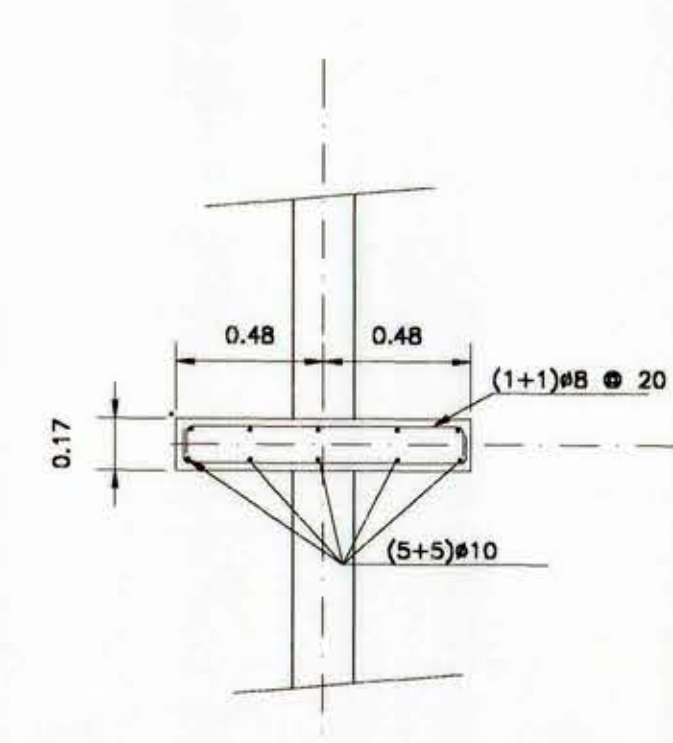
DETALLE C escala 1/25
