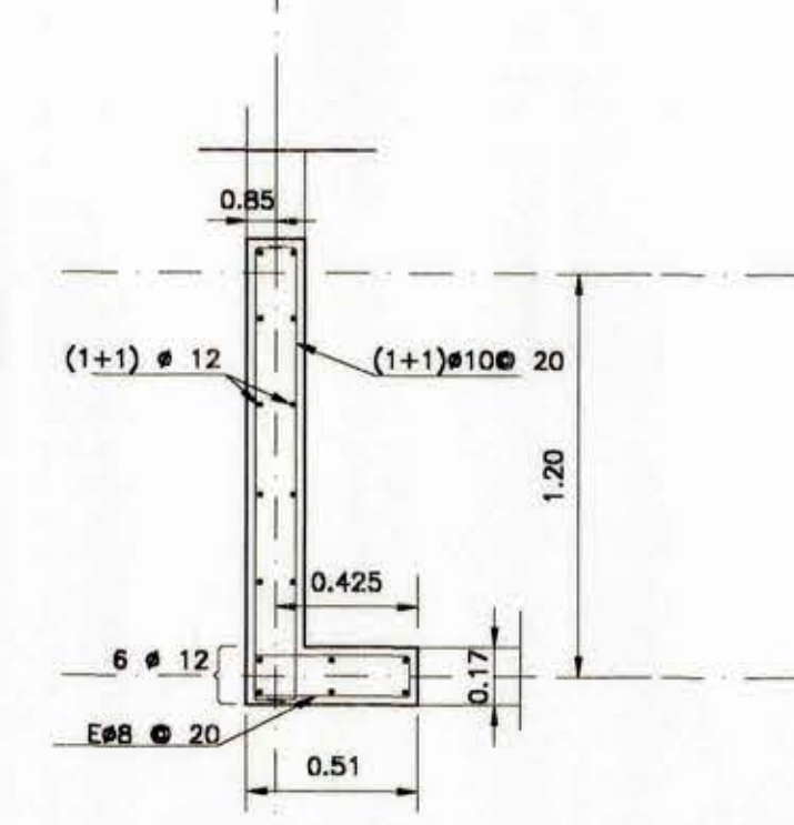
DETALLE D escala 1/25
