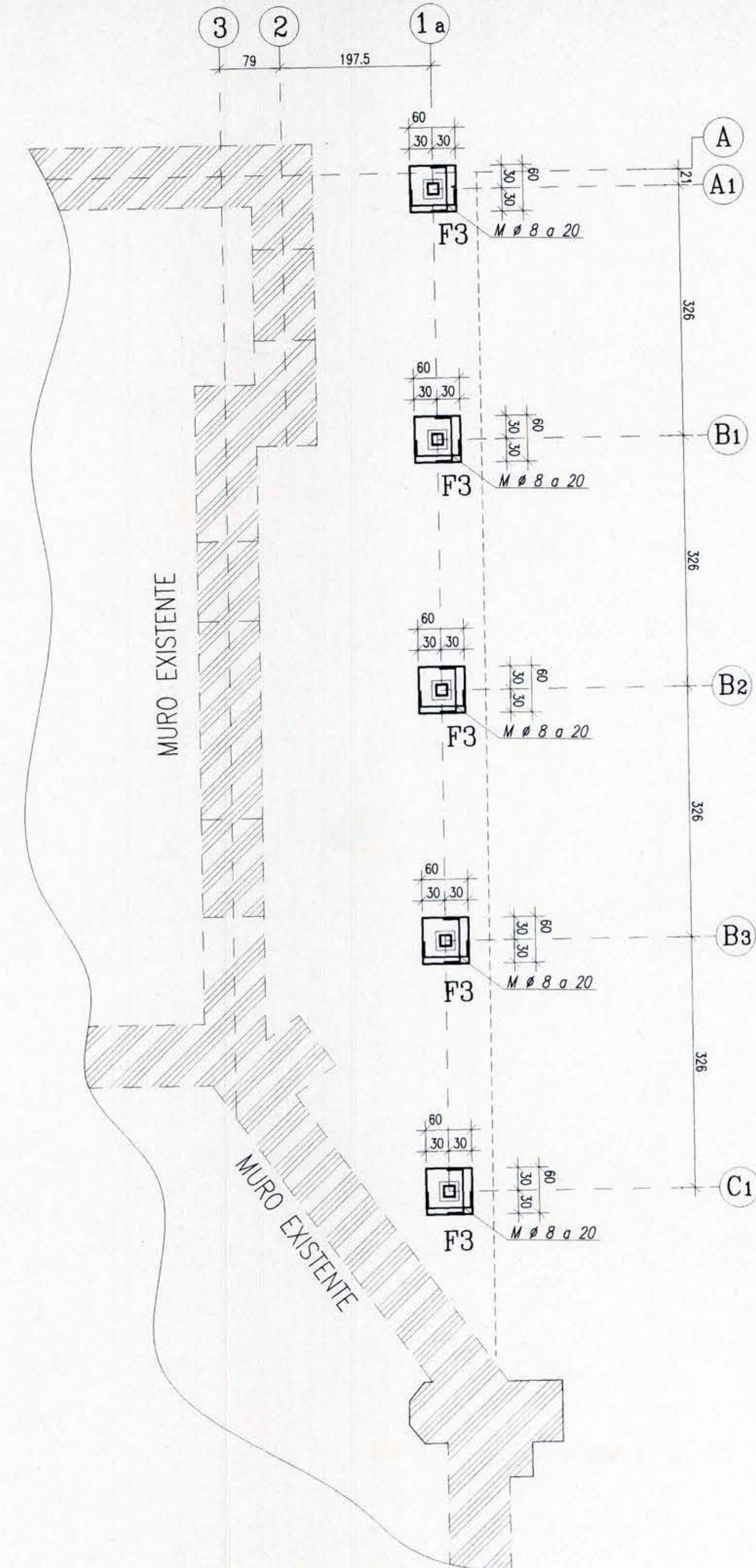
PLANTA DE FUNDACIONES (TECHO PASILLO)
