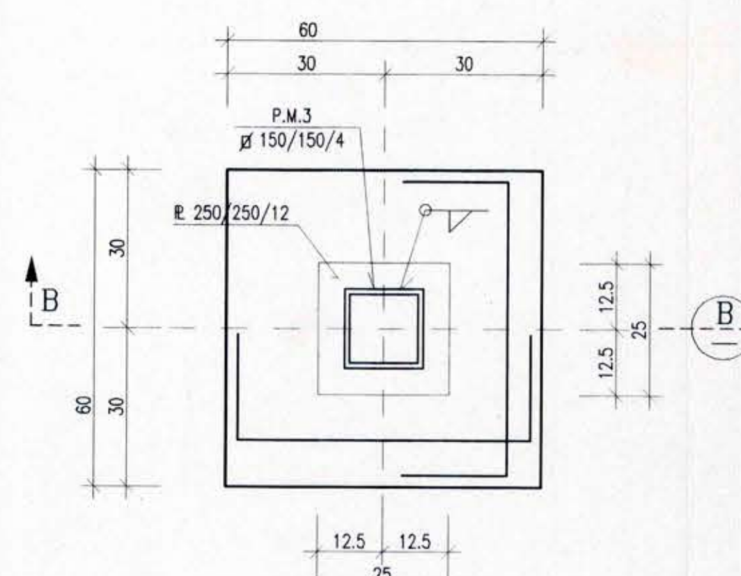
SECCION FUNDACION F3
