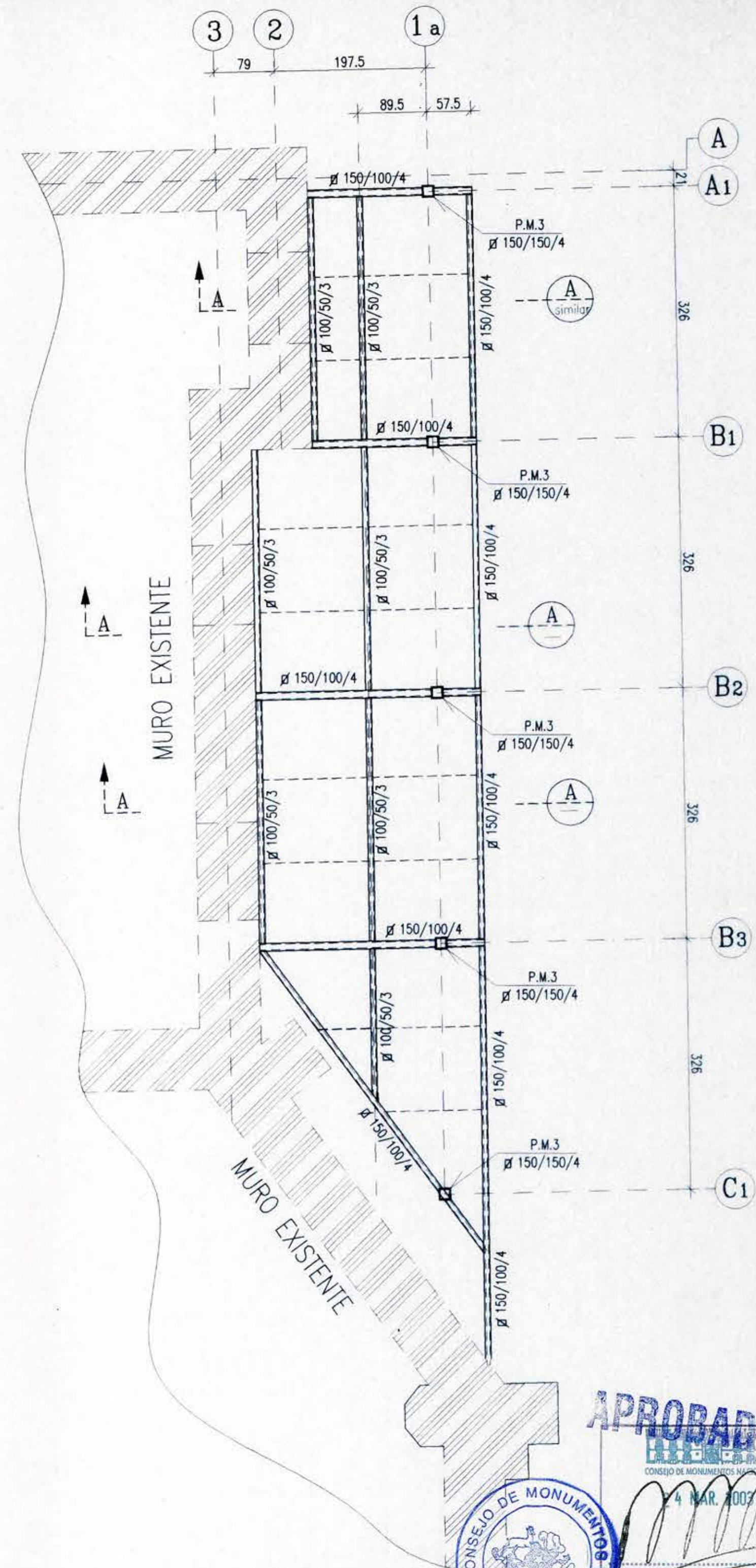
PLANTA DE ESTRUCTURA (TECHO PASILLO)
