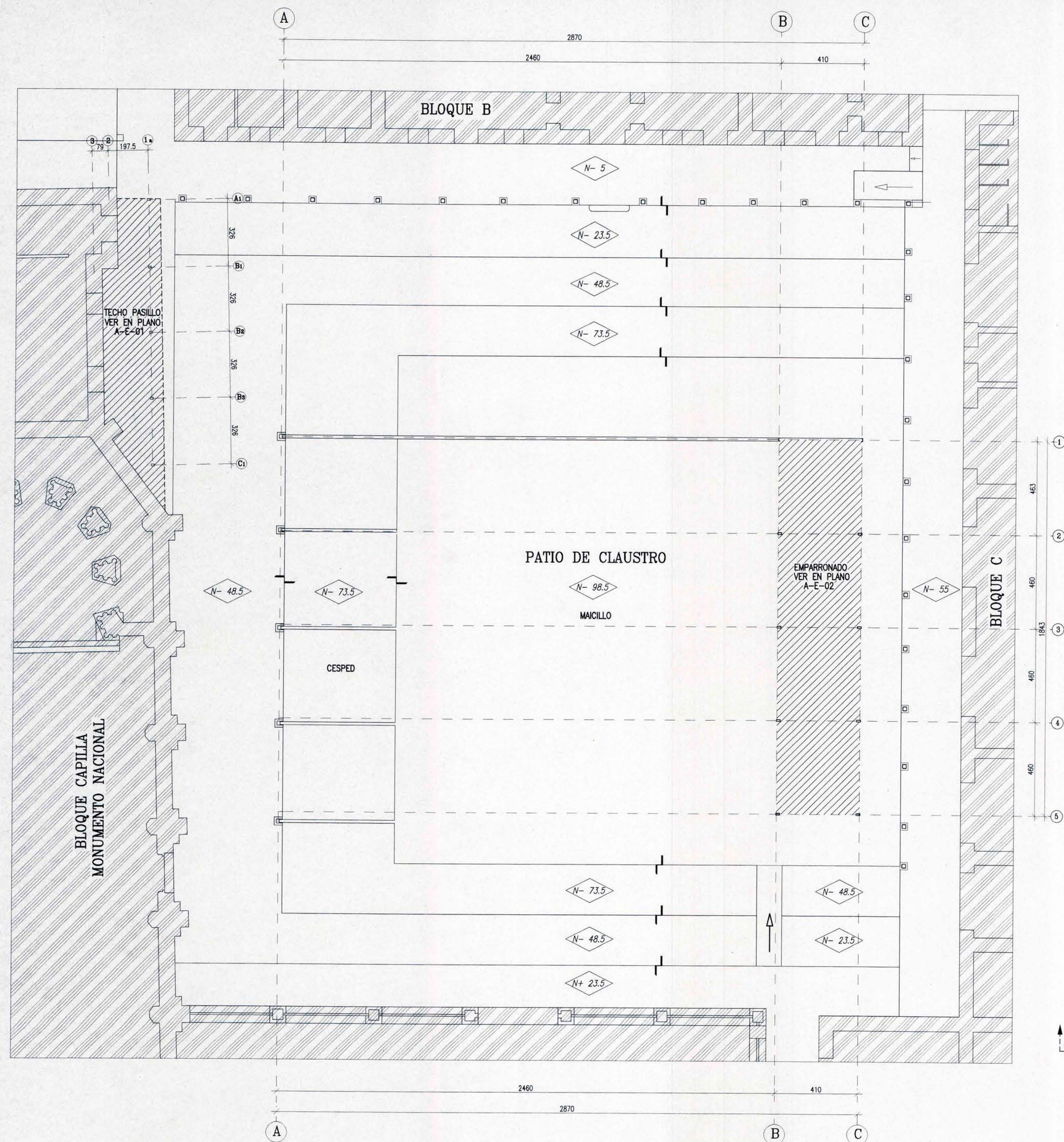
PLANTA DE FUNDACIONES (BLOQUE PATIO DE CLAUSTRO)
