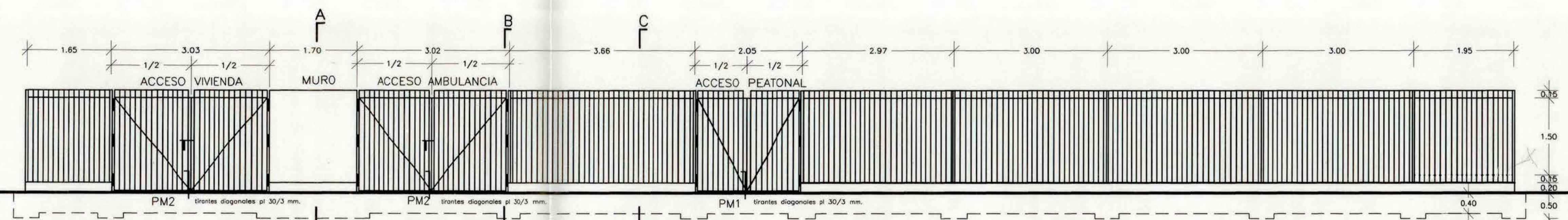
ELEVACION CIERRO ESCALA 1 : 50
