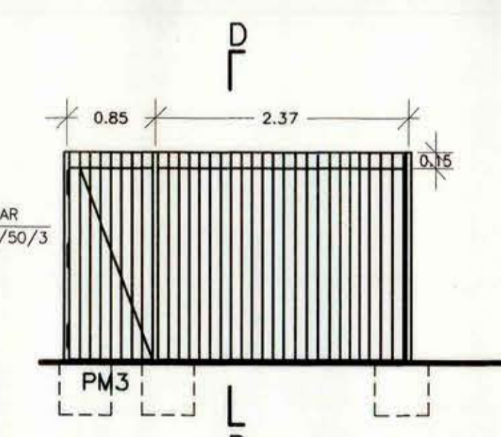
ELEVACION REJA 2 ESCALA 1 : 50
