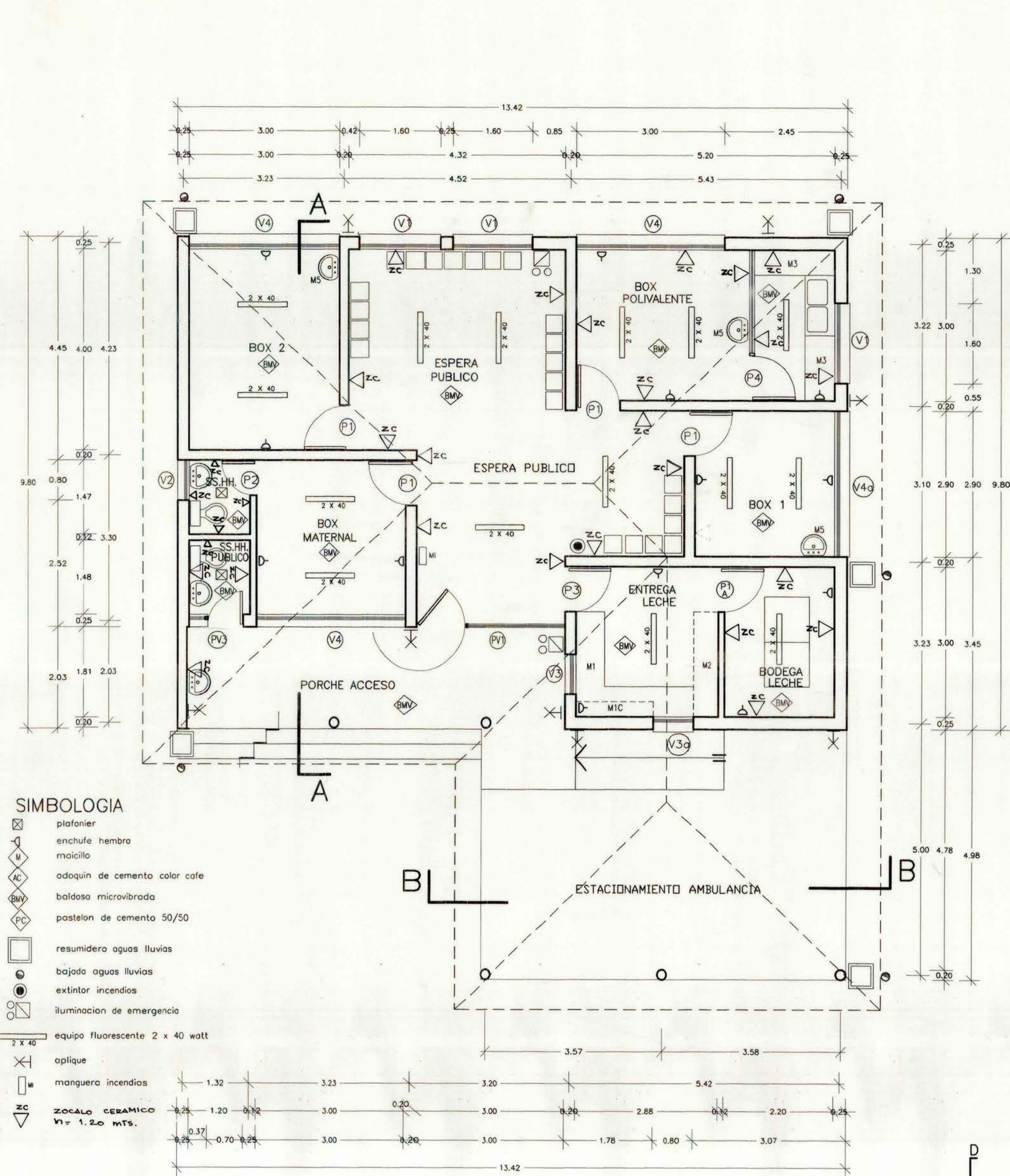
PLANTA ARQUITECTURA ESCALA 1 : 50
