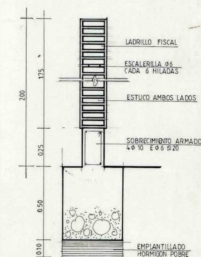
DET. MURO PATIO SERVICIO
