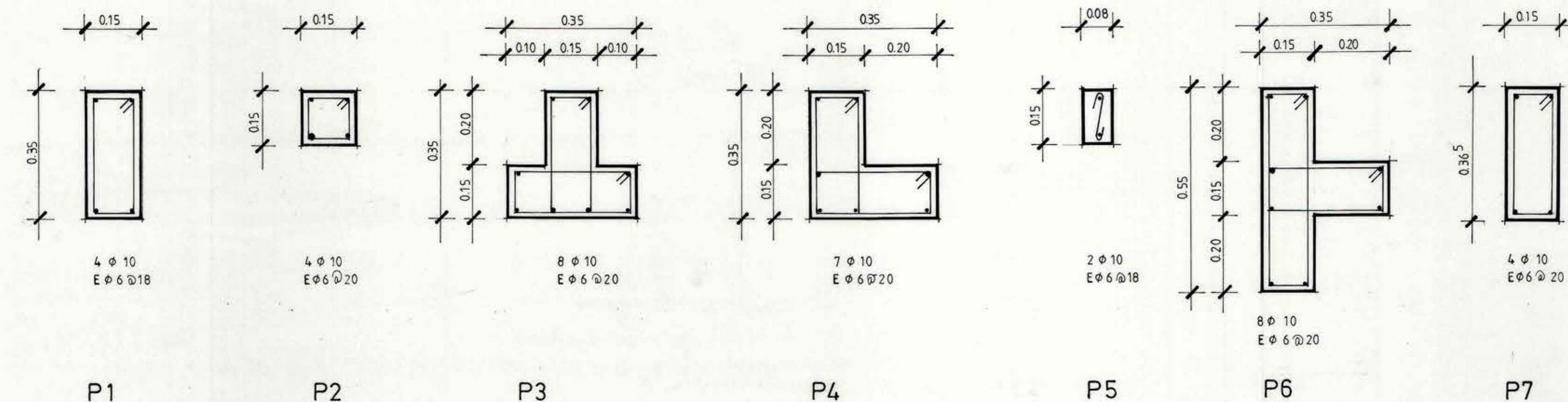
DETALLES DE PILARES ESCALA 1:10
