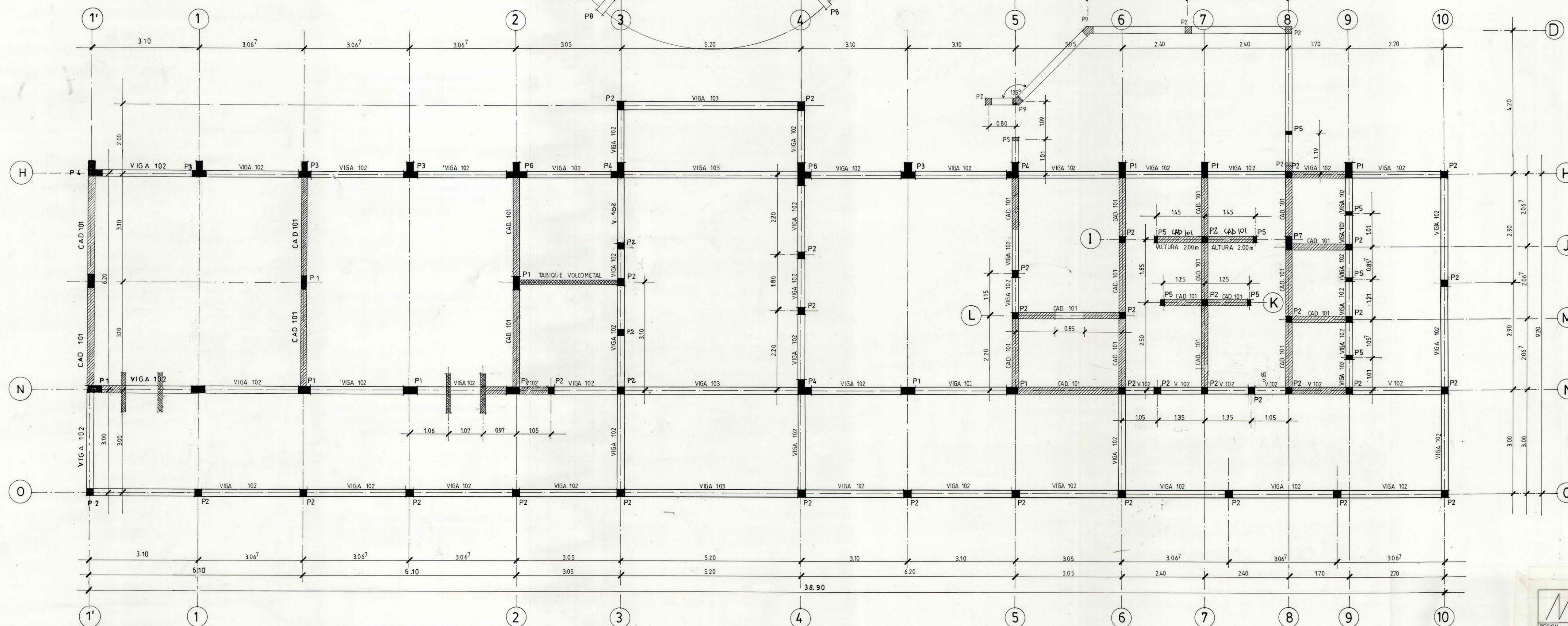
PLANTA DE ESTRUCTURAS ESCALA 1:50
