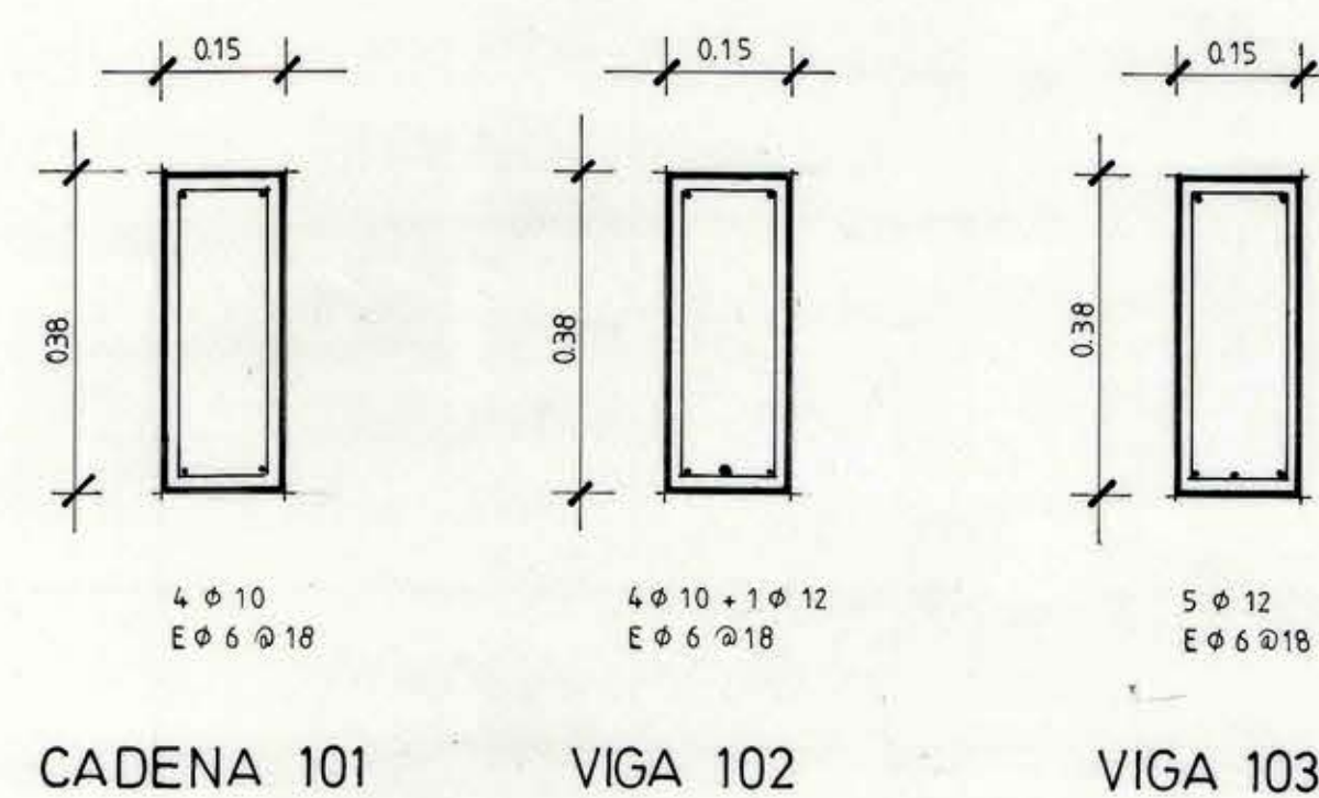
DETALLES DE VIGAS Y CADENA ESCALA 1:10
