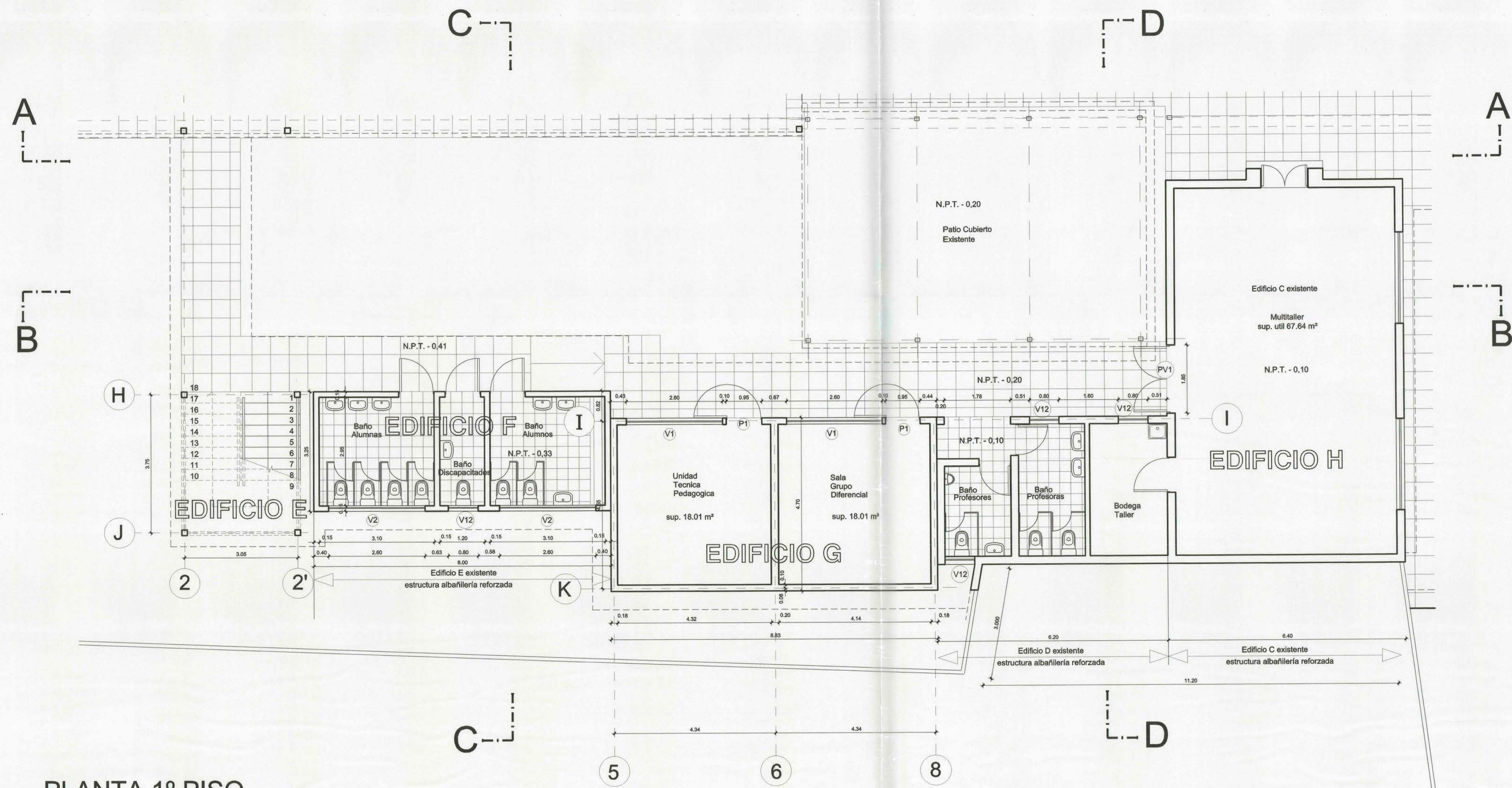
PLANTA 1º PISO Escala 1 : 50
