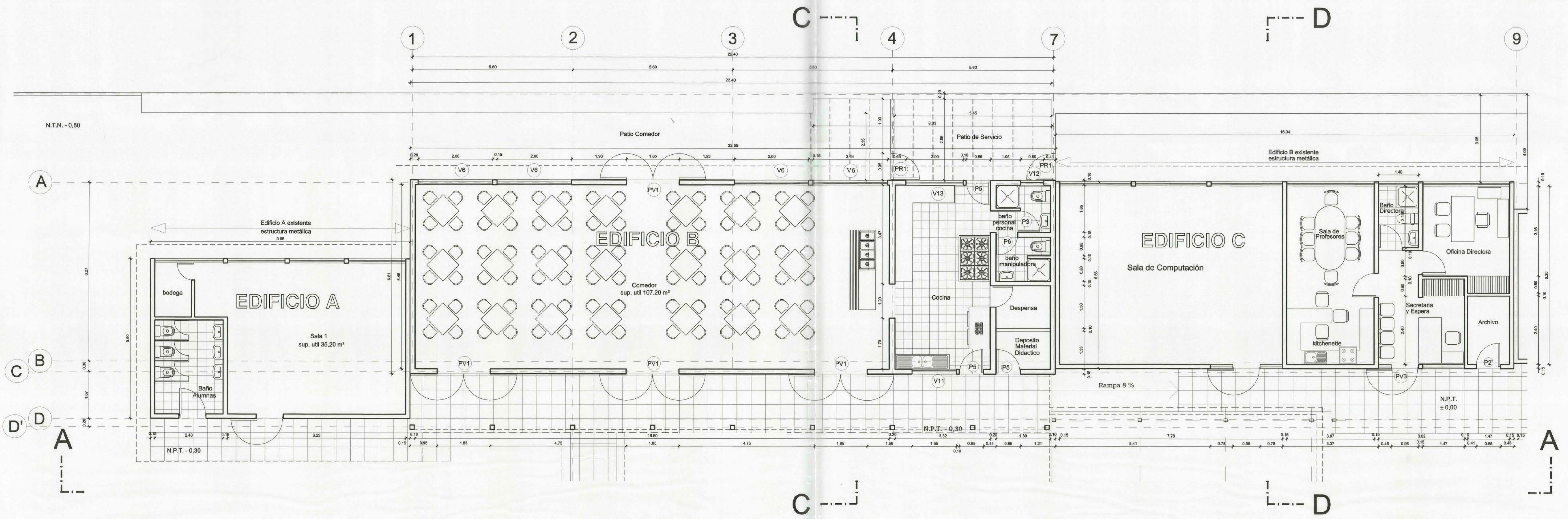
PLANTA 1º PISO Escala 1 : 50
