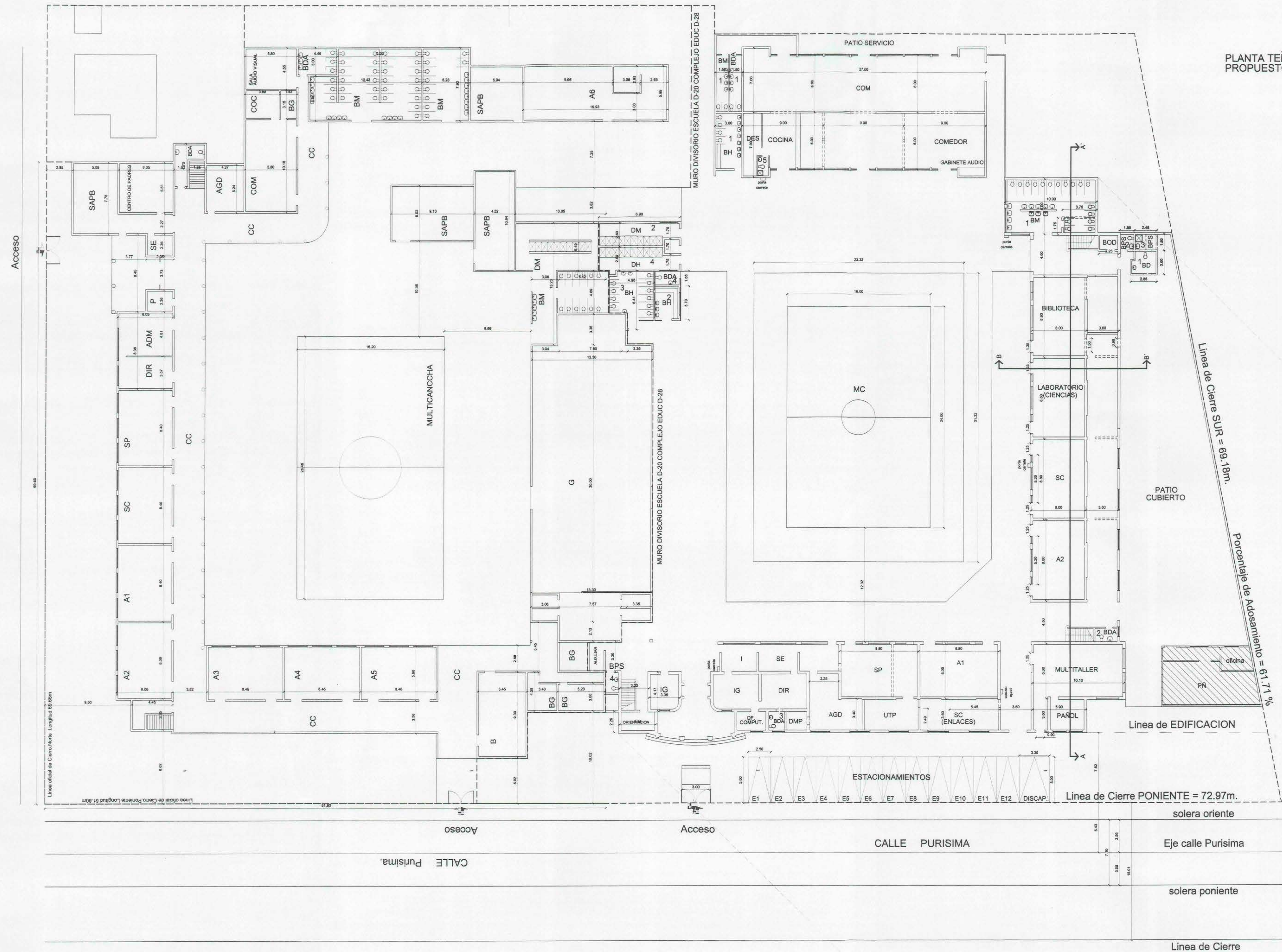
PLANTA EMPLAZAMIENTO SITUACION PROPUESTA ESCALA 1:200
