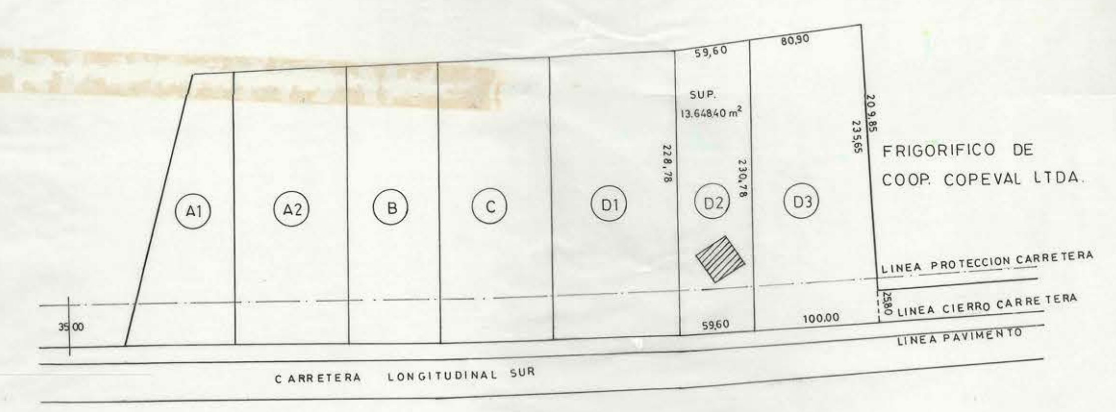
PLANO DE UBICACION ESC.: 1:3000.
