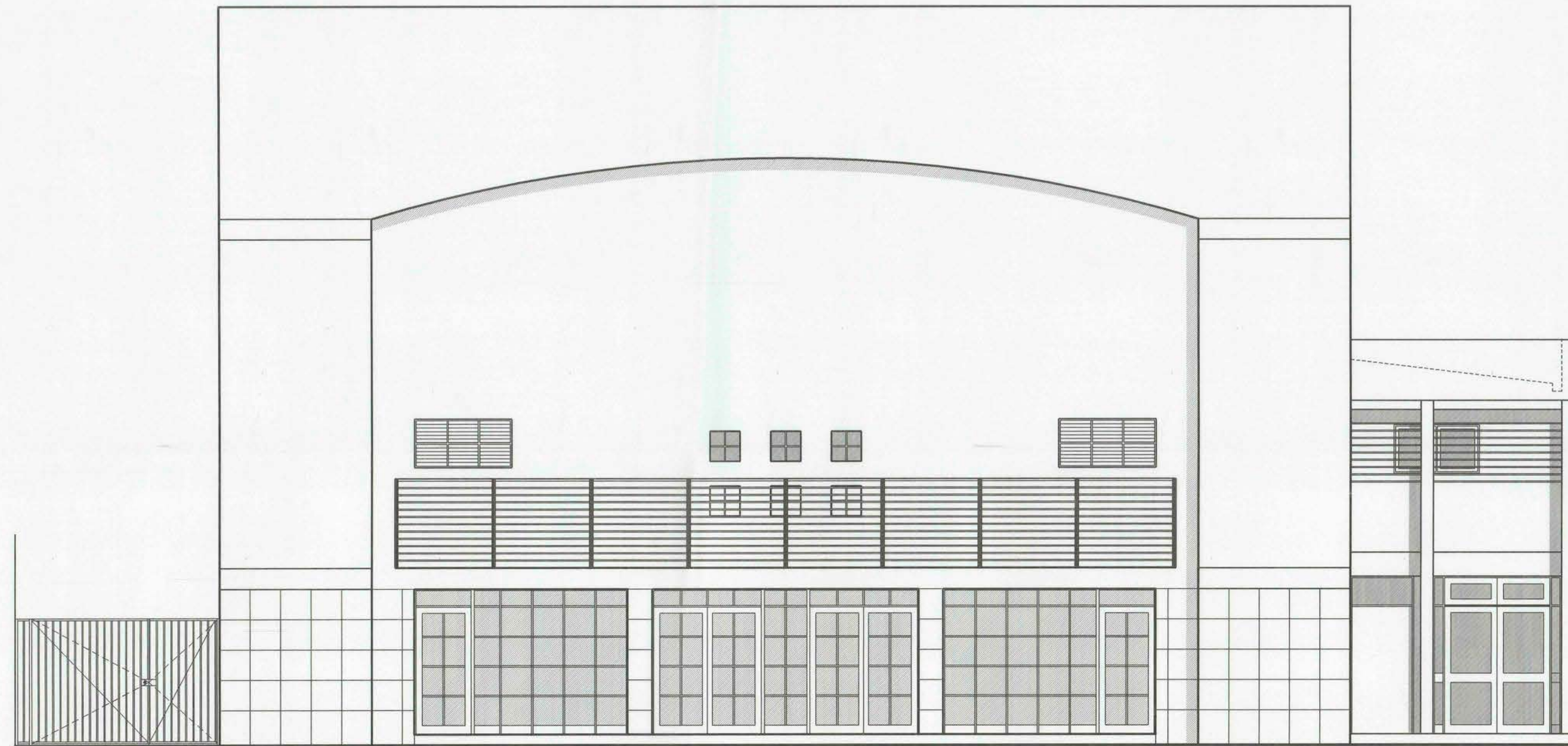
ELEVACION PRINCIPAL ESCALA 1:50
