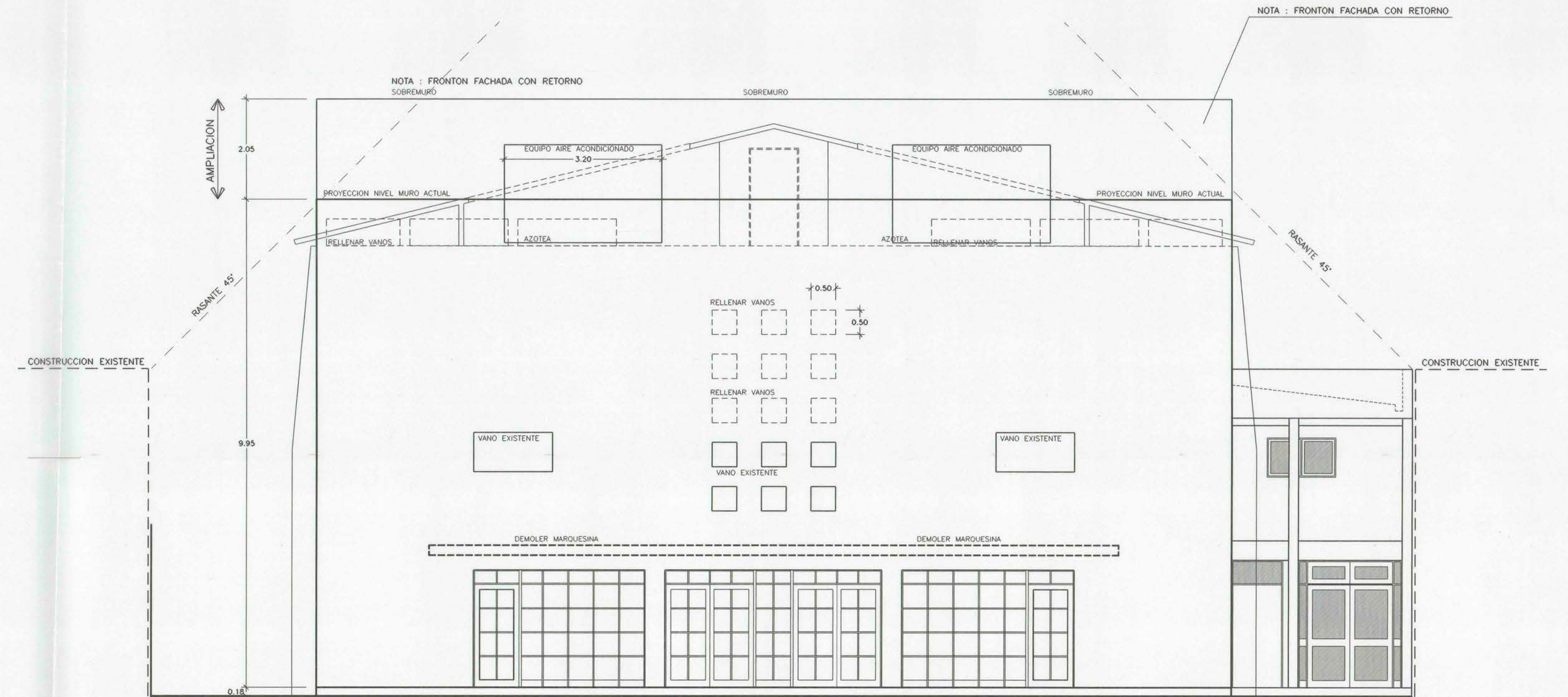
ELEVACION PRINCIPAL A MODIFICAR ESCALA 1:50
