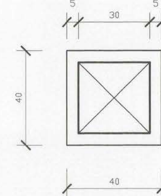
DETALLE PILAR ESCALA 1:10
