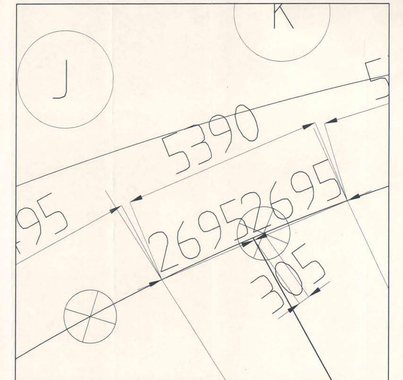
DETALLE APOYO CUPULA ENTRE EJES J/K NOR-ORI ESC:1/50
