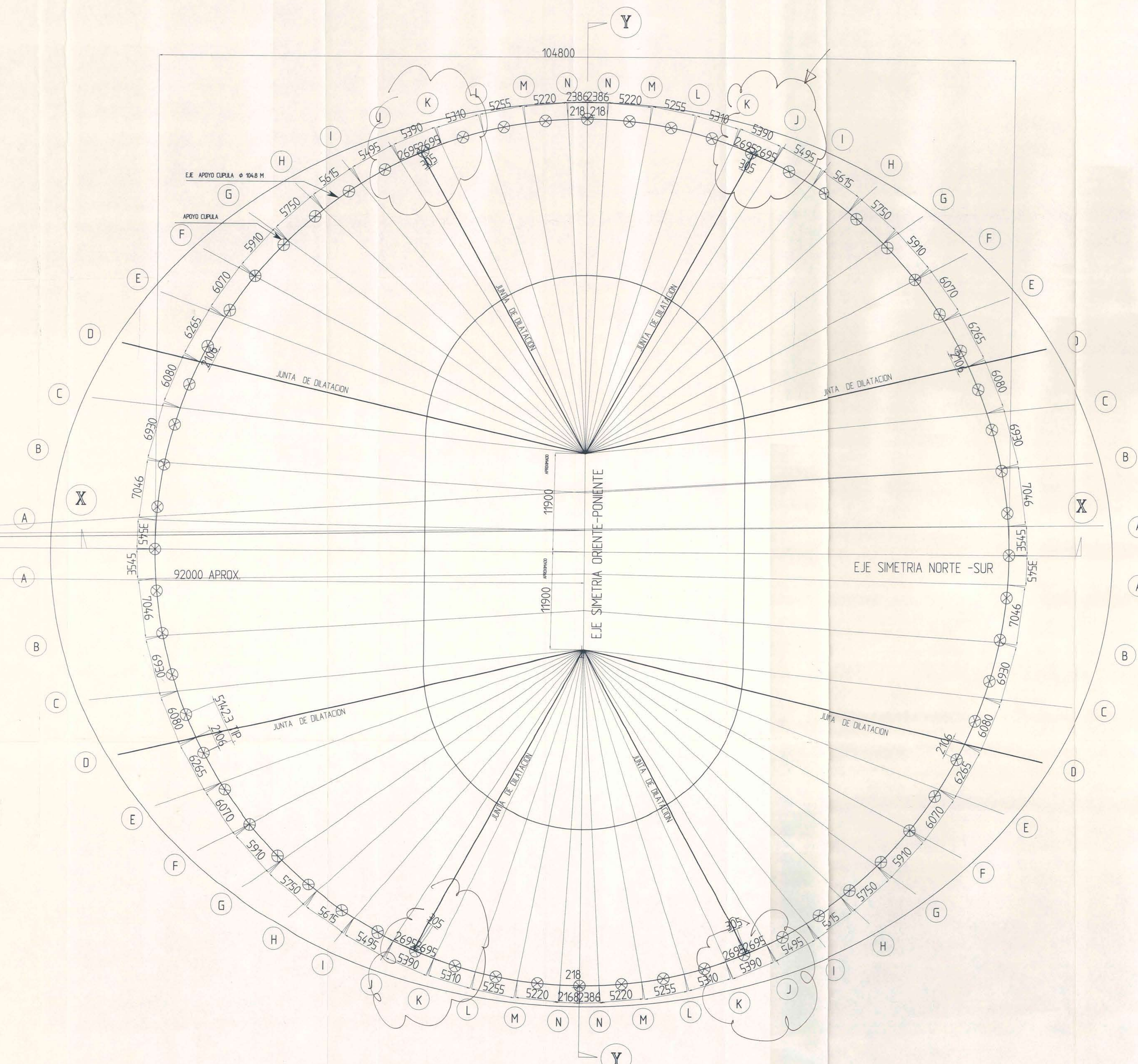
PLANTA EJES + ESTRUCTURA DE APOYO CUPULA ESCALA 1:200
