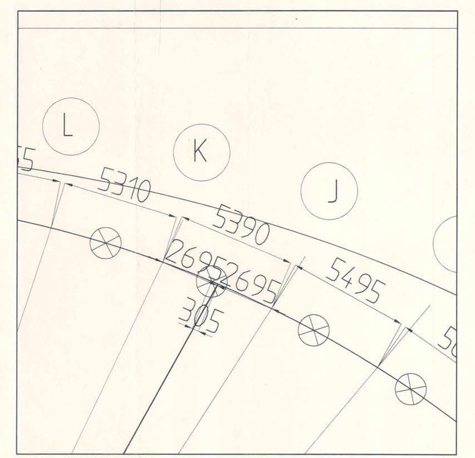
DETALLE APOYO CUPULA ENTRE EJES J/K SUR-ORI ESC:1/100
